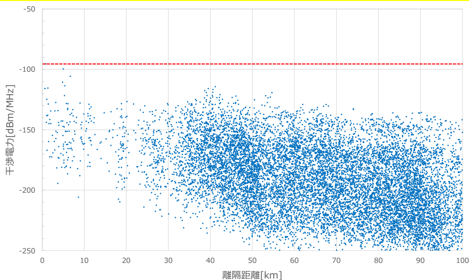
図5. 7. 2. 1-2 基地局が茨城県つくば市の地球局へ及ぼす シングルエントリ（1局）の干渉電力（同一周波数） （赤線：地球局の短時間干渉基準）
