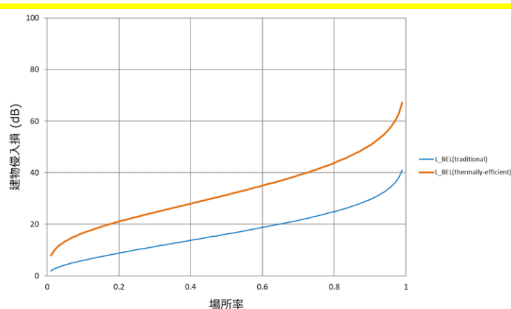
図 4. 6. 2. 1-5 勧告 ITU-R P. 2109 に基づく 4.5GHz 帯の建物侵入損
