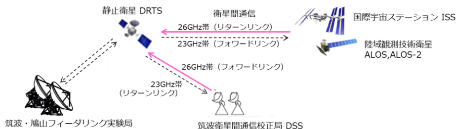
図5. 1. 1. 2-1 衛星間通信の概要
