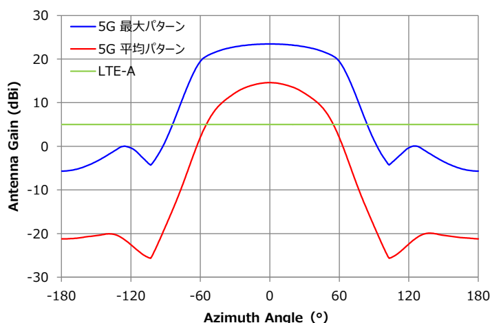
(a) 水平面パターン
