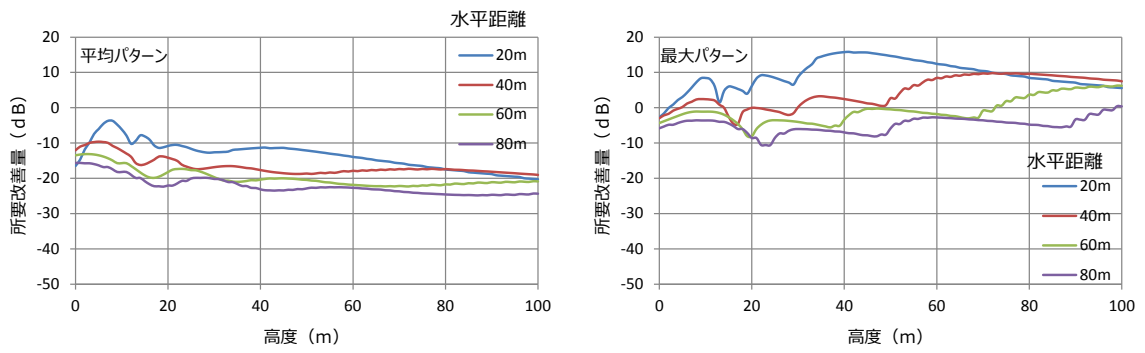
(b) 帯域外干渉 (周波数離調 60MHz)
