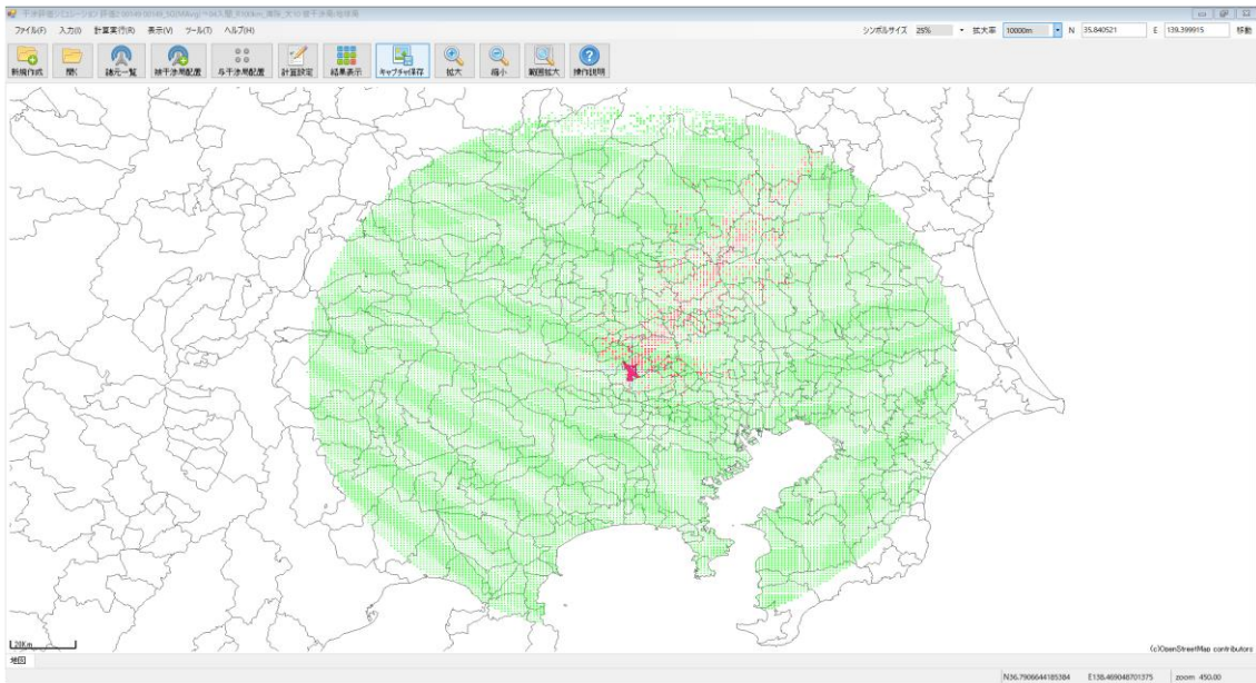
(a) 公共業務用無線局の周囲 100km の範囲に 1 局/km 2 の密度で基地局を配置した場合
