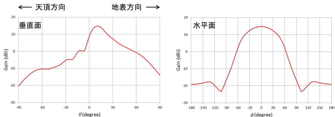
(a) マクロセル基地局
