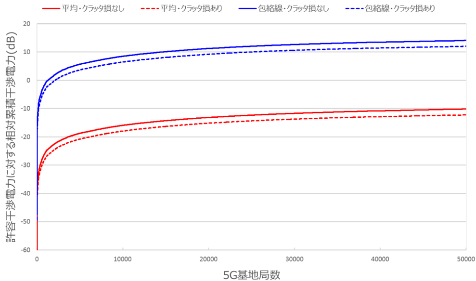
図5. 3. 2. 1-6 静止衛星3に対する検討結果 (同一周波数干渉)
