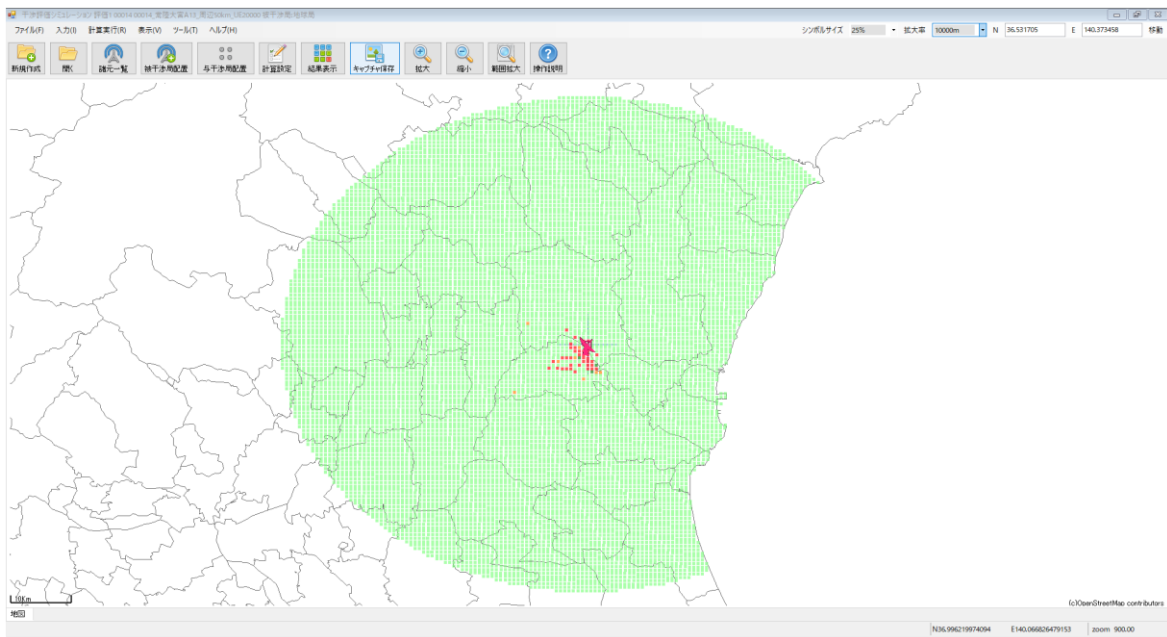
(b) 茨城県常陸大宮市 図4. 3. 2. 1-6 陸上移動局から首都圏の地球局等への干渉影響
