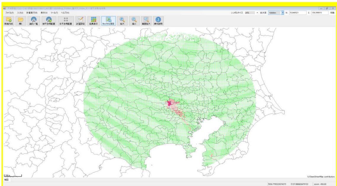
(c) 建物種別 Thermally-efficient、場所率 50%、基地局の空中線高 50m (高層階) 図 4. 6. 2. 1-7 公共業務用無線局から屋内基地局への干渉検討結果の一例 (公共業務用無線局の周囲 100km の範囲に 1局/km 2 の密度で基地局を配置、 関東地方①、方位角②)
