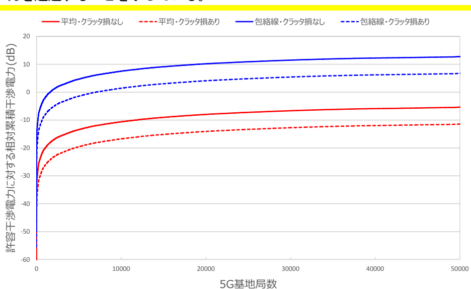
(a) 同一周波数干渉
