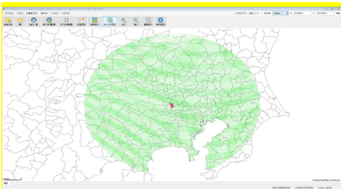
(c) 建物種別 Thermally-efficient、場所率 50%、基地局の空中線高 50m (高層階) 図 4. 6. 2. 1-9 屋内基地局から公共業務用無線局への干渉検討結果の一例 (公共業務用無線局の周囲 100km の範囲に 1局/km 2 の密度で基地局を配置、 関東地方①、方位角②)
