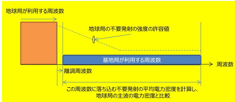
図5. 4. 2. 2-5 隣接周波数干渉における同一周波数干渉に比較した干渉電力レベルの低減量の算出方法
