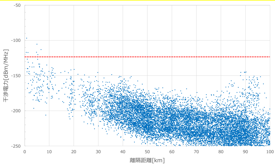
図5. 7. 2. 1-1 基地局が茨城県つくば市の地球局へ及ぼす シングルエントリ（1局）の干渉電力（同一周波数）
