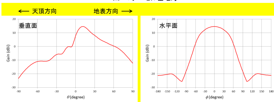
(b) スモールセル基地局
