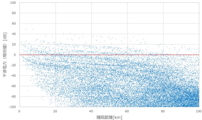
(a) 公共業務用無線局の周囲100kmの範囲に1局/km 2 の密度で基地局を配置した場合
