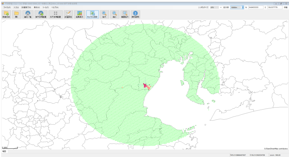
(c) 三重県鈴鹿市 図 4. 3. 2. 1-16 陸上移動局から中京・近畿圏の地球局等への干渉影響
