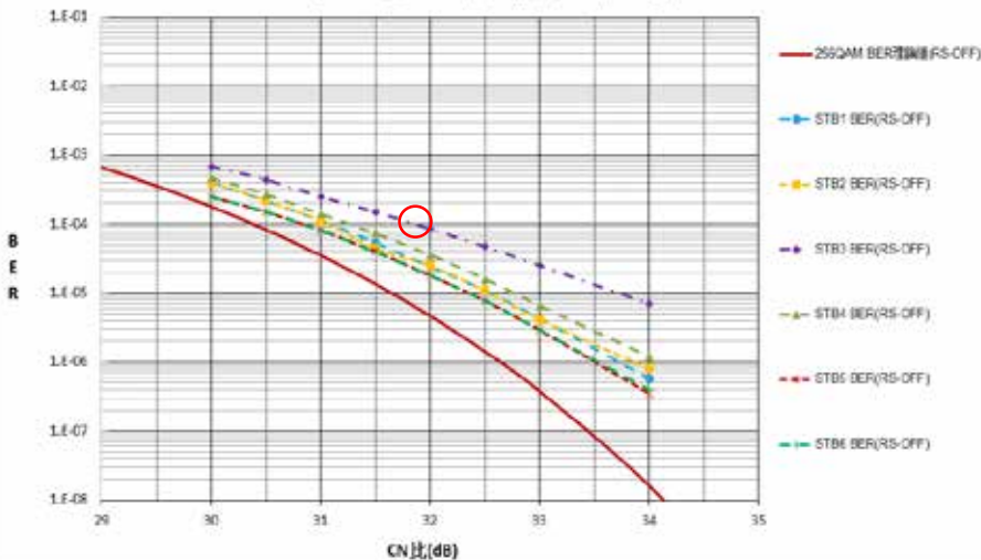
256QAM CN比 vs BER (U61, 入力55dB \mu Vの時)
