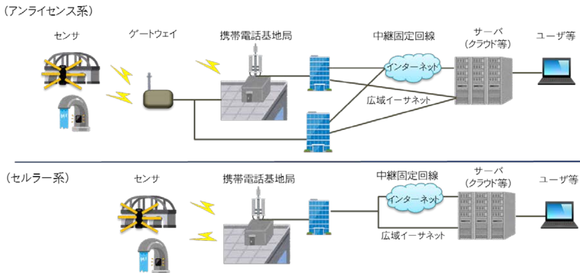
図 3.2 LPWA サービスのネットワーク構成イメージ
