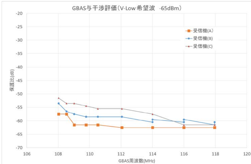
図参 31 保護比 (中間 3seg/V-Low 希望波-65dBm)
