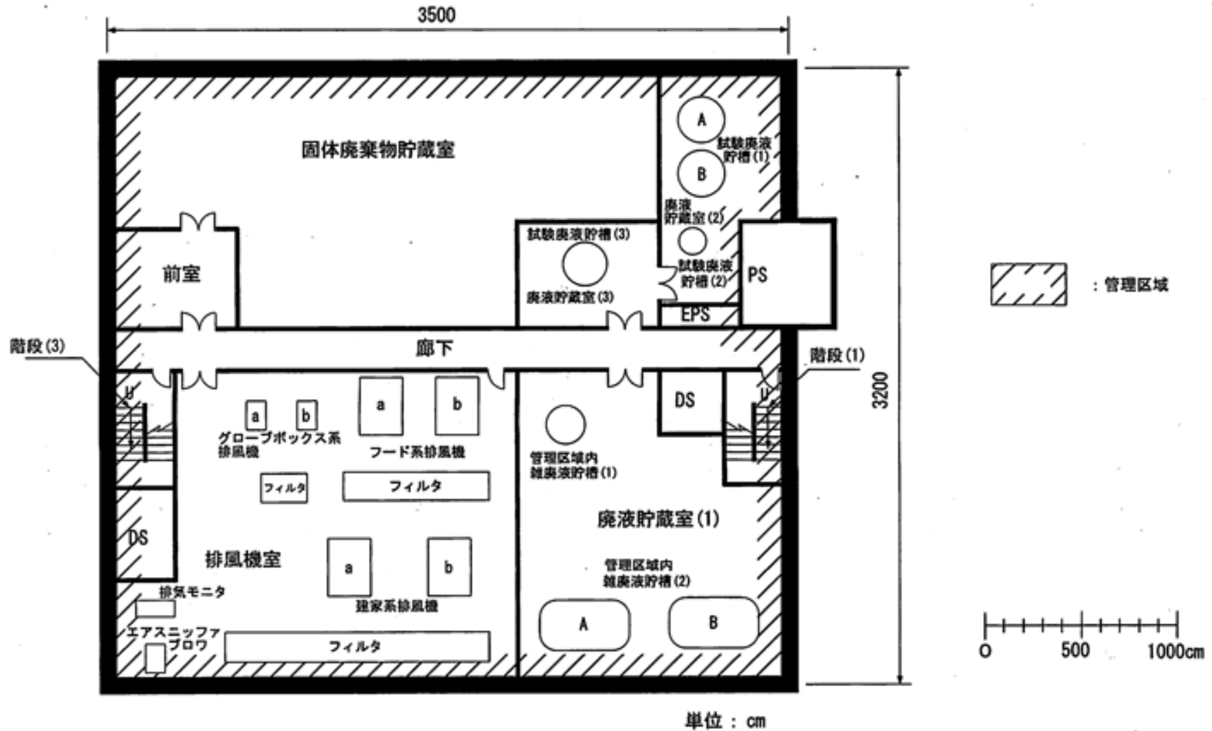
地層処分放射化学研究施設 主要機器配置図 (地下1階)
