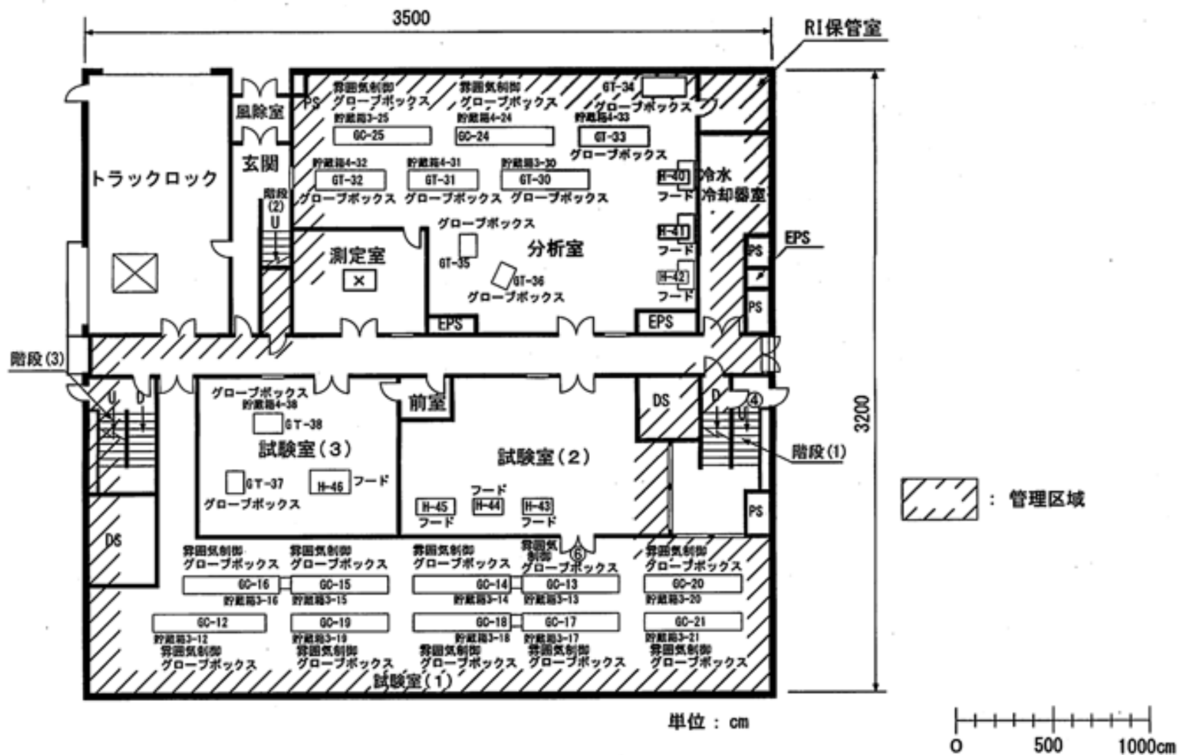
地層処分放射化学研究施設 主要機器配置図 (1階)
