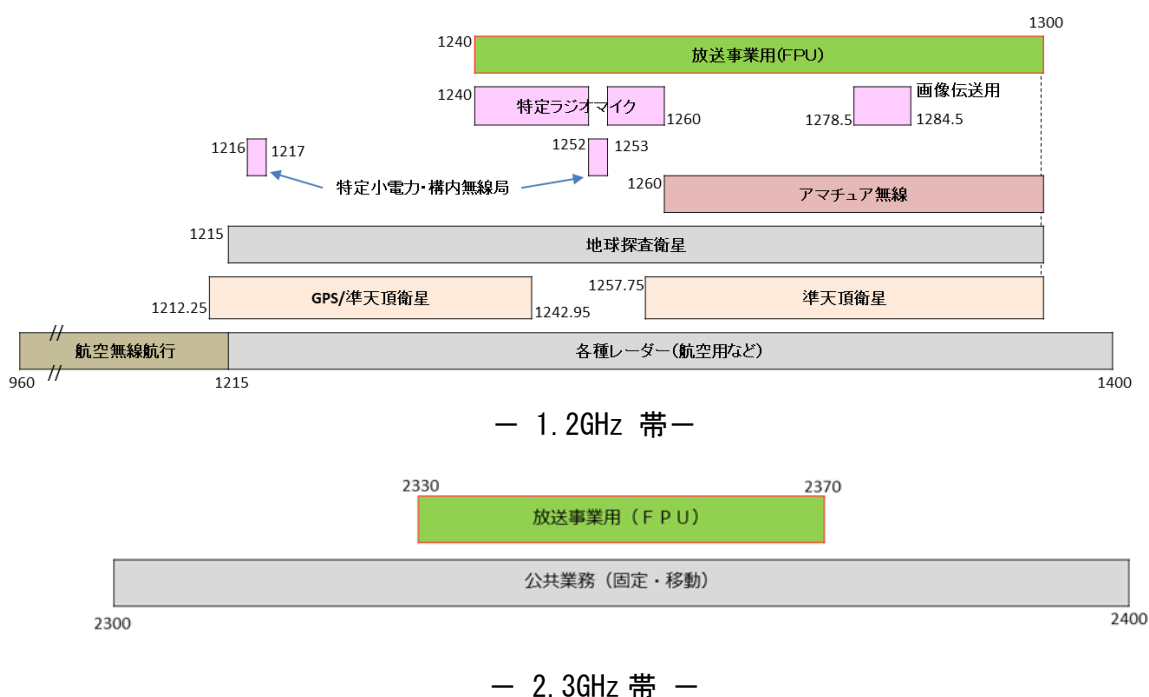
図7 1240～1300MHz、2330～2370MHz 周波数帯の割当状況
