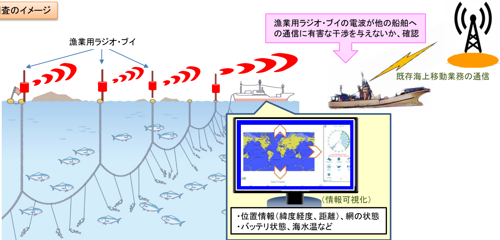
26MHz帯漁業用ラジオ・ブイから送信された各種情報を船舶で受信
