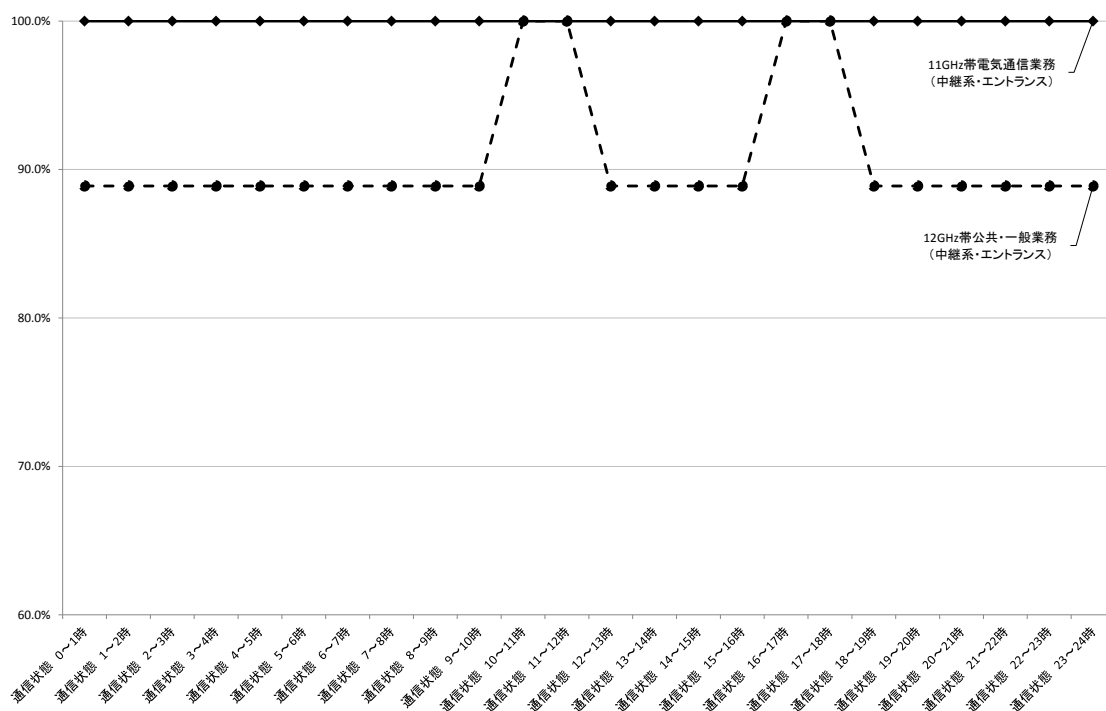
図表一陸一 6－7 「通信状態」のシステム別比較 (11GHz 帯電気通信業務（中継系・エントランス）、12GHz 帯公共・一般業務（中継系・エントランス）)
