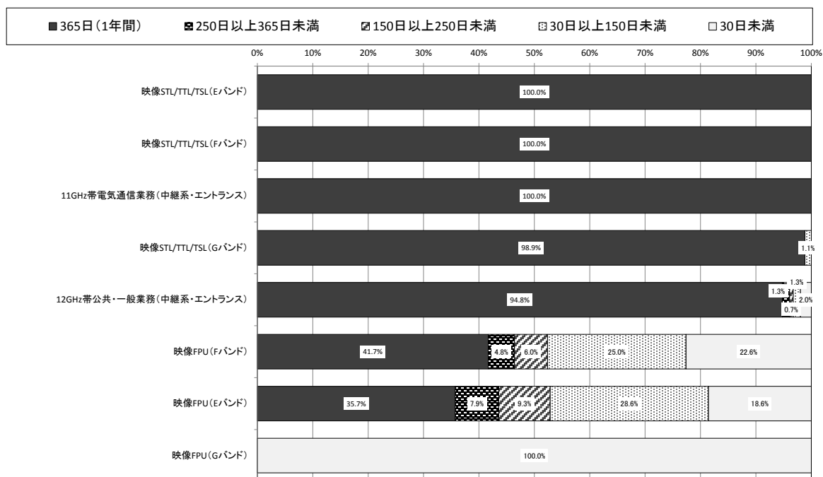
図表－全－6－8 「年間の運用状態」のシステム別比較
