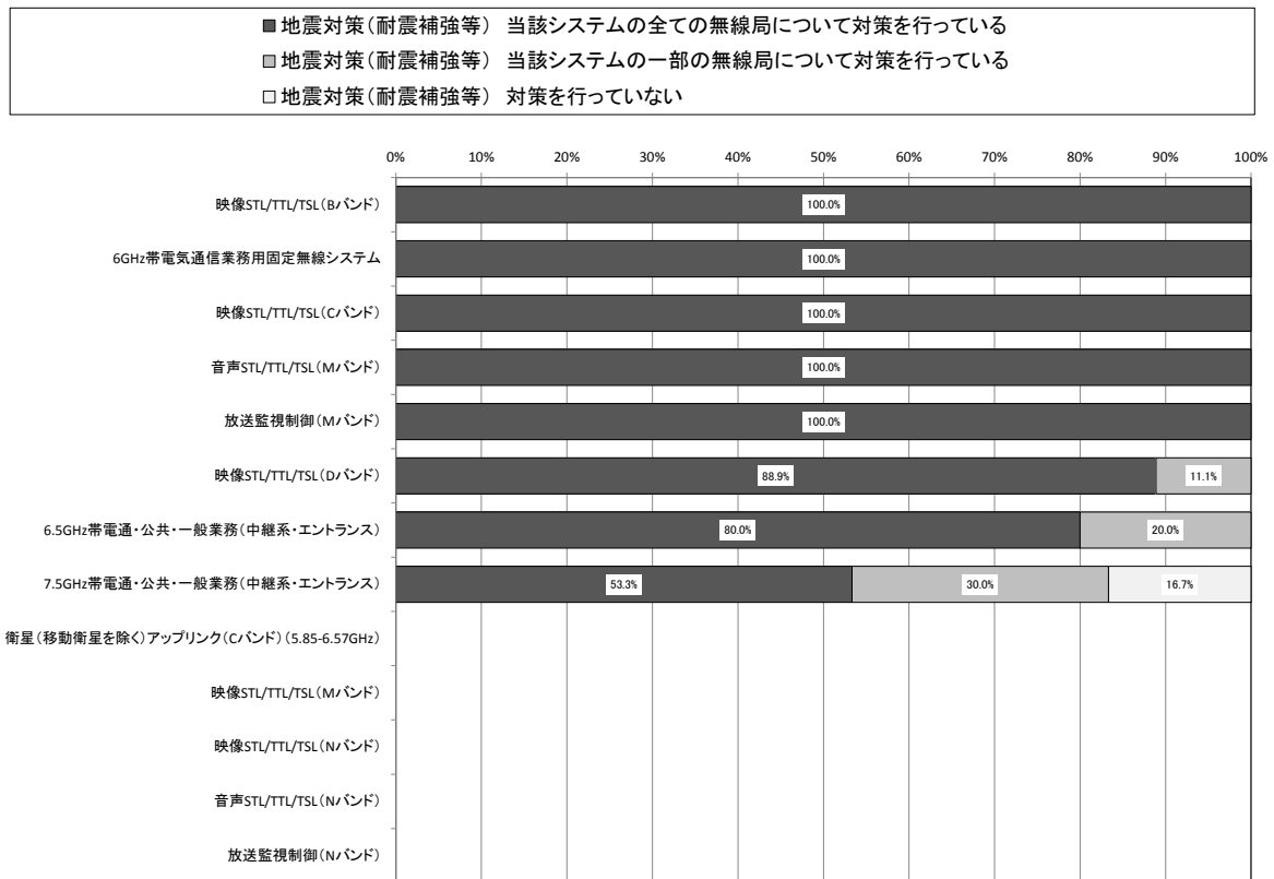
図表一信－４－１５ 「地震対策（耐震補強等）」のシステム別比較
