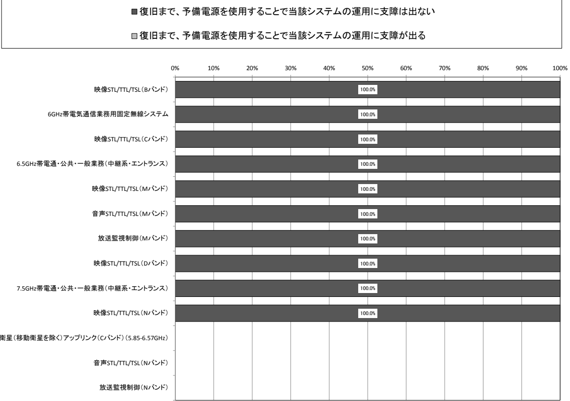
図表一四－４－２４ 「予備電源によるシステムの運用可否」のシステム別比較
