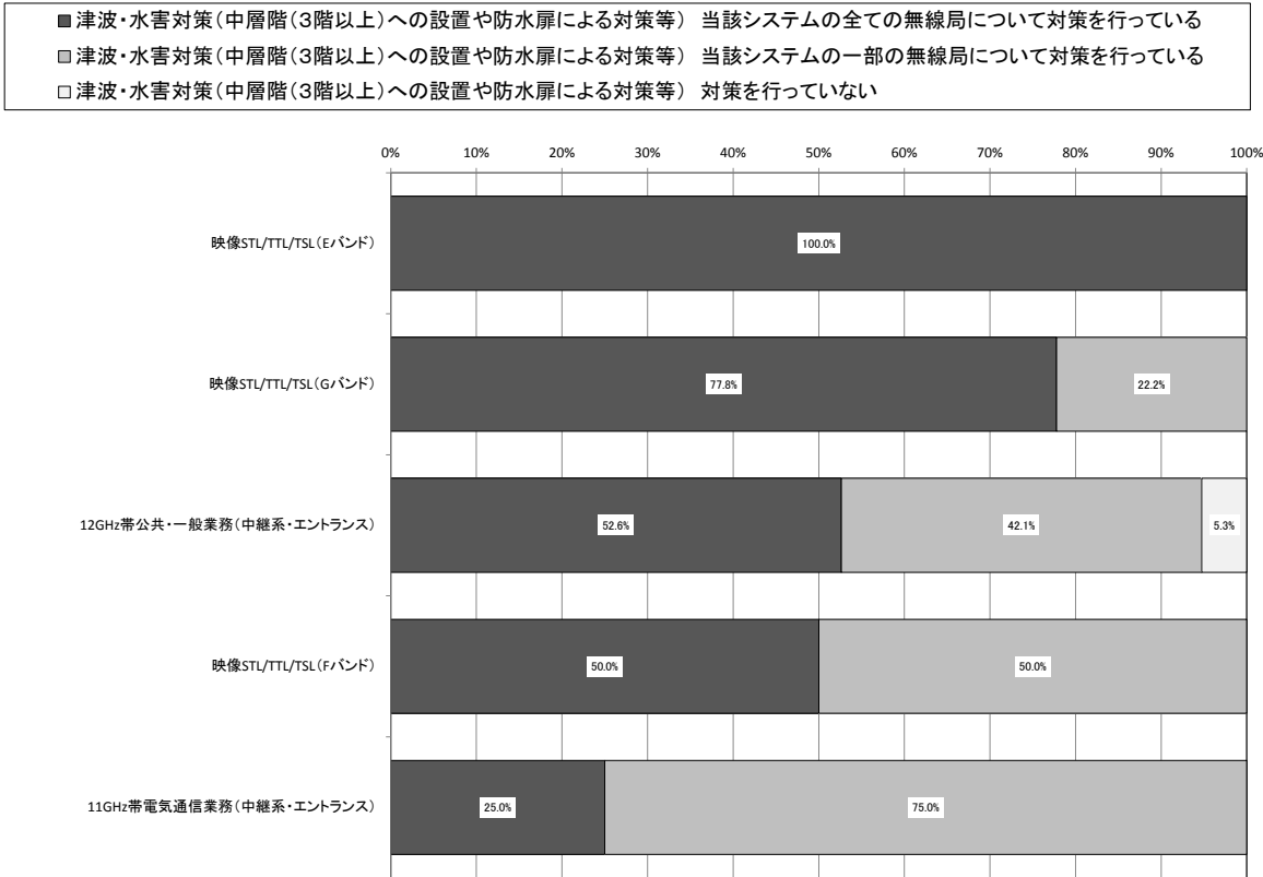
図表一近一 6－1 6 「津波・水害対策（中層階（3 階以上）への設置や防水扉による対策等）」のシステム別比較
