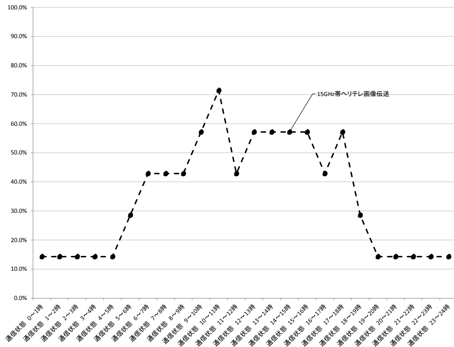
図表－海－７－７ 「通信状態」のシステム別比較（15GHz 帯ヘリテレ画像伝送）
