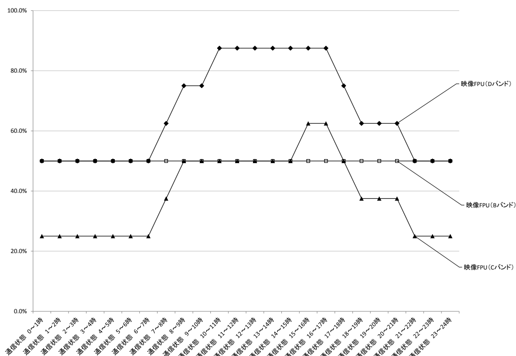
図表一信－４－７ 「通信状態」のシステム別比較（映像 FPU（B バンド）、映像 FPU（C バンド）、映像 FPU（D バンド））
