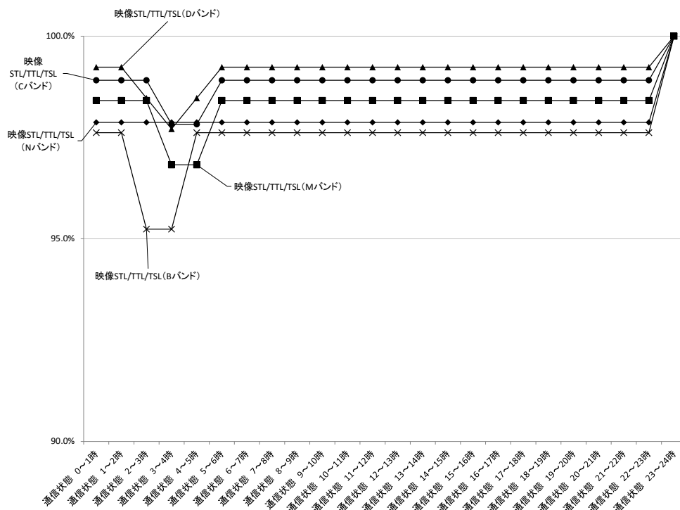
図表一全一４－８ 「通信状態」のシステム別比較（映像 STL/TTL/TSL（Bバンド）、映像 STL/TTL/TSL（Cバンド）、映像 STL/TTL/TSL（Mバンド）、映像 STL/TTL/TSL（Dバンド）、映像 STL/TTL/TSL（Nバンド））
