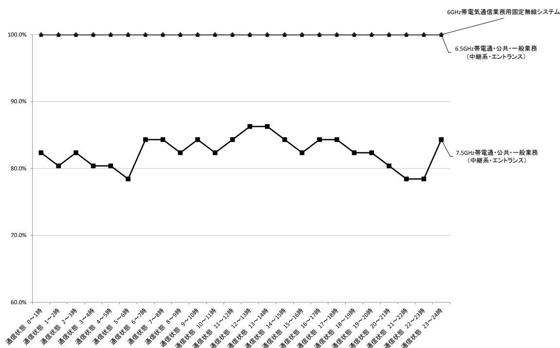
図表一東一4一5「通信状態」のシステム別比較 (6GHz帯電気通信業務用固定無線システム、6.5GHz帯電通・公共・一般業務(中継系・エントランス)、 7.5GHz帯電通・公共・一般業務(中継系・エントランス))
