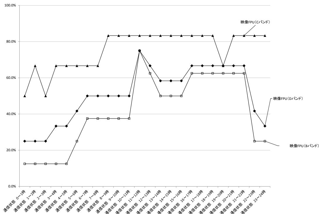
図表一関一４－７ 「通信状態」のシステム別比較（映像 FPU（B バンド）、映像 FPU（C バンド）、映像 FPU（D バンド））
