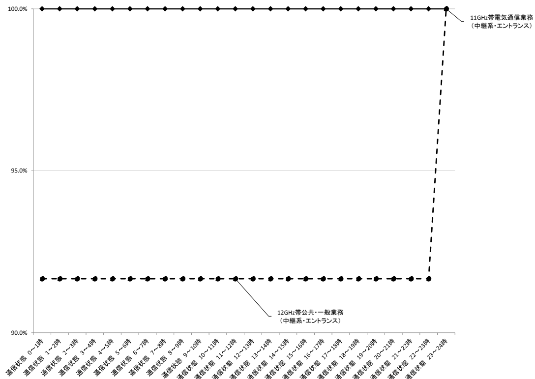
図表一東一六一七「通信状態」のシステム別比較 (11GHz 帯電気通信業務(中継系・エントランス)、12GHz 帯公共・一般業務(中継系・エントランス))
