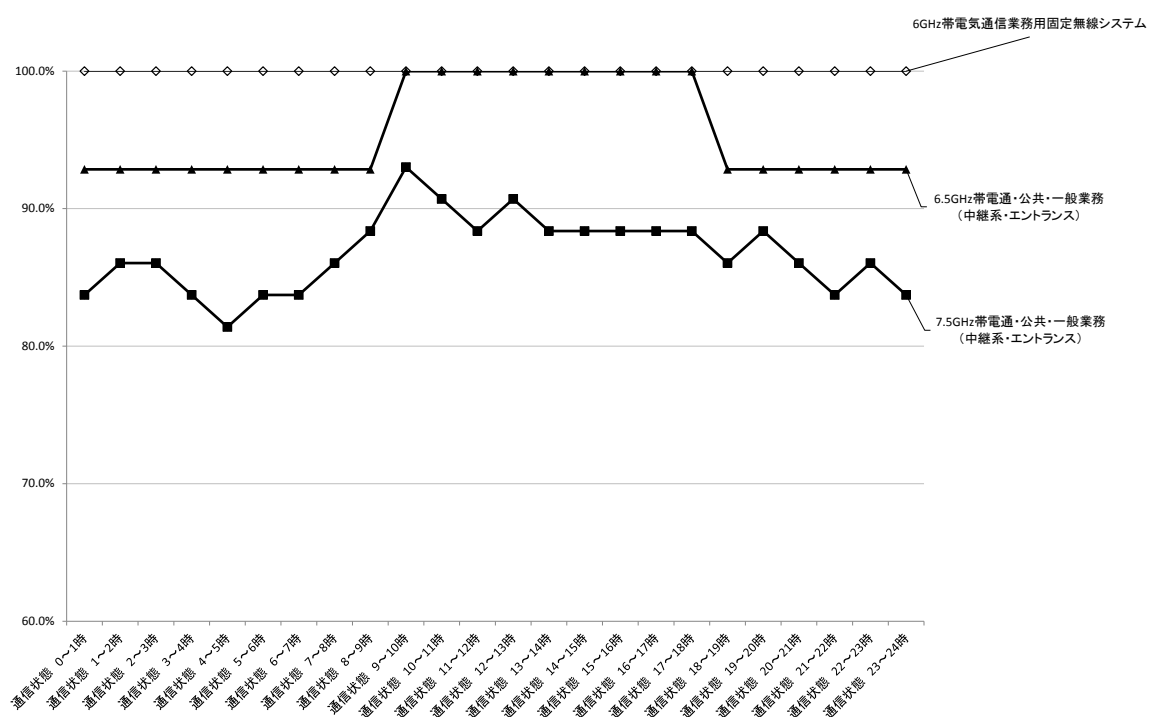
図表－近－４－５ 「通信状態」のシステム別比較 (6GHz 帯電気通信業務用固定無線システム、6.5GHz 帯電通・公共・一般業務(中継系・エントランス)、 7.5GHz 帯電通・公共・一般業務(中継系・エントランス))
