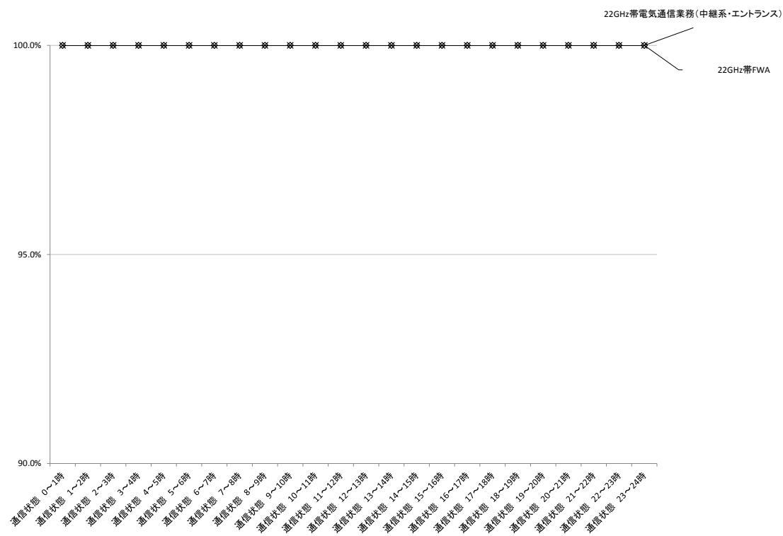
図表一近一８－６ 「通信状態」のシステム別比較（22GHz 帯 FWA、 22GHz 帯電気通信業務（中継系・エントランス））
