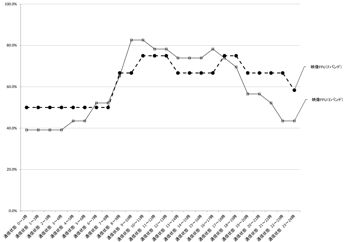
図表一九－６－６ 「通信状態」のシステム別比較（映像 FPU（E バンド）、映像 FPU（F バンド）、映像 FPU（G バンド））
