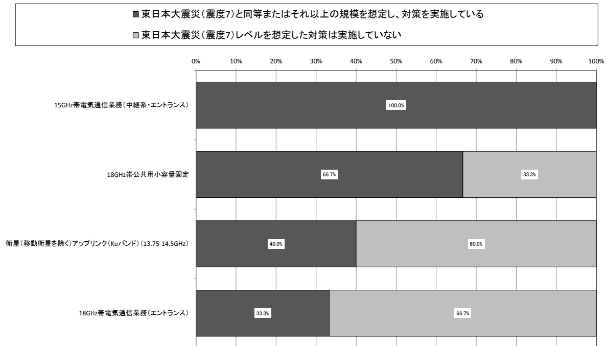
図表－近－７－１３ 「想定している地震の規模」のシステム別比較
