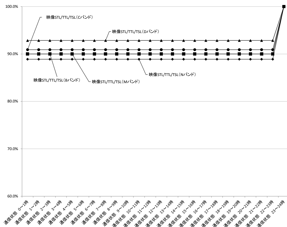
図表－関－４－８ 「通信状態」のシステム別比較（映像 STL/TTL/TSL（B バンド）、映像 STL/TTL/TSL（C バンド）、映像 STL/TTL/TSL（M バンド）、映像 STL/TTL/TSL（D バンド）、映像 STL/TTL/TSL（N バンド））
