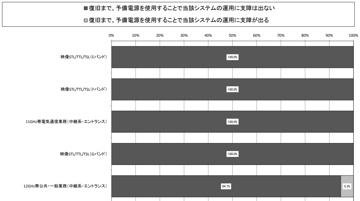
図表－近－６－２２ 「予備電源によるシステムの運用可否」のシステム別比較
