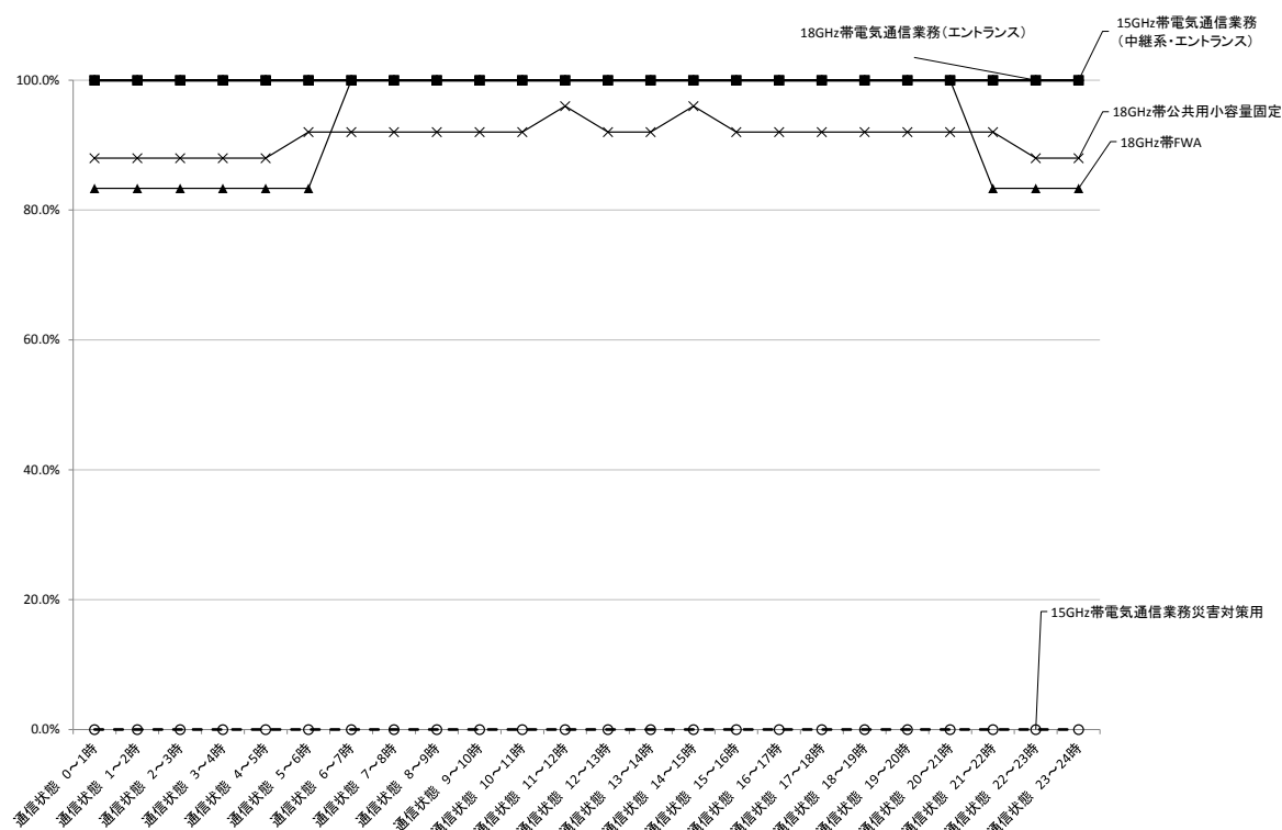
図表一中一七ー六「通信状態」のシステム別比較（15GHz 帯電気通信業務（中継系・エントランス）、15GHz 帯電気通信業務災害対策用、15GHz 帯電気通信業務テレビ伝送用、18GHz 帯公共用小容量固定、18GHz 帯 FWA、18GHz 帯電気通信業務（エントランス））
