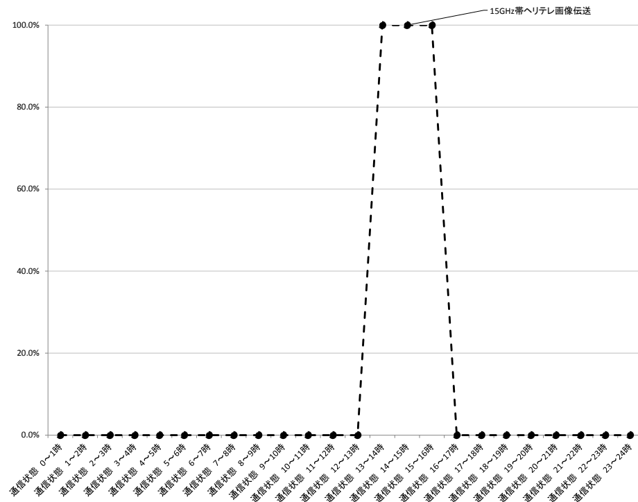
図表一沖一七ー七 「通信状態」のシステム別比較（15GHz 帯ヘリテレ画像伝送）
