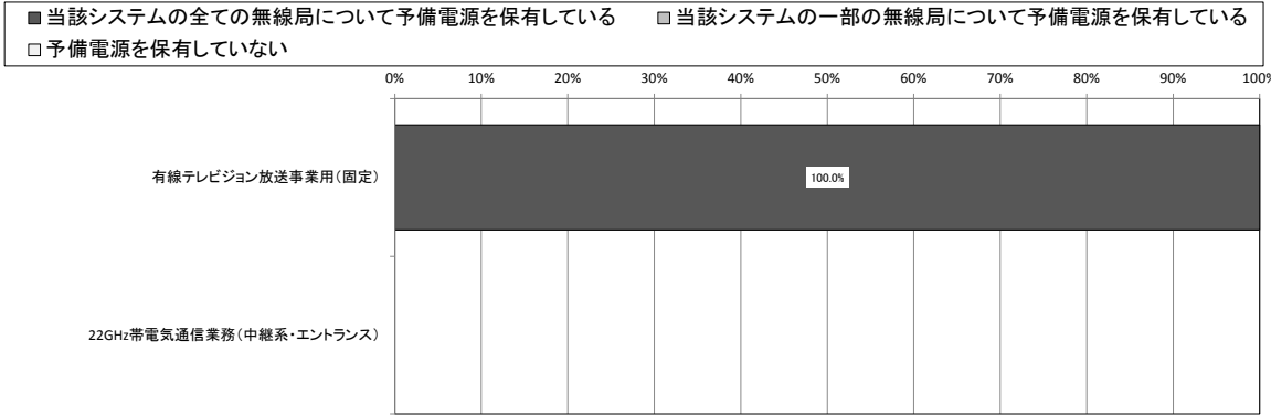
図表一中－８－１８ 「予備電源の有無」のシステム別比較
