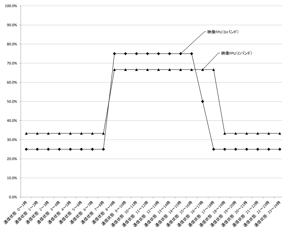
図表－沖－４－７ 「通信状態」のシステム別比較（映像 FPU（B バンド）、映像 FPU（C バンド）、映像 FPU（D バンド））
