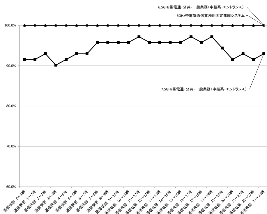
図表一九-4-5 「通信状態」のシステム別比較 (6GHz 帯電気通信業務用固定無線システム、6.5GHz 帯電通・公共・一般業務(中継系・エントランス)、 7.5GHz 帯電通・公共・一般業務(中継系・エントランス))
