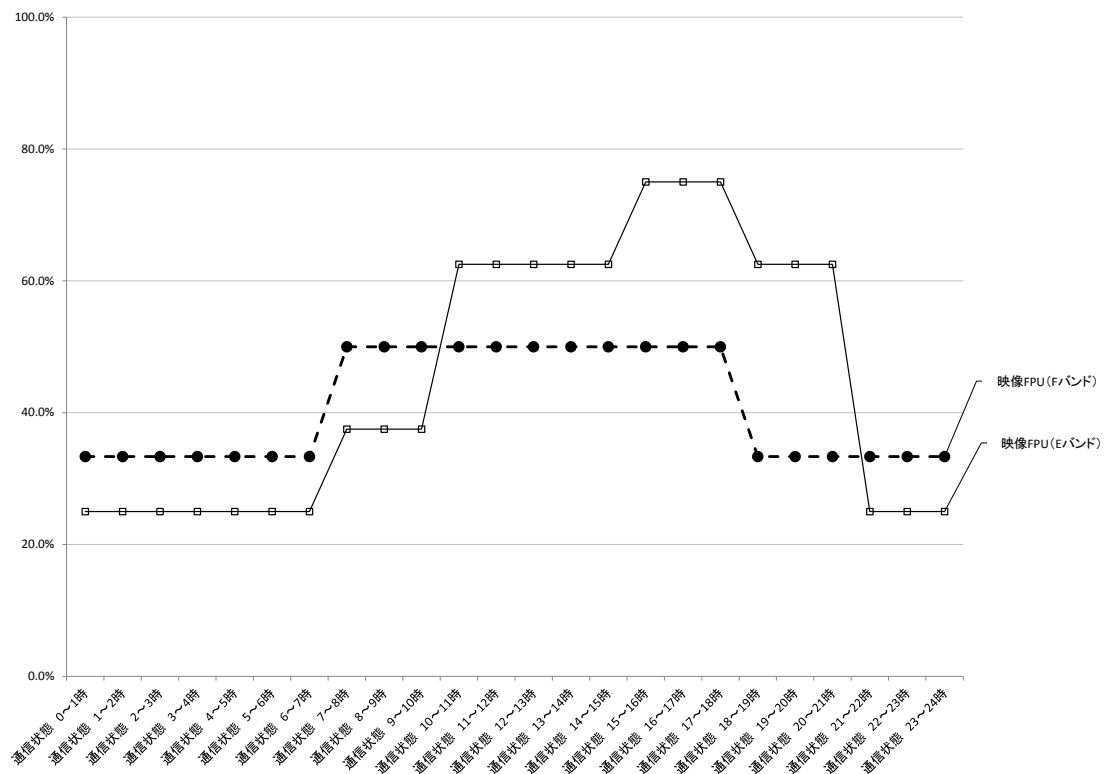
図表一信一 6-6 「通信状態」のシステム別比較（映像 FPU（E バンド）、映像 FPU（F バンド）、映像 FPU（G バンド））
