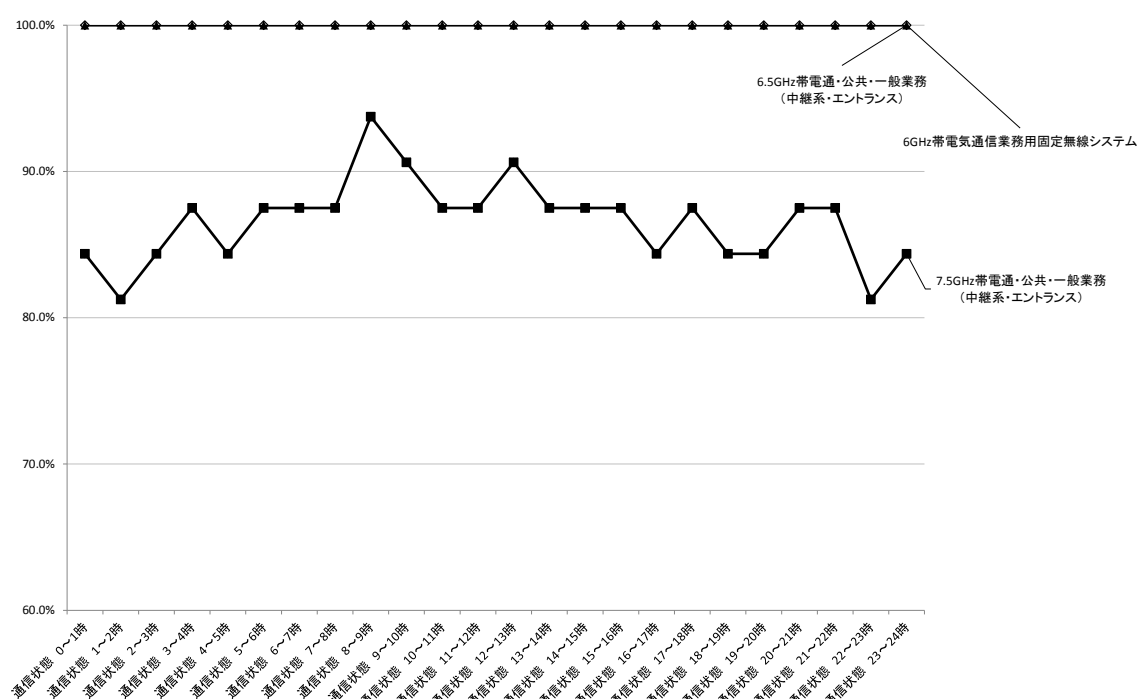
図表一海一4一5「通信状態」のシステム別比較 (6GHz帯電気通信業務用固定無線システム、6.5GHz帯電通・公共・一般業務(中継系・エントランス)、 7.5GHz帯電通・公共・一般業務(中継系・エントランス))
