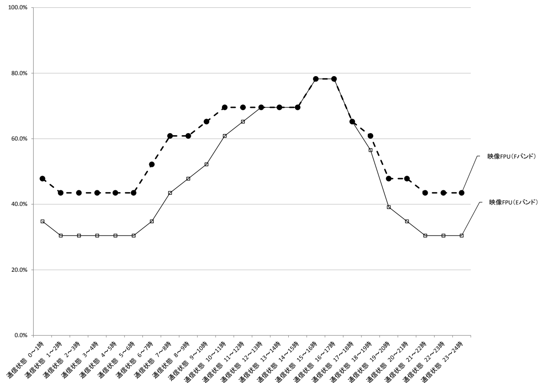
図表一東－６－６ 「通信状態」のシステム別比較（映像 FPU（E バンド）、映像 FPU（F バンド）、映像 FPU（G バンド））
