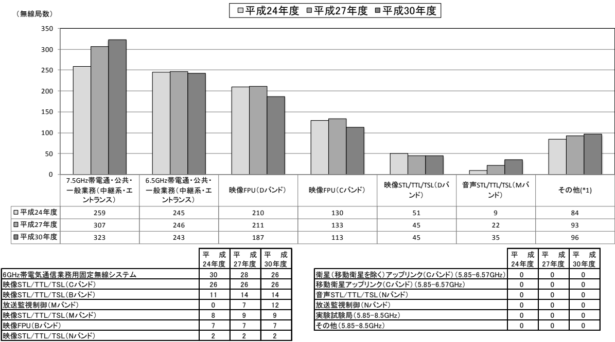
図表一四一四一四 無線局数の推移のシステム別比較
