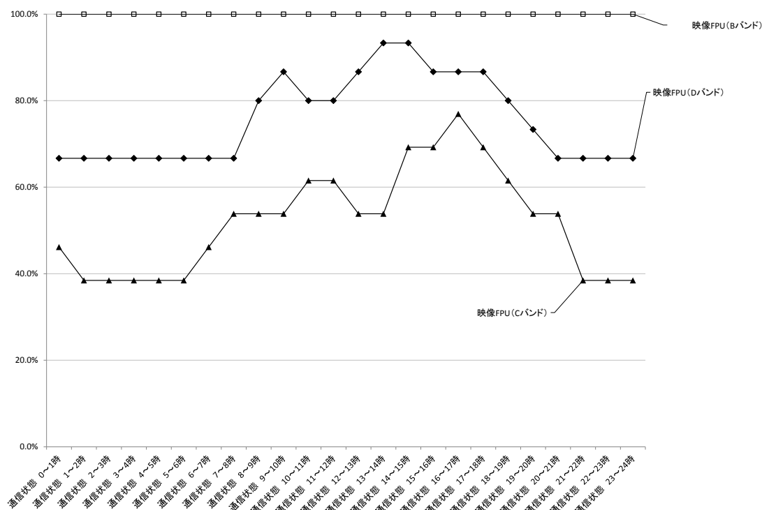
図表一東-4-7 「通信状態」のシステム別比較（映像 FPU（B バンド）、映像 FPU（C バンド）、映像 FPU（D バンド））
