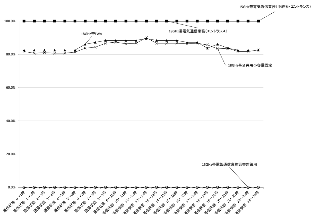
図表一全一七ー六 「通信状態」のシステム別比較（15GHz 帯電気通信業務（中継系・エントランス）、15GHz 帯電気通信業務災害対策用、15GHz 帯電気通信業務テレビ伝送用、18GHz 帯公共用小容量固定、18GHz 帯 FWA、18GHz 帯電気通信業務（エントランス））
