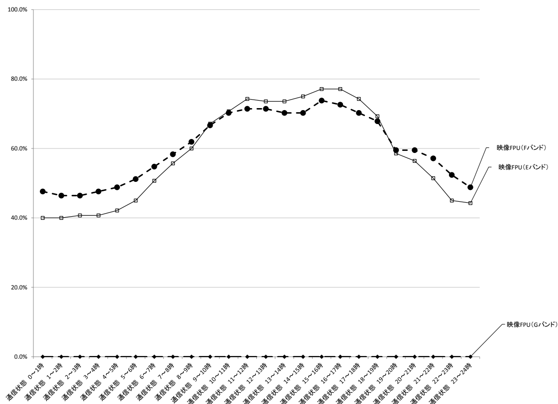
図表－全－6－6 「通信状態」のシステム別比較（映像 FPU（E バンド）、映像 FPU（F バンド）、映像 FPU（G バンド））
