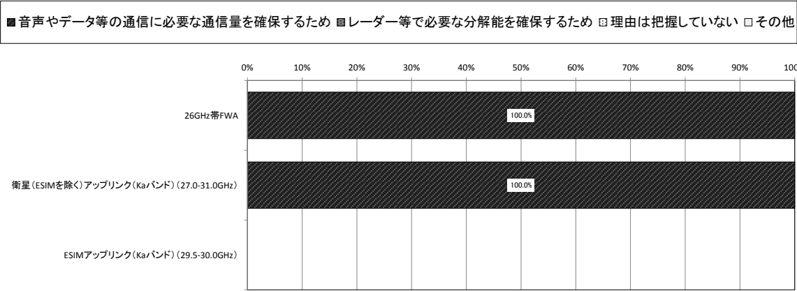
図表一九ー九ー九 「電波の容量」のシステム別比較
