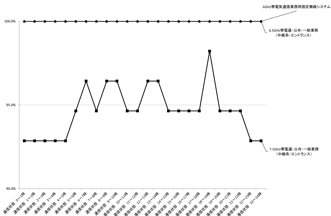
図表一中-4-5 「通信状態」のシステム別比較 (6GHz帯電気通信業務用固定無線システム、6.5GHz帯電通・公共・一般業務(中継系・エントランス)、 7.5GHz帯電通・公共・一般業務(中継系・エントランス))
