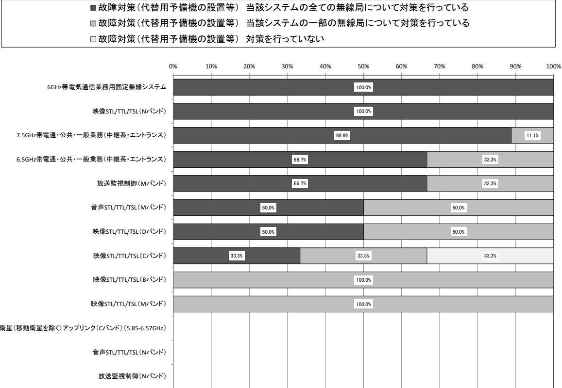
図表一陸－４－２０「故障対策（代替用予備機の設置等）」のシステム別比較
