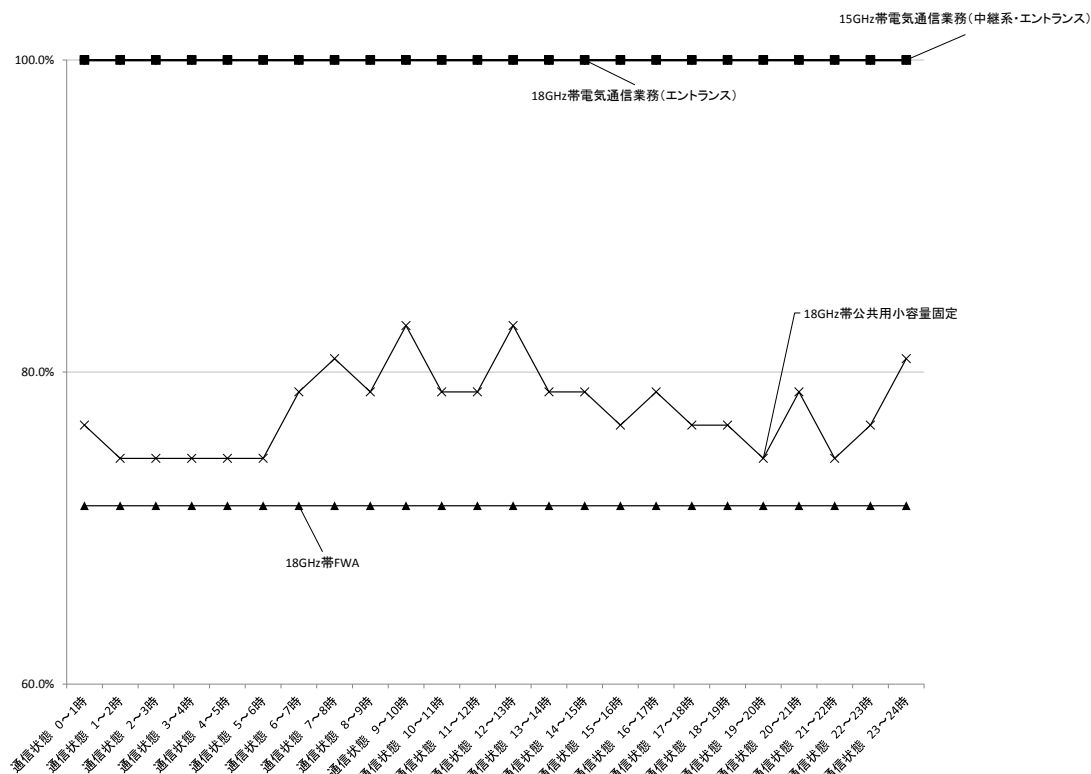
図表一東一七ー六 「通信状態」のシステム別比較（15GHz 帯電気通信業務（中継系・エントランス）、15GHz 帯電気通信業務災害対策用、15GHz 帯電気通信業務テレビ伝送用、18GHz 帯公共用小容量固定、18GHz 帯 FWA、18GHz 帯電気通信業務（エントランス））
