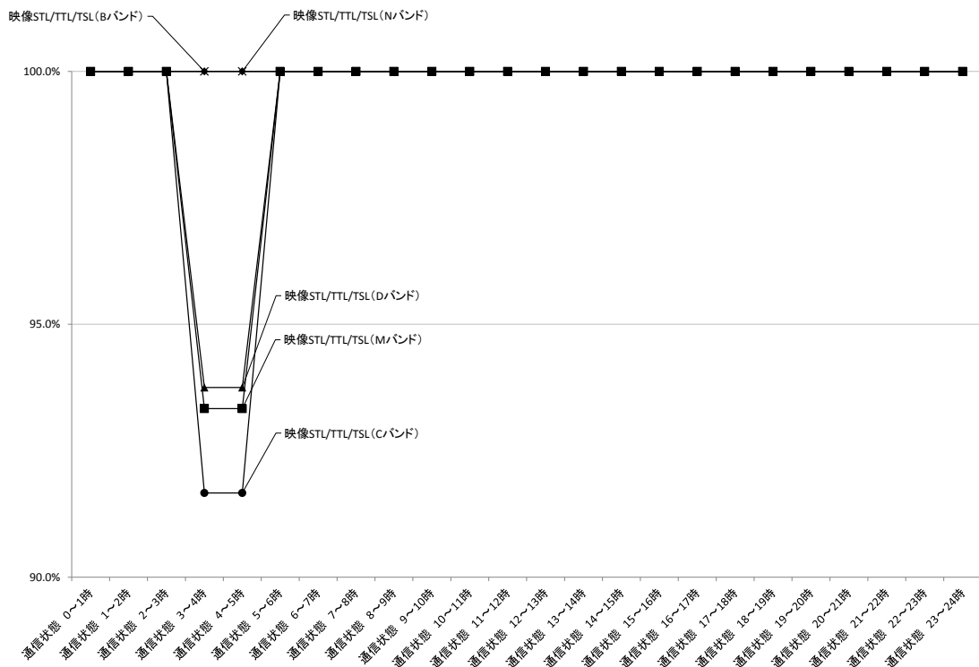
図表一中-4-8 「通信状態」のシステム別比較（映像 STL/TTL/TSL（Bバンド）、映像 STL/TTL/TSL（Cバンド）、映像 STL/TTL/TSL（Mバンド）、映像 STL/TTL/TSL（Dバンド）、映像 STL/TTL/TSL（Nバンド））
