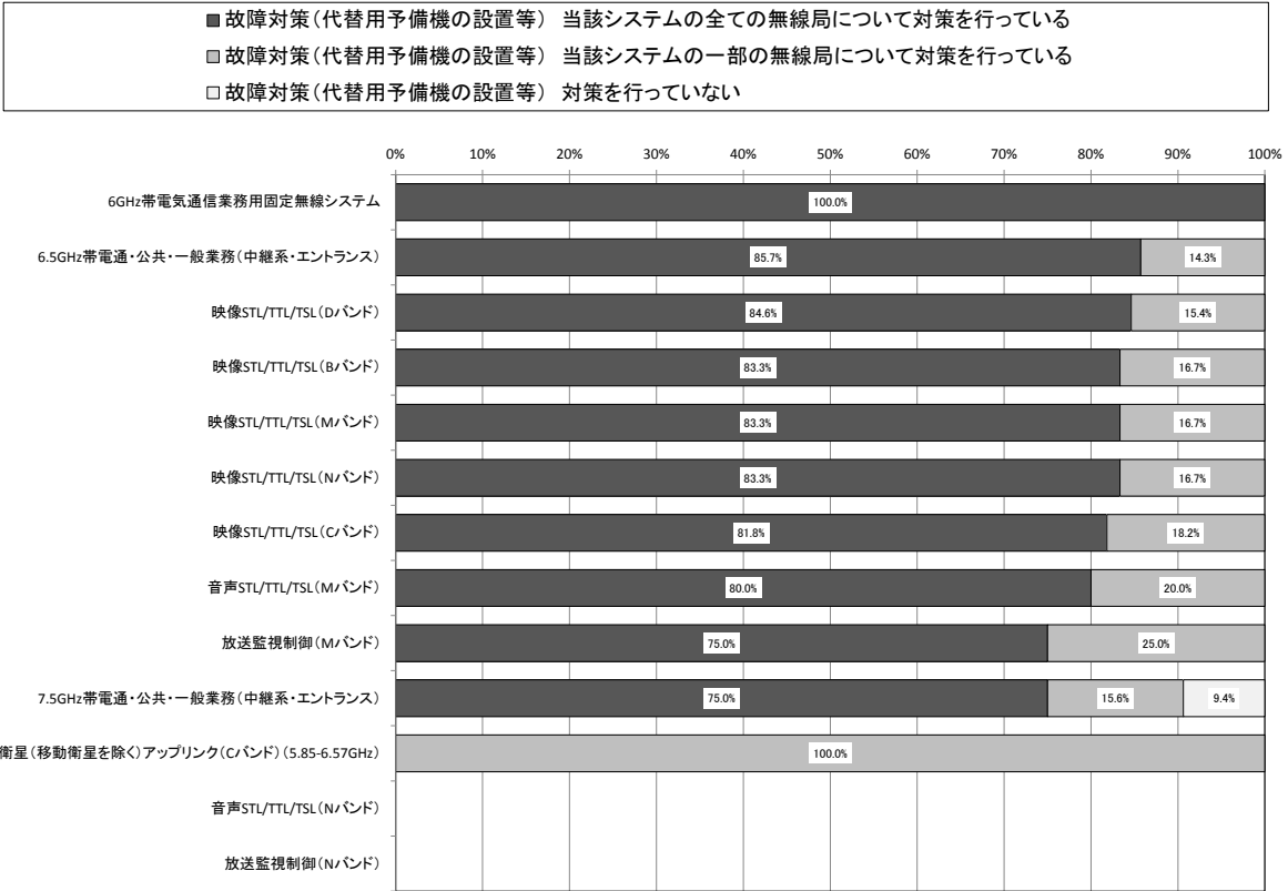
図表－海－４－２０ 「故障対策（代替用予備機の設置等）」のシステム別比較
