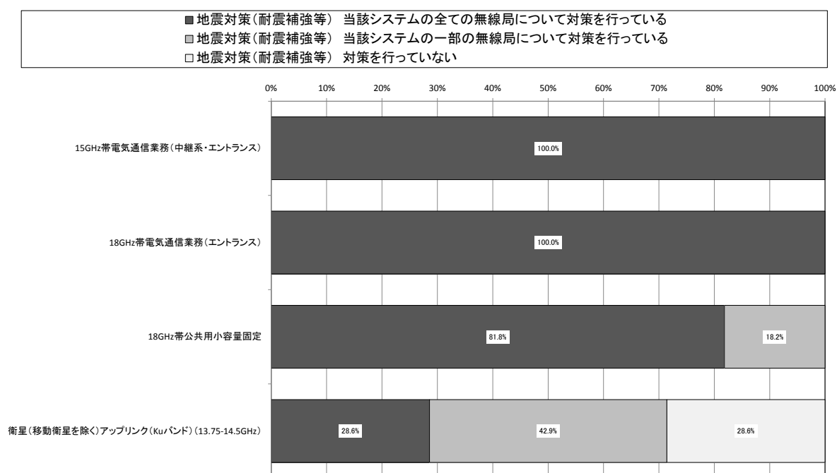
図表一近一七ー一 2 「地震対策（耐震補強等）」のシステム別比較
