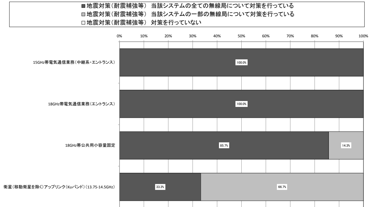
図表一陸－７－１２ 「地震対策（耐震補強等）」のシステム別比較
