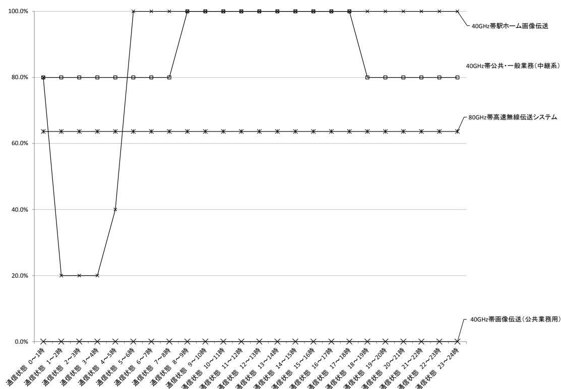
図表一関一 10-5 「通信状態」のシステム別比較(40GHz 帯画像伝送(公共業務用)、40GHz 帯公共・一般業務(中継系)、38GHz 帯 FWA、40GHz 帯駅ホーム画像伝送、80GHz 帯高速無線伝送システム、120GHz 帯映像 FPU)
