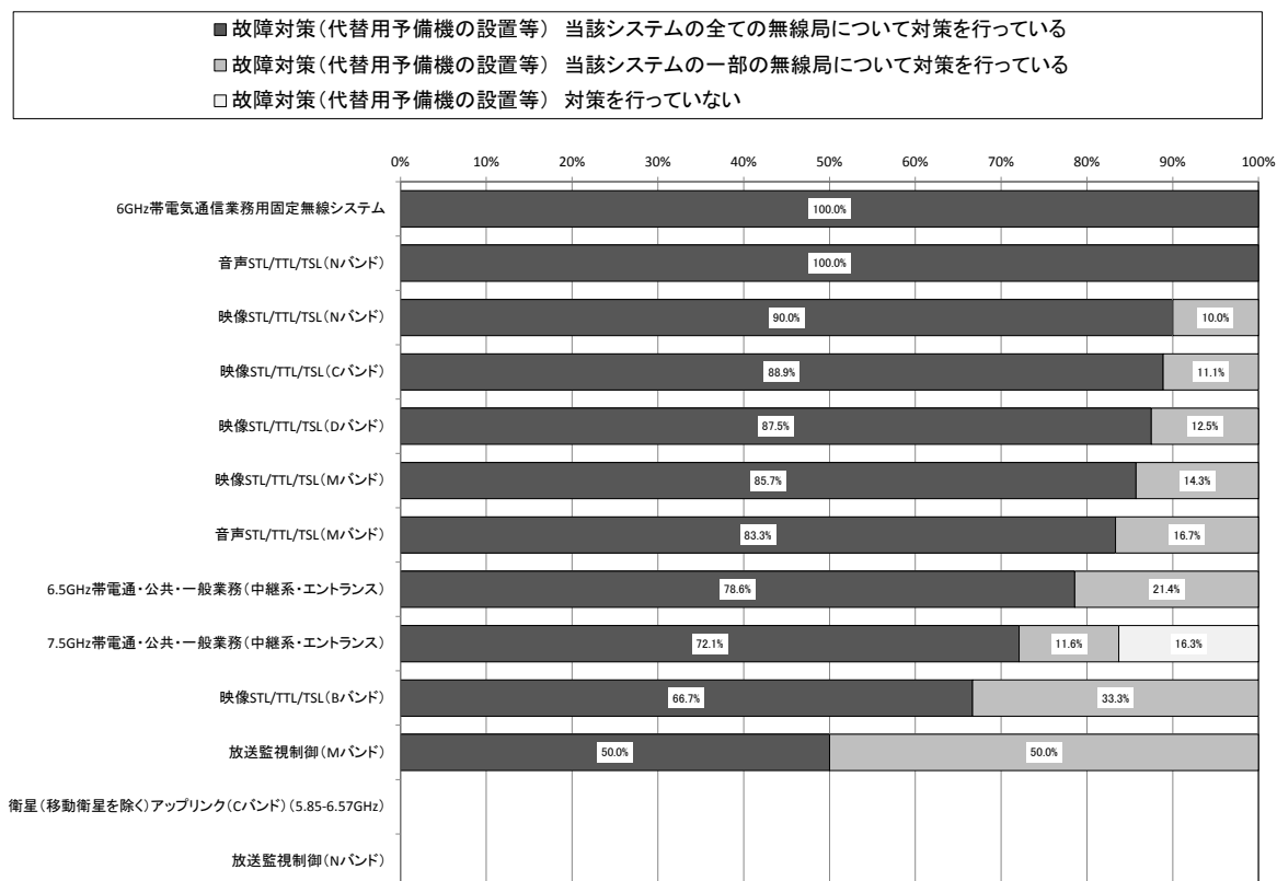
図表一近一４－２０ 「故障対策（代替用予備機の設置等）」のシステム別比較
