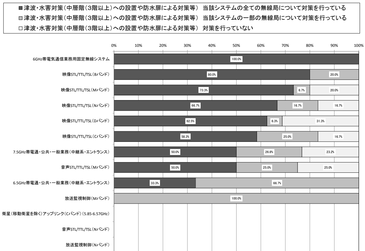
図表一中－４－１８ 「津波・水害対策（中層階（３階以上）への設置や防水扉による対策等）」のシステム別比較
