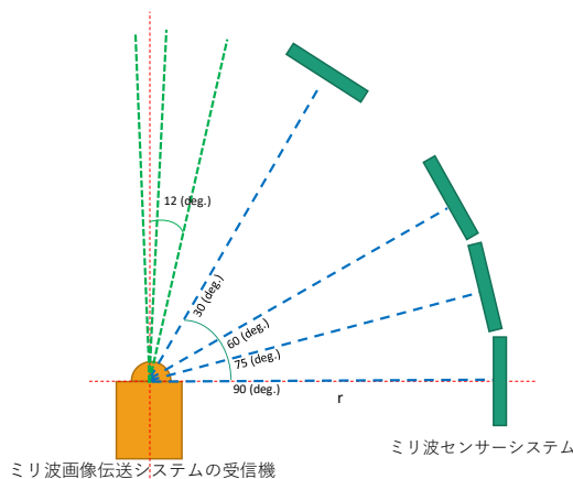
図4-3-16 ミリ波画像伝送システムの受信機
