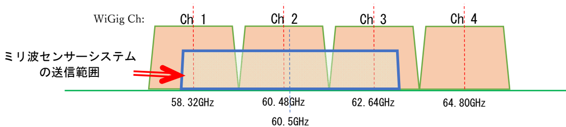
図 4-3-8 実機検証利用帯域概略図
