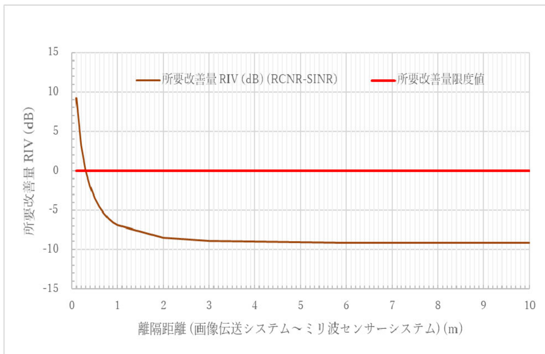
図 4-3-20 離隔距離を変えた場合所要改善量
