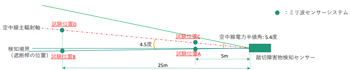
図 4-3-25 踏切障害物検知装置との干渉検討における配置図
