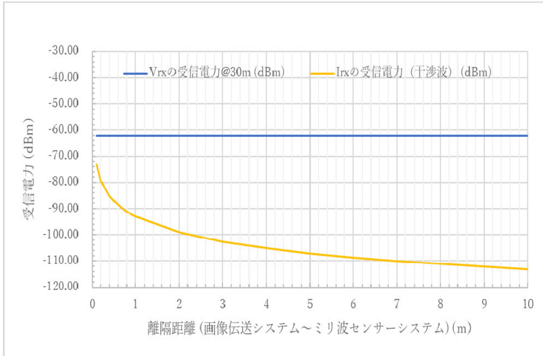
図 4-3-19 離隔距離を変えた場合の干渉波受信電力
