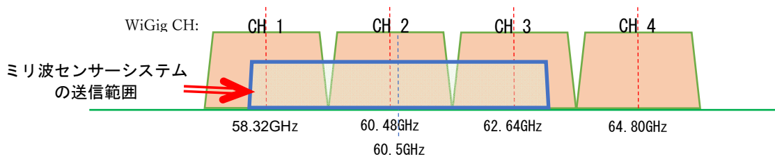
図 4-3-8 実機検証利用帯域概略図
