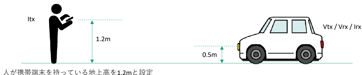
図4-3-26 自動車レーダーシステムとの干渉検討における配置図
