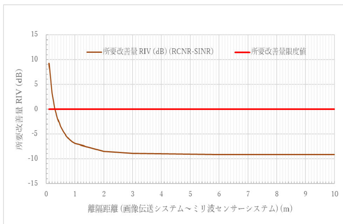
図 4-3-20 離隔距離を可変した場合所要改善量
