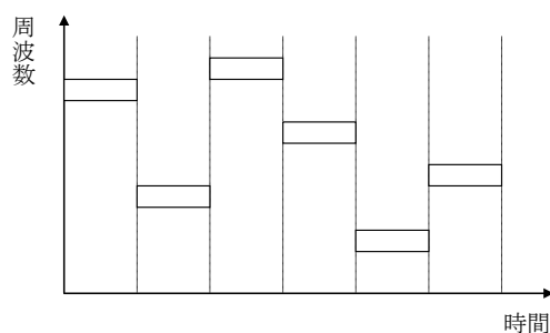
図1-3 周波数ホッピングのイメージ
