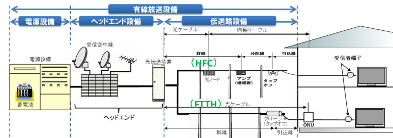
図2-2-3-1 有線放送に関する設備の構成例
