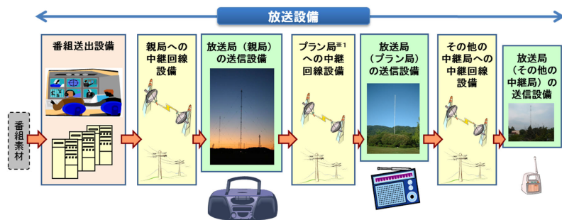
図2-2-1-2 中波放送に関する設備の構成例
