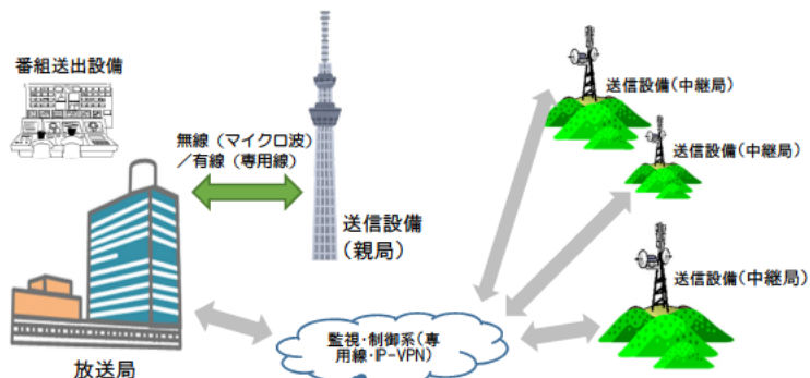
図3-2-2-1 放送ネットワーク 監視・制御設備系の構成例
