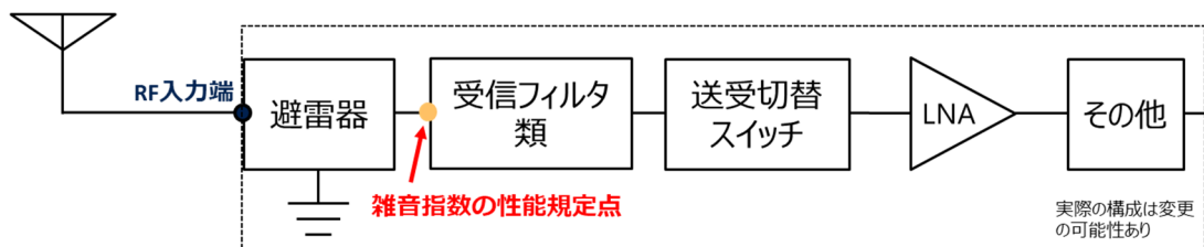
図 3-4 雑音指数の性能規定点の例
