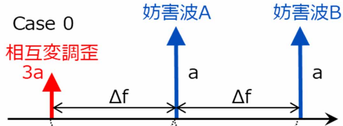
図 9-2 近傍妨害波と遠方妨害波の組合せ (Case 0)
