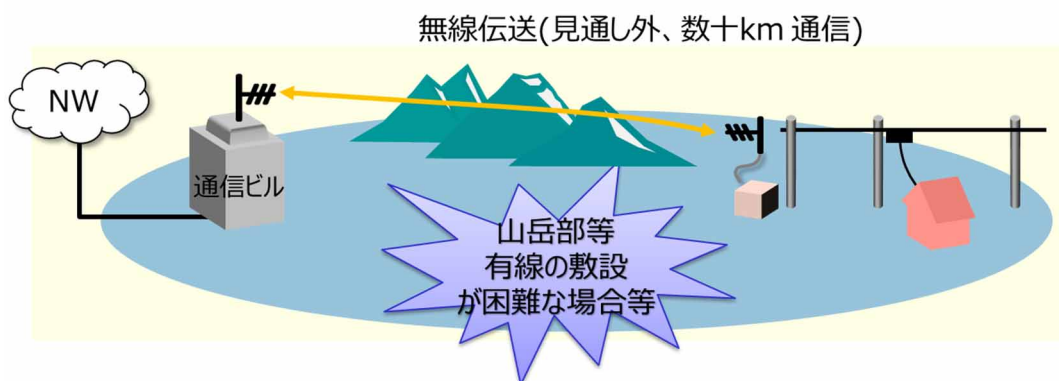
図 1-1 現行の VHF 帯加入者系無線システムの回線提供例
