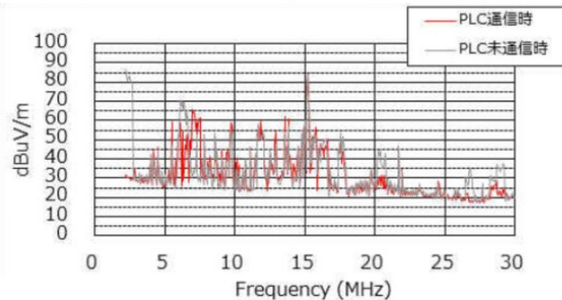
航海中の船舶での鋼船に設置されたPLC設備からの磁界強度（等価電界強度表示）の測定例
