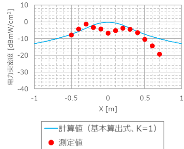
3.5GHz帯, 高さ0.1m地点の水平方向 (Y=0, Z=0.1)
