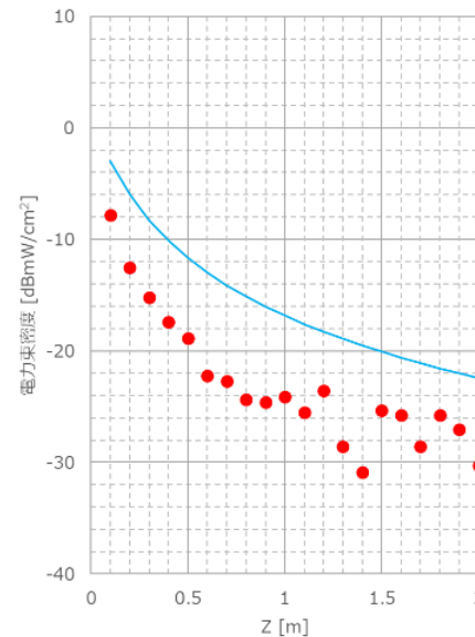
1.5GHz帯, 空中線の直上 (X=0, Y=0)
