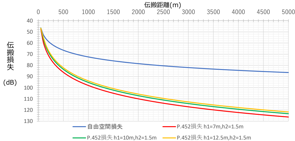
図1. ITU-R P.452及び自由空間伝搬損失特性
