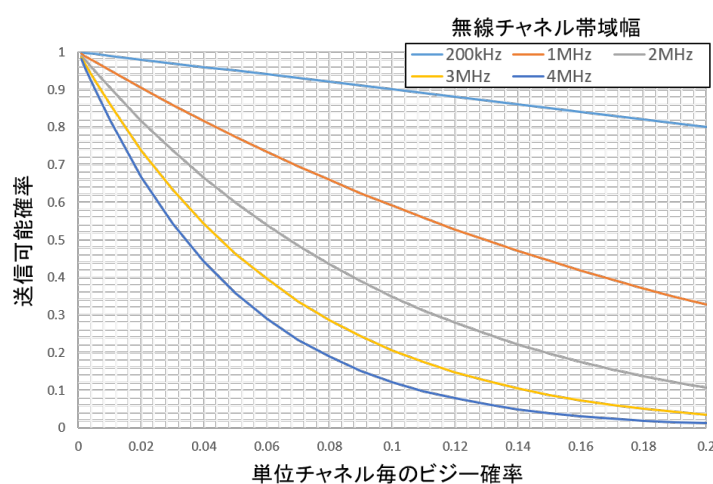
図 2-7 単位チャンネル毎のビジー確率と送信可能確率の関係
