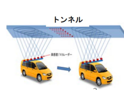
非破壊検査
