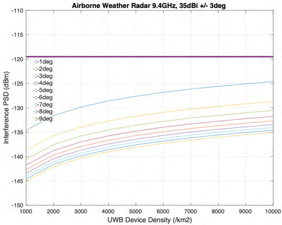
図5-17 高度26m条件での計算結果（アンテナ特性2）
