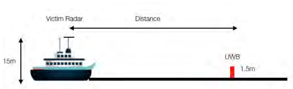
図5-4 Xバンド船舶レーダーでのシングルエントリー シミュレーションモデル
