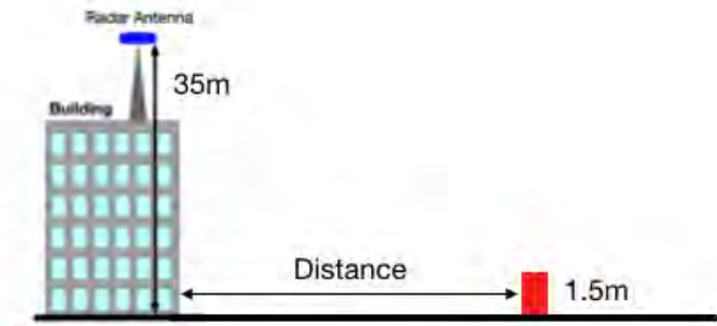
図5-1 沿岸監視レーダーでのシングルエントリー シミュレーションモデル
