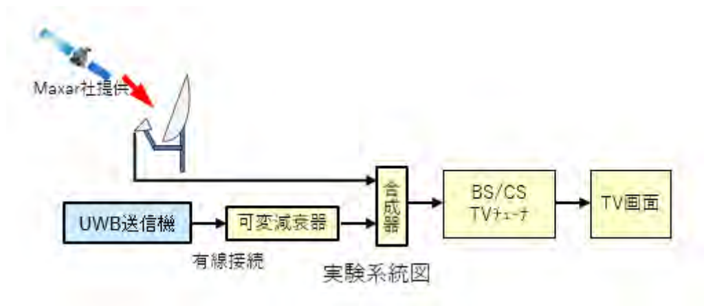
図6-18 C/I評価実験系統図
