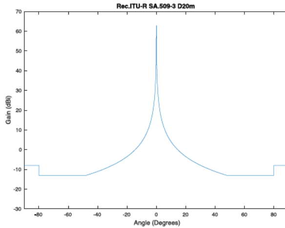
図 3-18 勧告 ITU-R SA.509-3 のアンテナ特性
