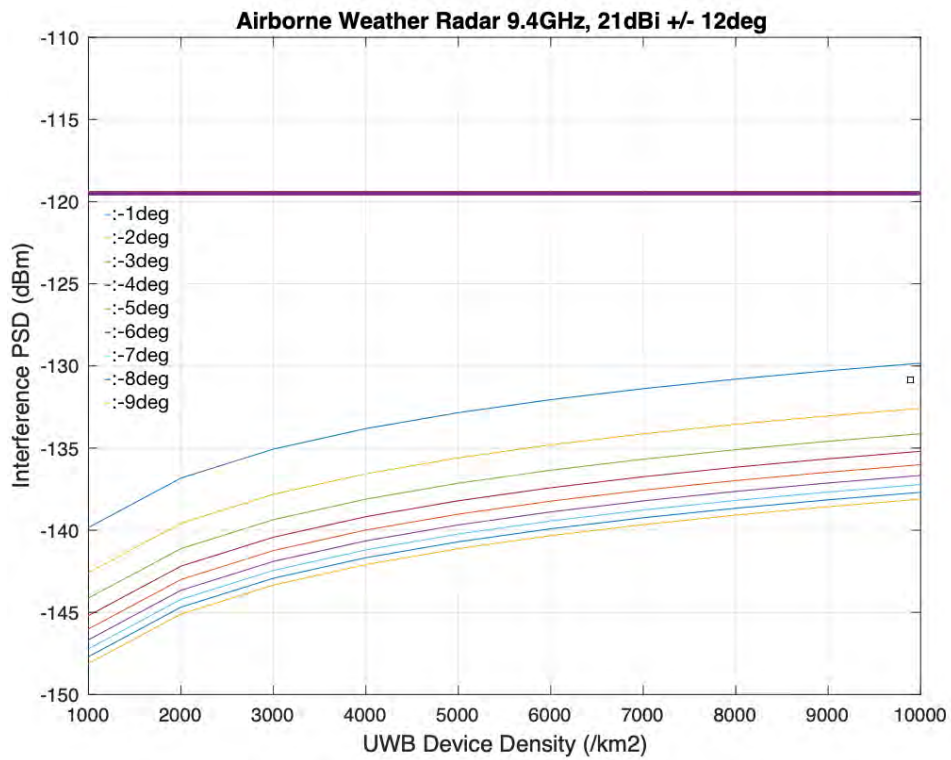
図5-15 高度1050m条件での計算結果（アンテナ特性1）
