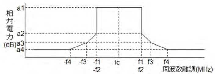
図1 送信信号特性
