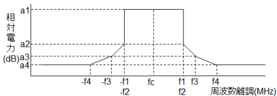
図2-4 送信信号特性
