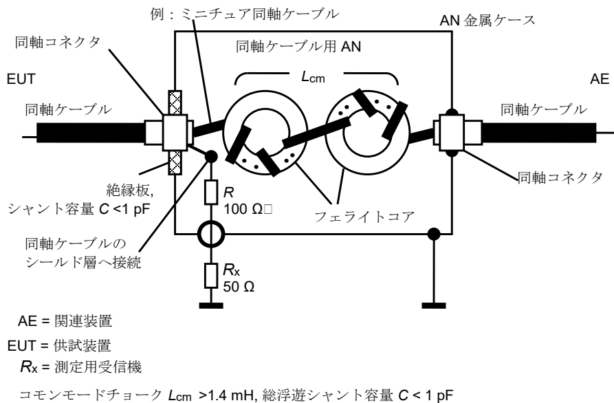
図 F.1 - 同軸ケーブル用 AN の例
