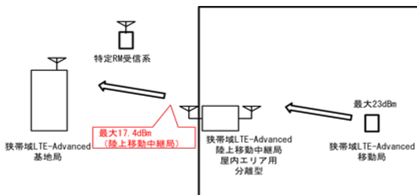
図 2. 4. 4. 1-11 狭帯域 LTE-Advanced 陸上移動中継局(屋内用分離型)からの与干渉イメージ
