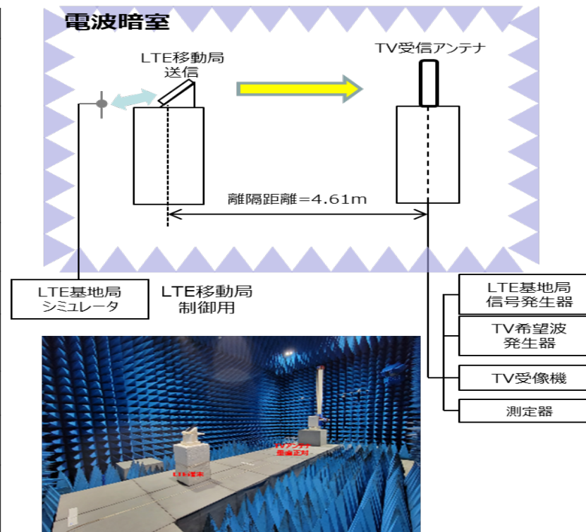
図 2. 3. 4. 1 - 3 実証実験の試験構成概要
