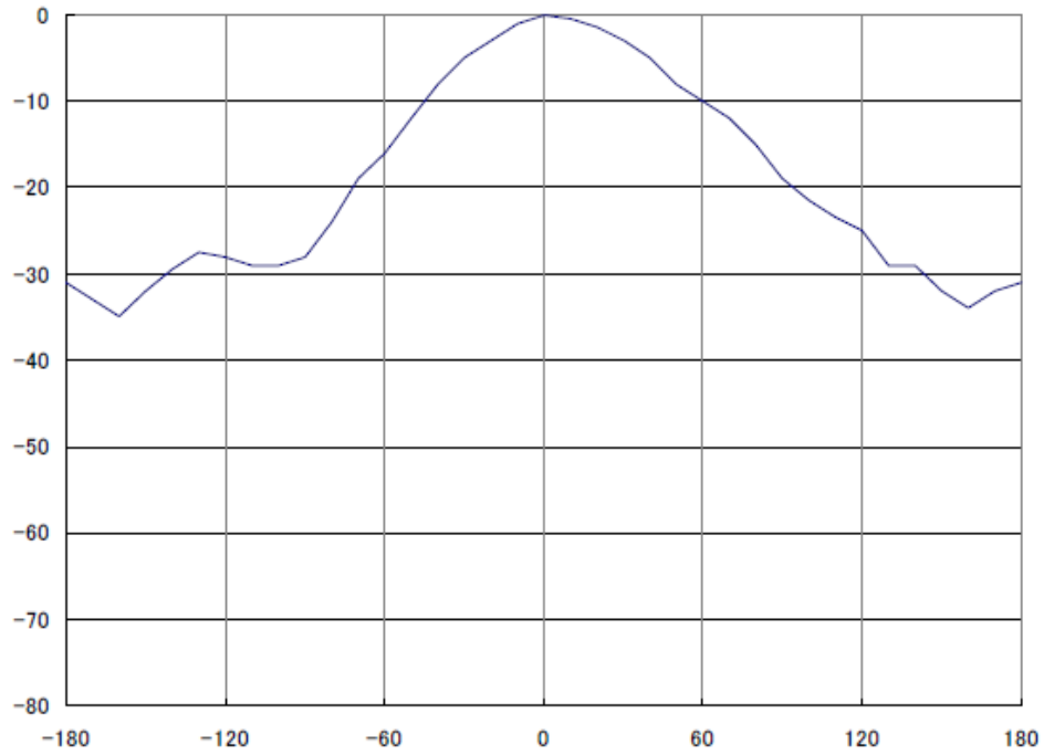
図 2. 2. 3-4 狭帯域 LTE-Advanced 陸上移動中継局（屋内エリア用）基地局対向器アンテナ指向特性（水平）
