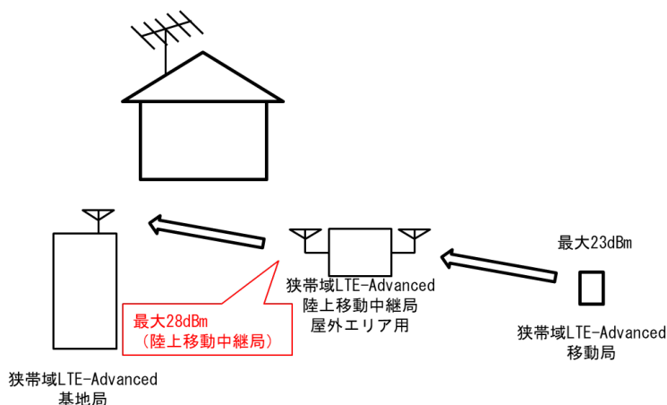
図 2. 3. 4. 1-10 狭帯域 LTE-Advanced 陸上移動中継局（屋外用）からの与干渉イメージ
