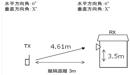
検討モデル案③ 家庭TV 簡易ANTブースタ無 (5mH)
