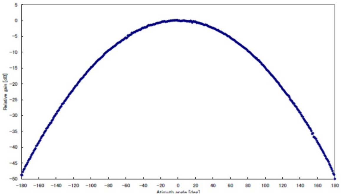
図 2. 2. 1-1 狭帯域 LTE-Advanced 基地局の送受信アンテナパターン (水平面) (「携帯電話等高度化委員会報告」(平成 24 年 2 月 17 日) 図 2. 2. 1-2 を引用)
