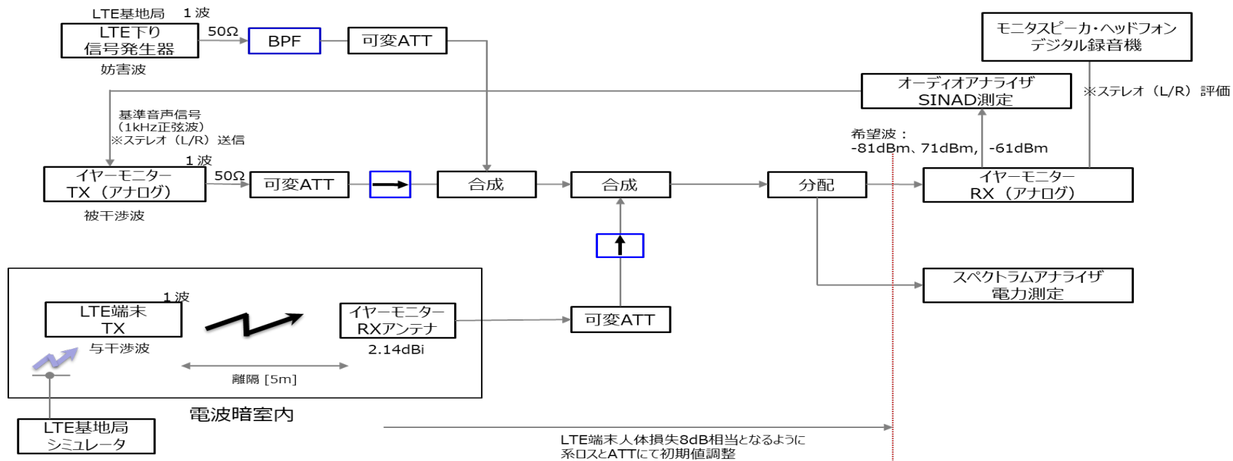
(e) RM-5の実験系 (イヤーマニター)
