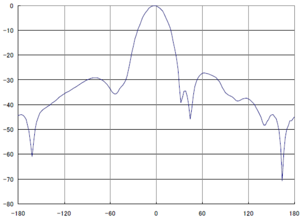
図2. 2. 3-3 狭帯域 LTE-Advanced 陸上移動中継局（屋外エリア用）基地局対向器アンテナ指向特性（垂直）
