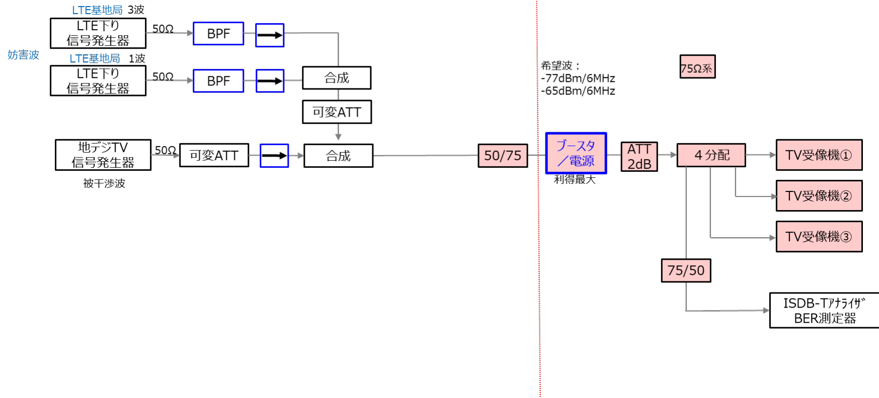
(b) 事前確認 TV-01 の実験系 (ブースタ)
