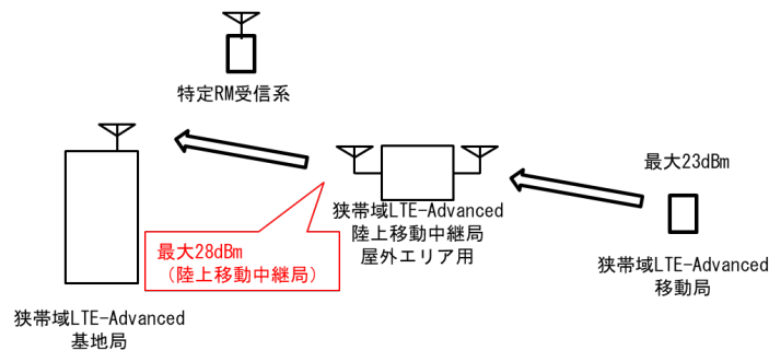
図 2. 3. 4. 1-9 狭帯域 LTE-Advanced 陸上移動中継局(屋外用)からの与干渉イメージ
