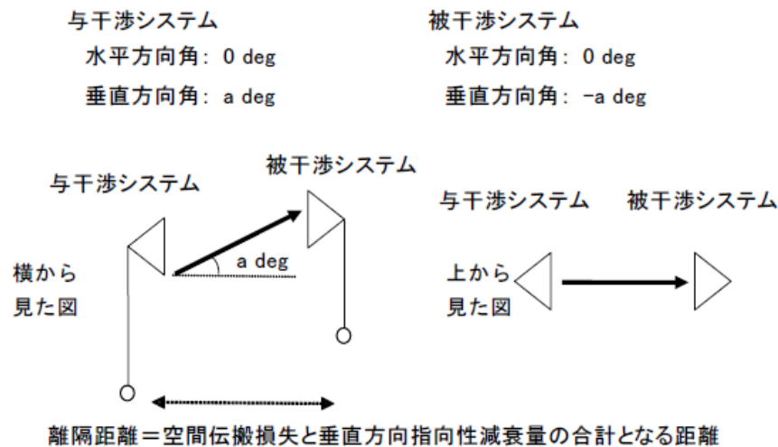
図2. 1. 2-1 1対1対向モデル
