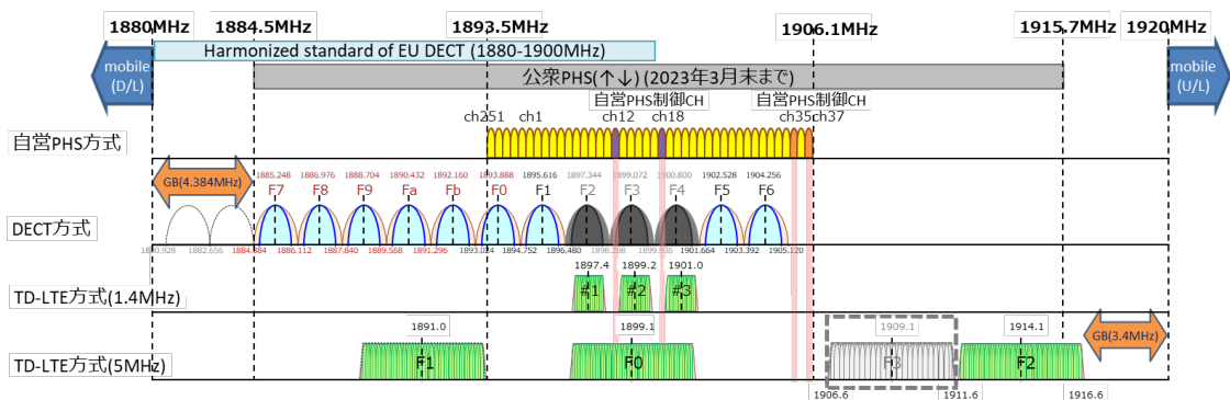
参图 3-4 周波数配置案(ケース 3)
