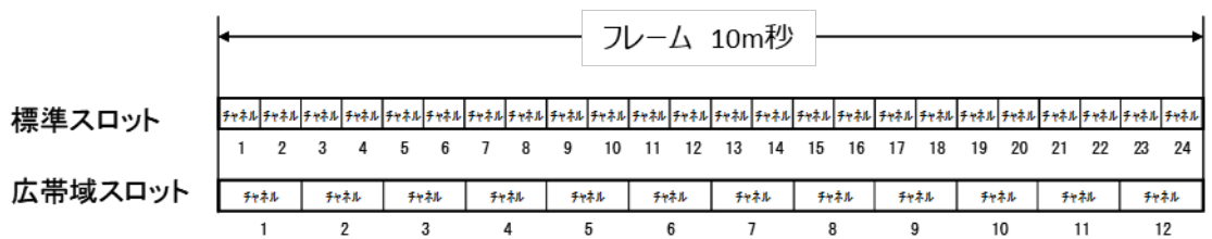
図4. 2-2 DECT方式のフレーム構成
