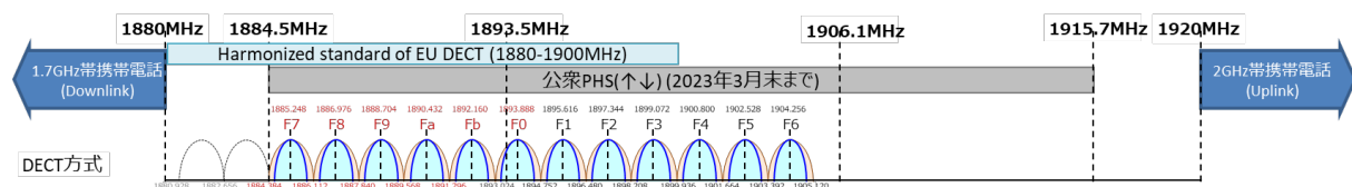
図 1. 2 - 1 DECT 方式の周波数
