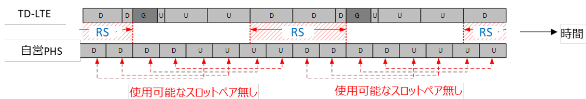
参図 3-8 TD-LTE 方式と自営 PHS 方式の時間軸上の配置
