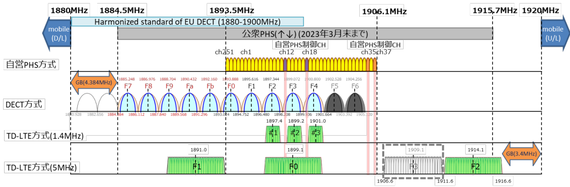
参图 3-3 周波数配置案(ケース 2)
