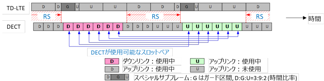
参図 3-6 TD-LTE 方式と DECT 方式の時間軸上の配置
