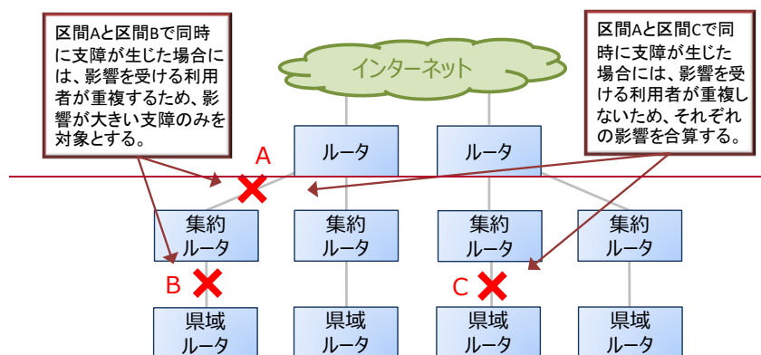
<図1-11>複数の設備が同一原因で同時期に故障した場合における影響の考え方
