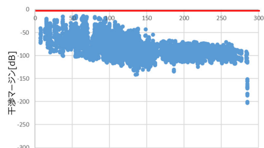
図3. 3. 1. 4-2 4 下りの干渉マージン(短時間) (常陸大宮、8台/局、4dBm/MHz、屋外設置率 50%) ※グラフは屋内設置した5Gレピータも含む
