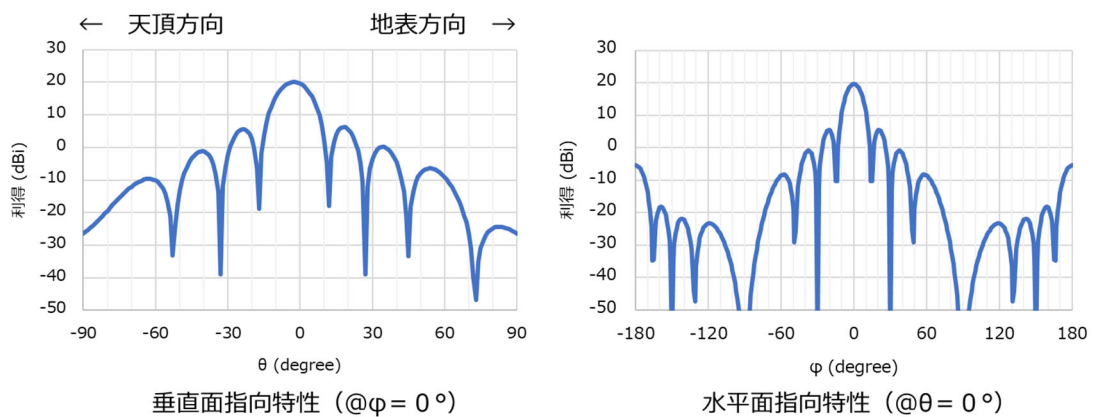
図 4. 3. 1-5 検討 B: 生成された固定アンテナパターン
