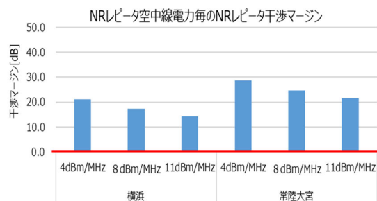
図 3. 3. 1. 4-5 送信電力ごとの干渉マージン(単体)
