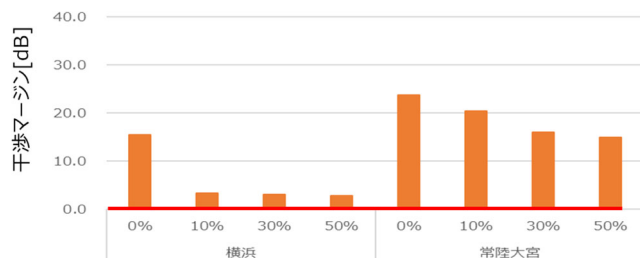
図3.3.1.4-9 屋外設置比率ごとの干渉マージン(総合)
