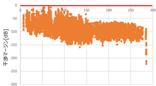
図3. 3. 1. 4-2 3 上りの干渉マージン(短時間) (常陸大宮、8台/局、4dBm/MHz、屋外設置率 50%) ※グラフは屋内設置した5Gレピータも含む
