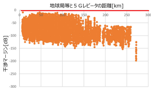
図3. 3. 1. 4-2 1 上りの干渉マージン(短時間) (横浜、8台/局、4dBm/MHz、屋外設置率 50%) ※グラフは屋内設置した5Gレピータも含む
