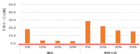
図 3. 3. 1. 4-3 屋外設置比率ごとの干渉マージン(単体)
