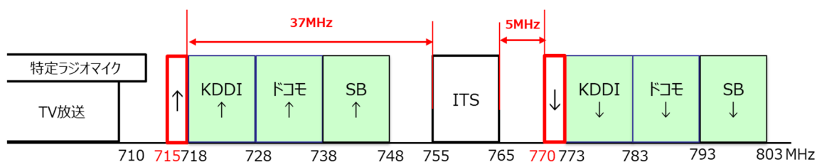
図 2. 5. 1 - 1 狭帯域 LTE-Advanced システムと ITS の周波数配置
