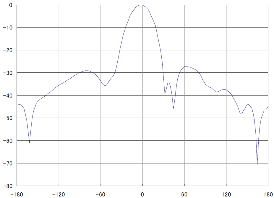
図2. 2. 3 - 3 狭帯域 LTE-Advanced 陸上移動中継局（屋外エリア用） 基地局対向器アンテナ指向特性（水平） （「携帯電話等高度化委員会報告」（平成 24 年 2 月 17 日）図 2. 2. 3 - 3 を引用）
