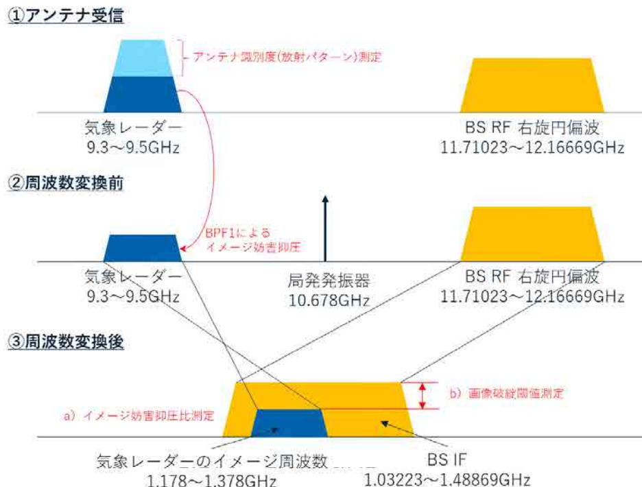
図 4. 1 - 2 気象レーダーからBS受信への干渉メカニズム
