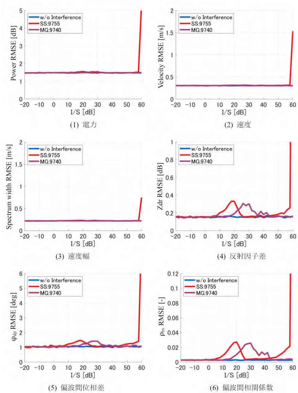
図 2. 2-6 降水エコー推定精度
