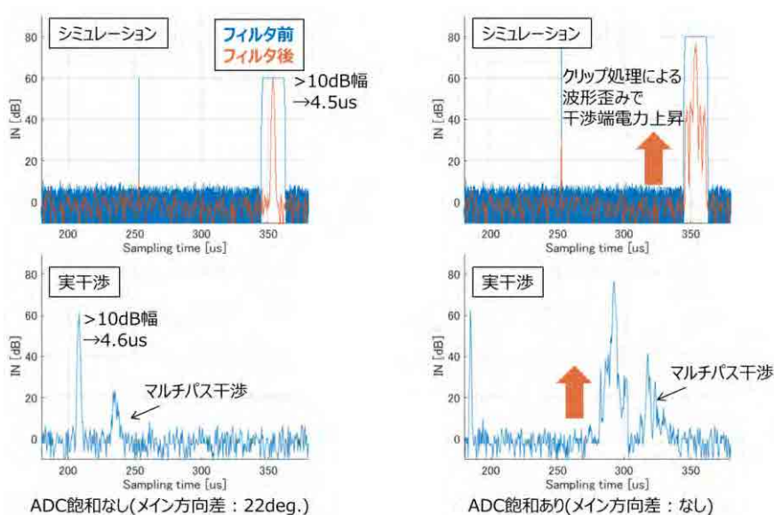
図 2. 2-13 干渉波形
