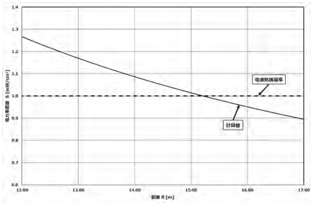
図2 X 帯高性能型気象レーダーの電波防護指針と適合性（例）
