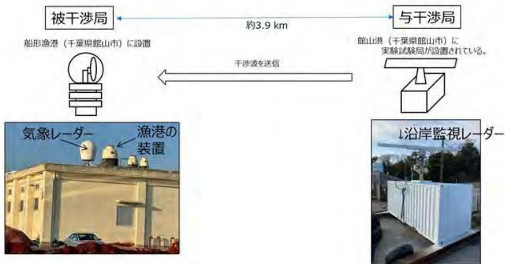
図 2. 2-10 試験環境
