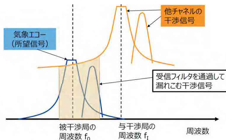
図 2. 1-1 4 他チャネルの気象レーダー間干渉時の周波数スペクトル配置
