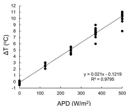
図4 電波ばく露強度APDとターゲット皮膚温度変化との関係 ばく露開始6分後の温度変化を示す(n=7-15)。点線は線形回帰モデル。(文献8より引用)
