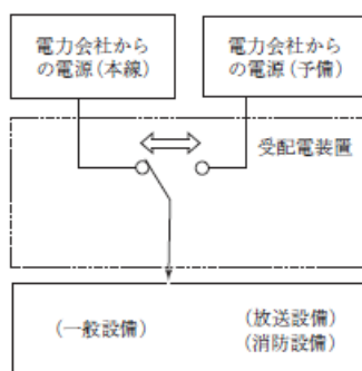
第21図 2系統受電とする場合の例
