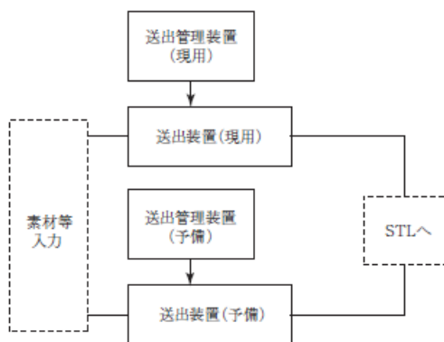
第1図 番組送出設備の現用予備構成の図
