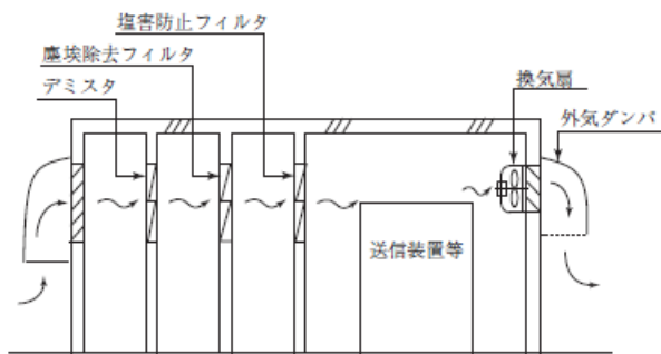
第22図 吸排気設備に対するフィルタ等の設置例
