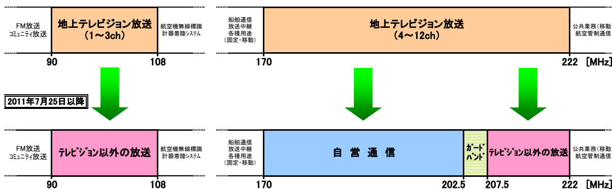
図表 4.2-7 VHF 帯（90-108MHz 及び 170-222MHz）の周波数配置案
