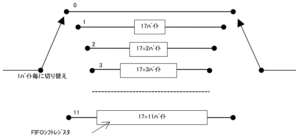
図3.5.7-1 バイトインターリーブ
