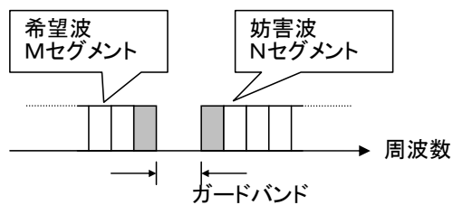
図5-52 希望波と妨害波の配置図
