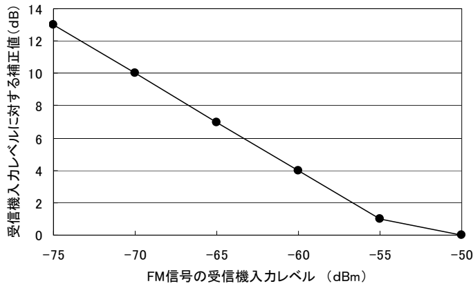
図5-3 FM信号の受信機入力レベルに対する
