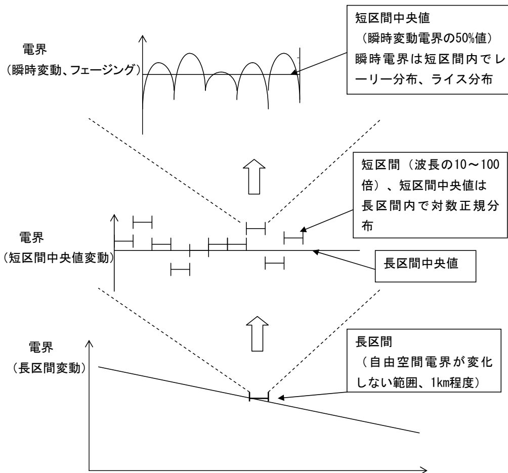
図2-1 移動受信時の電界変動
