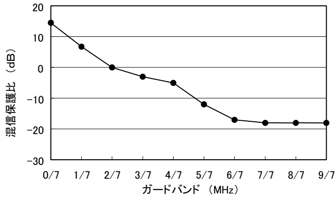
図5-44 携帯端末向けマルチメディア放送信号同士の隣接混信保護比
