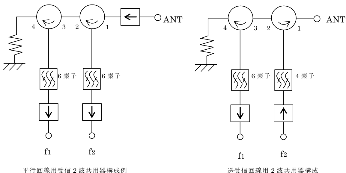
図 2-1 共用器構成例
