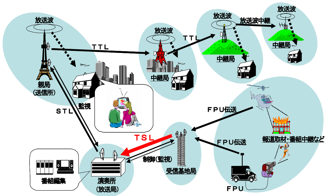
図 2 映像 TSL の例
