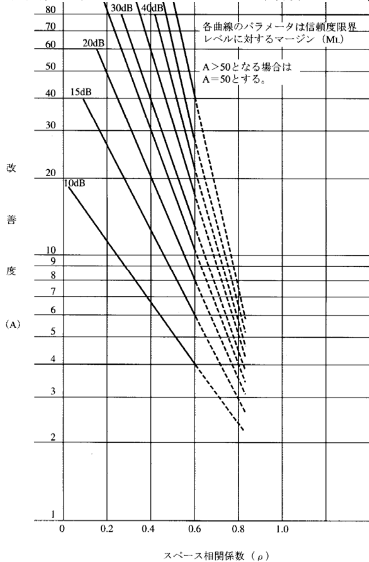
電波法関連審査基準別紙 1 別図第 46 号 スペースダイバーシチによる改善度による
