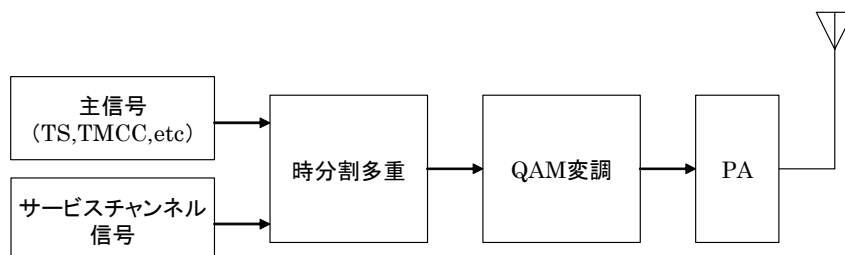
図1 TS 伝送方式のブロック図(例)
