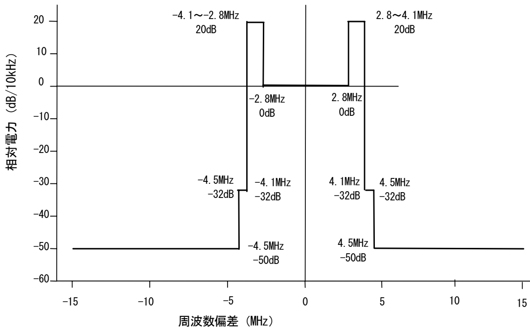
図3 送信電力スペクトル特性 (従属同期方式(低雑音方式)の場合)
