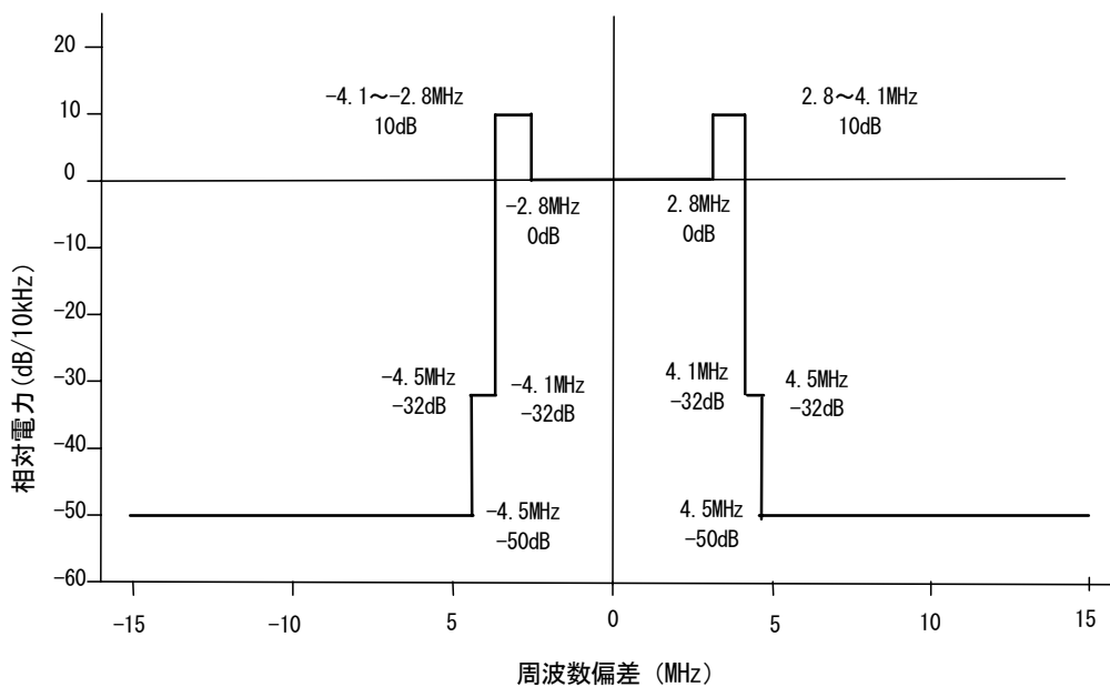
図3 送信電力スペクトル特性
