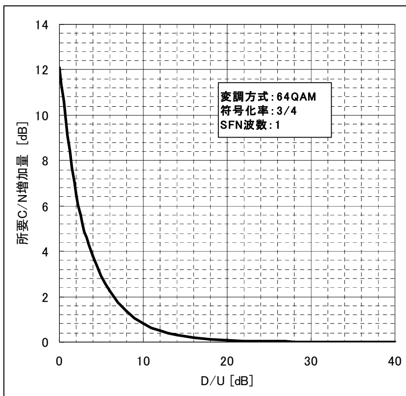
図 2. SFN 干渉波に対する D/U と所要 C/N 増加量 (ARIB TR-B14 付録 A.1.1.2 による)
