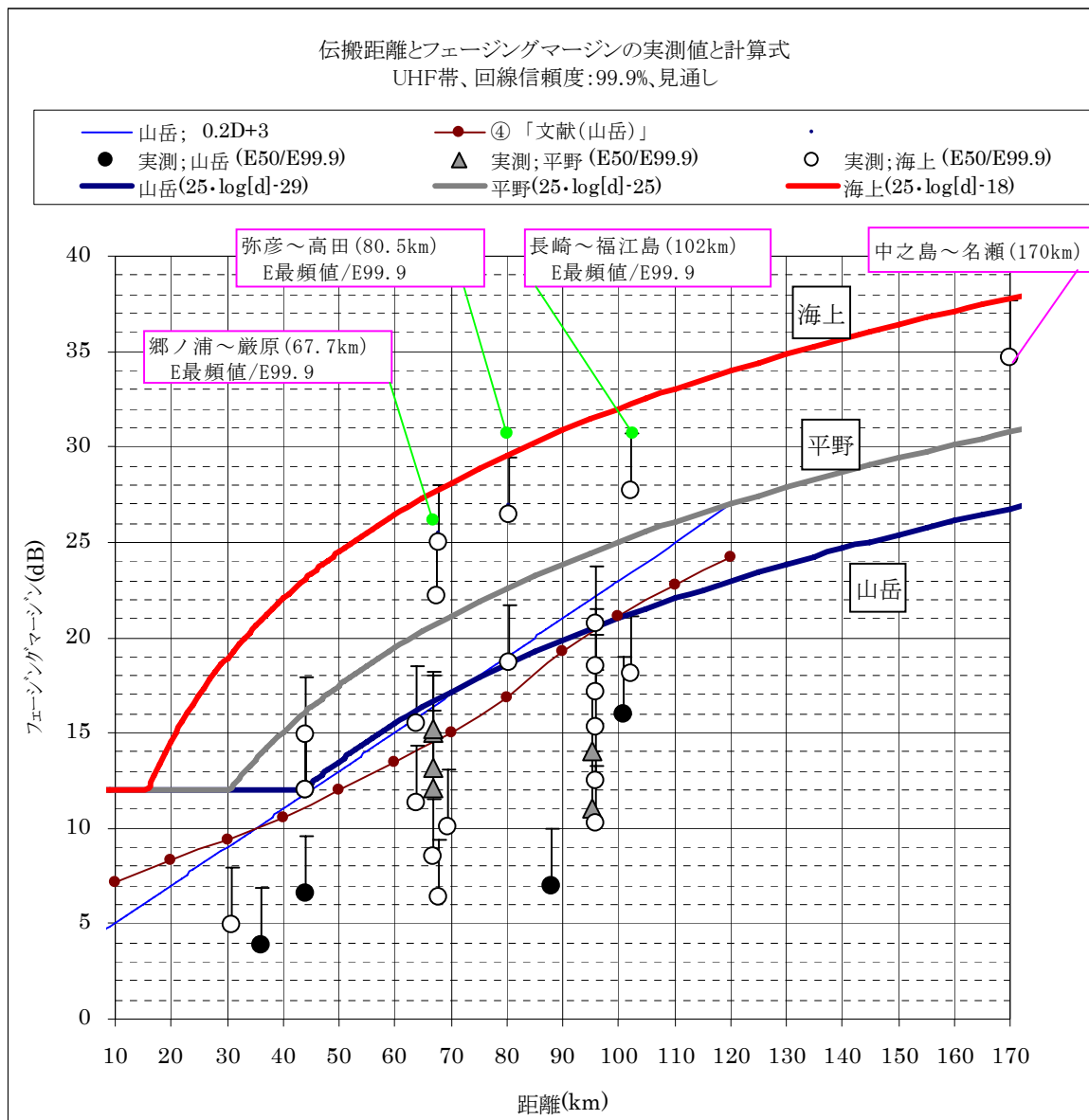
図1 実回線での伝搬距離と所要フェージングマージン (フェージング損失)との関係
