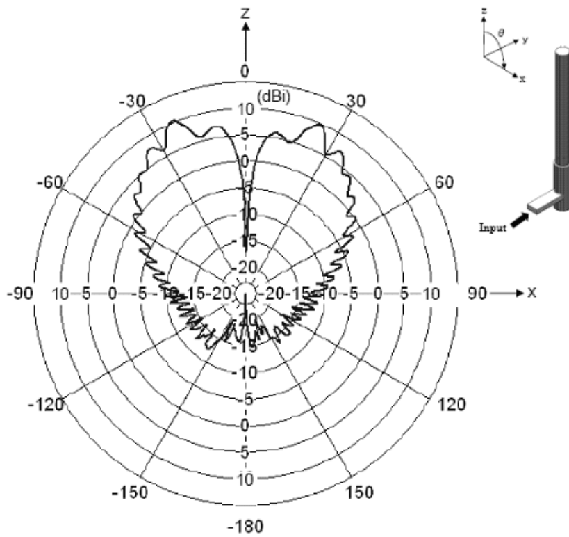
図2 誘電体ロッドアンテナの指向性(測定結果例) エラー! 参照元が見つかりません。
