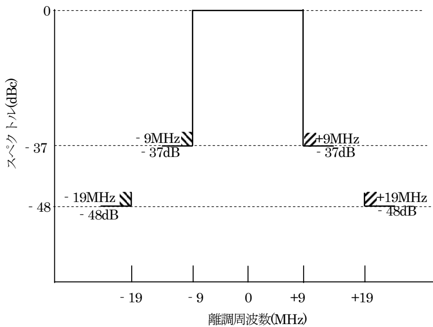
映像TSL 送信電カスペクトル特性
