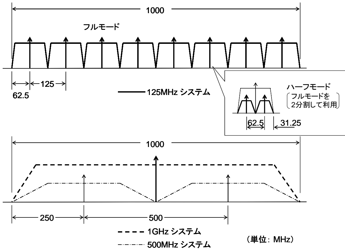
図 1 周波数配置
