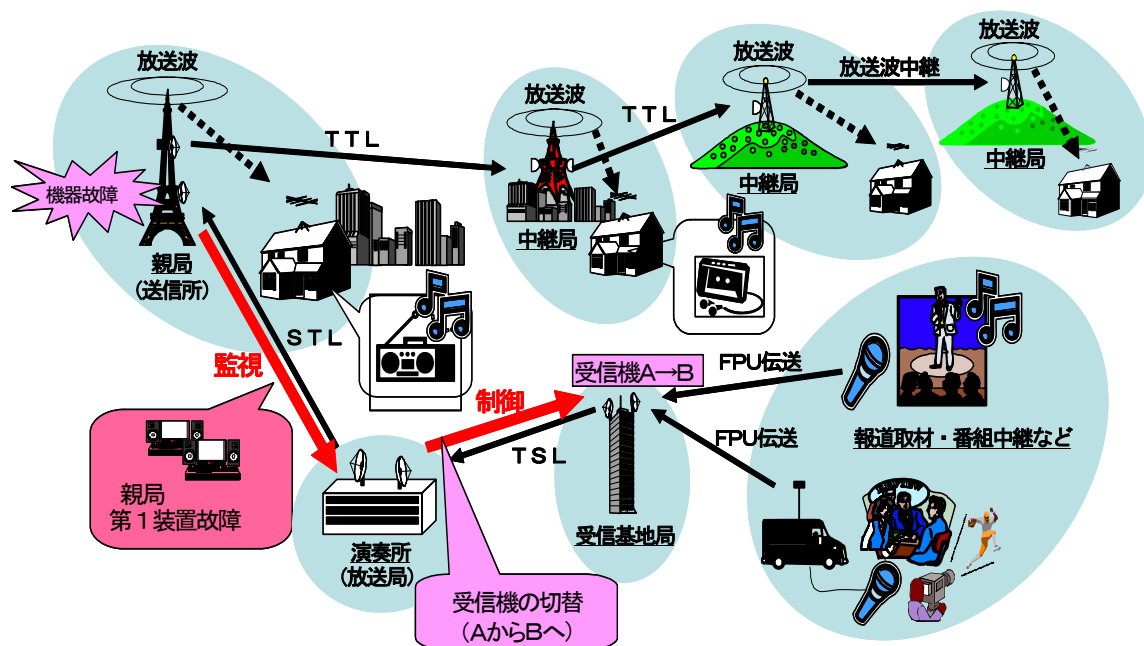
図3 監視・制御用固定回線の例
