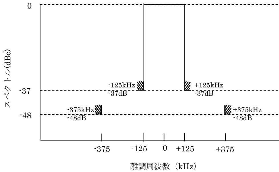
監視・制御 送信電カスペクトル
