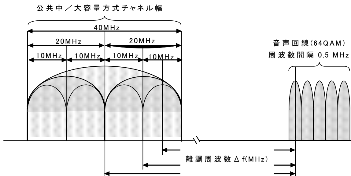
図1 公共中／大容量方式と音声回線(64QAM)の離調周波数関係
