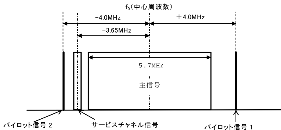
図1 伝送信号周波数配置の例
