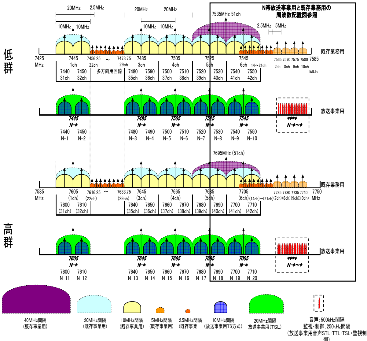
N帯(7.5GHz 帯)の周波数配置
