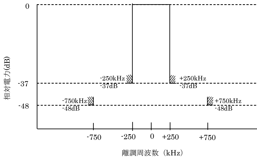
音声 STL/TTL/TSL 送信スペクトル
