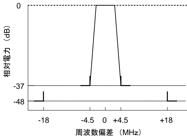
図6 送信電力スペクトル特性
