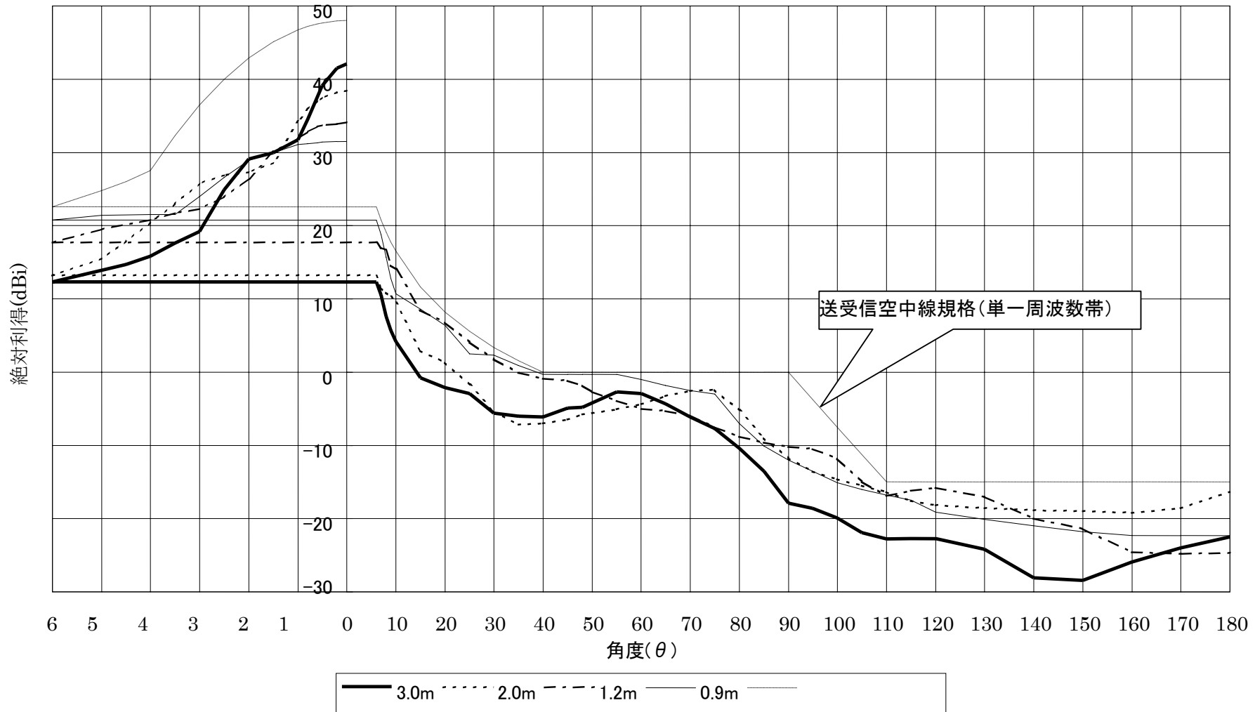
図1 M帯 パラボラアンテナ標準指向性
