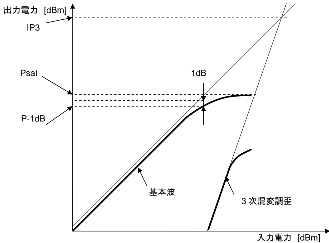
図1 P-1dB, Psat, IP3 の関係
