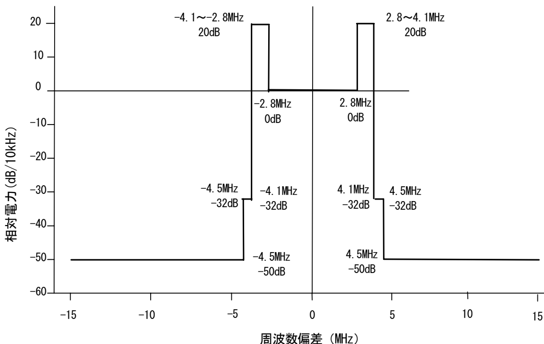
図4 送信電力スペクトル特性
