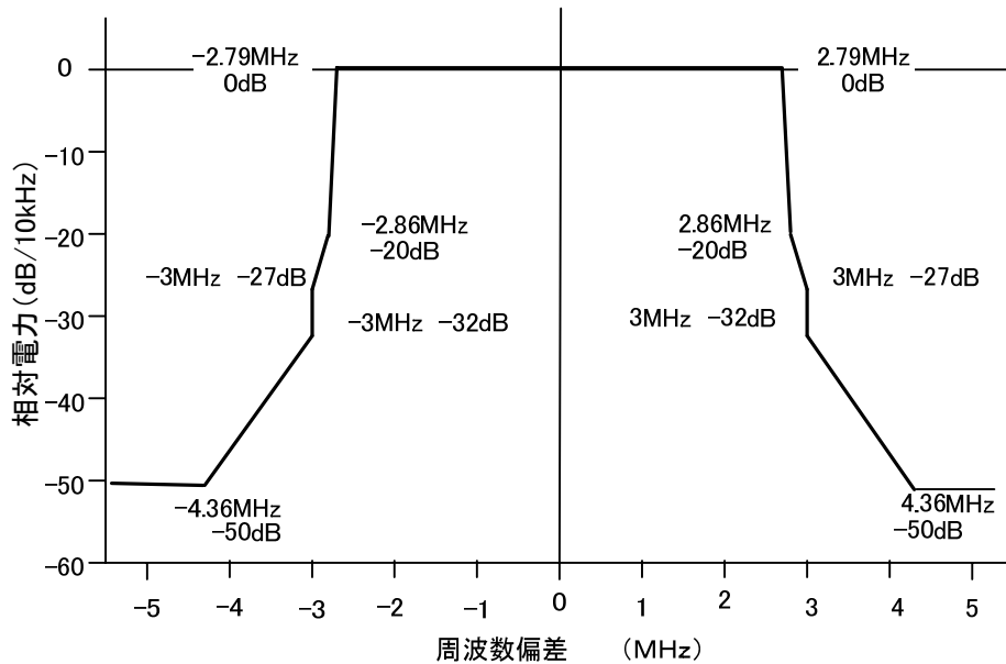
図5 受信IF出力電力スペクトル特性
