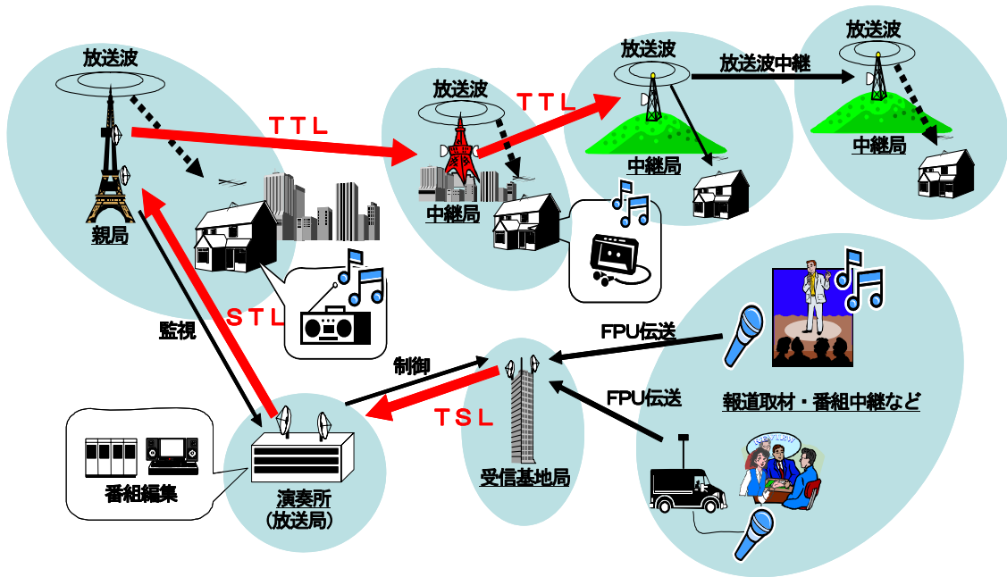
図1 音声STL/TTL/TSLの例
