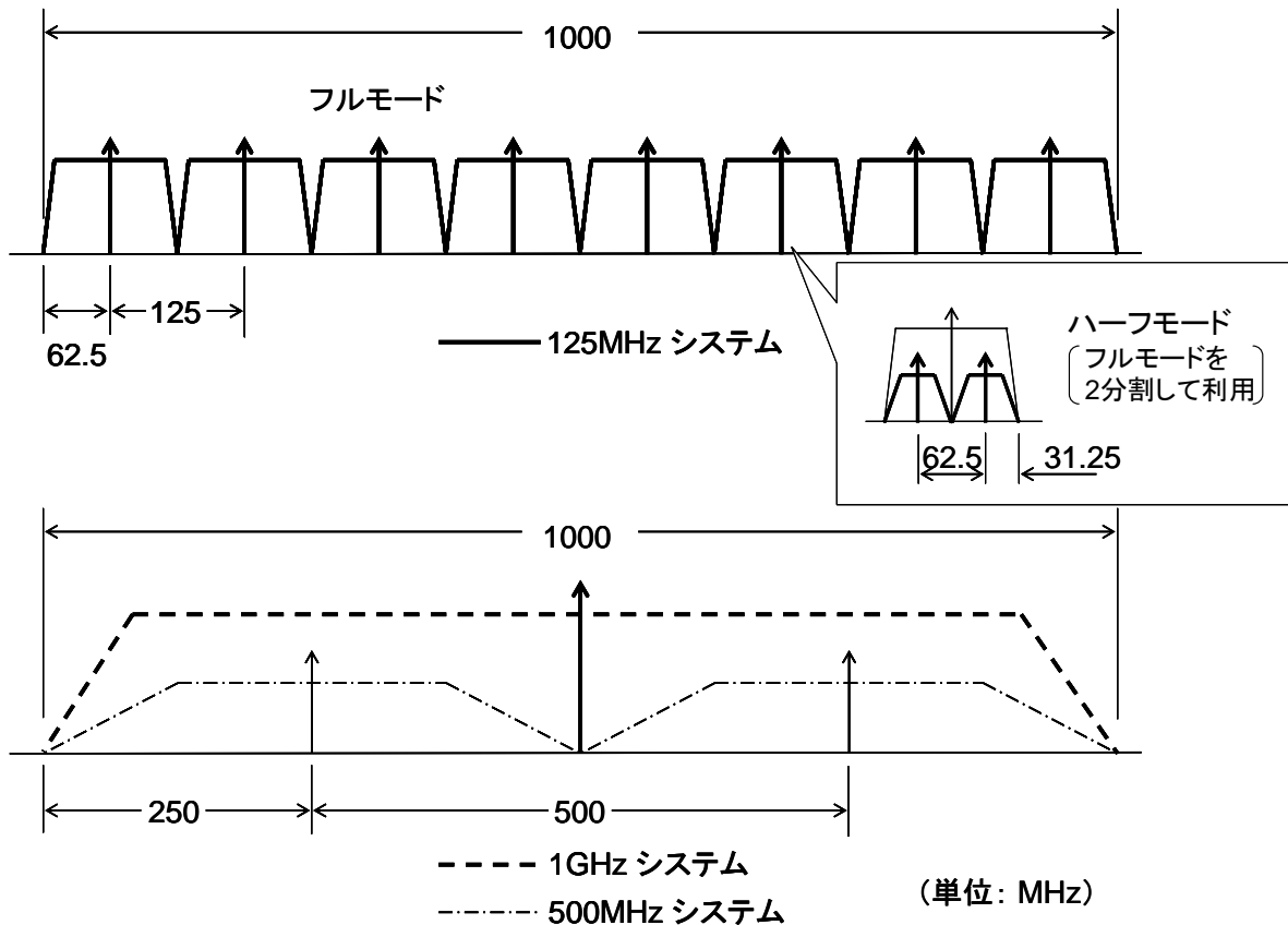
図3 42GHz帯/55GHz帯チャンネル配置
