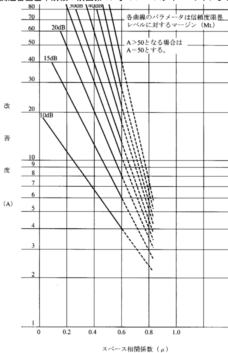
図1 スペースダイバーシティによる改善度
