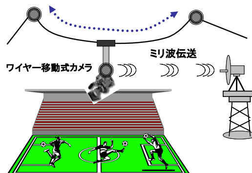
図2 移動式(ワイヤー移動式)カメラにおけるミリ波伝送の運用例
