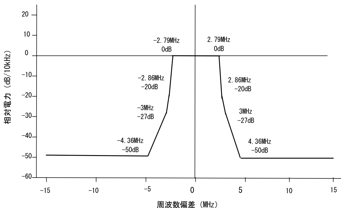
図2 送信電力スペクトル特性
