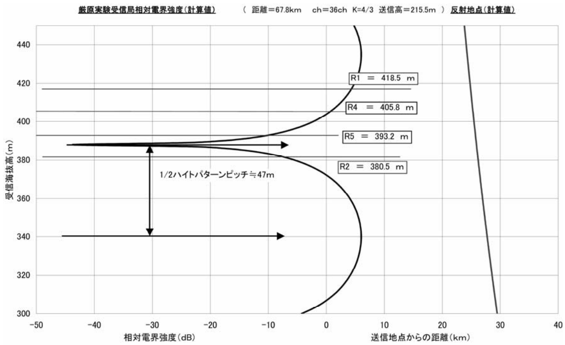
図2 郷ノ浦～巖原 受信ハイトパターン
