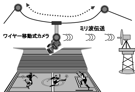
図 3-2 移動式(ワイヤー移動式)カメラにおけるミリ波伝送の運用例
