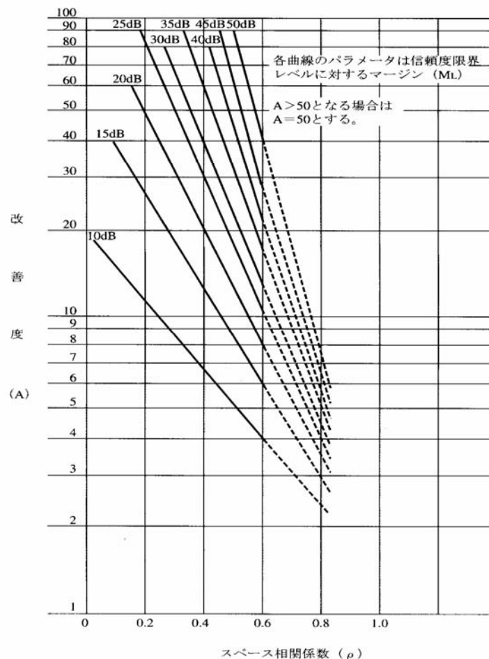
図 1 スペースダイバーシチによる改善度 (電波法関連審査基準別紙 1 別図第 46 号)
