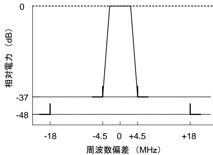
図 5 送信電力スペクトル特性
