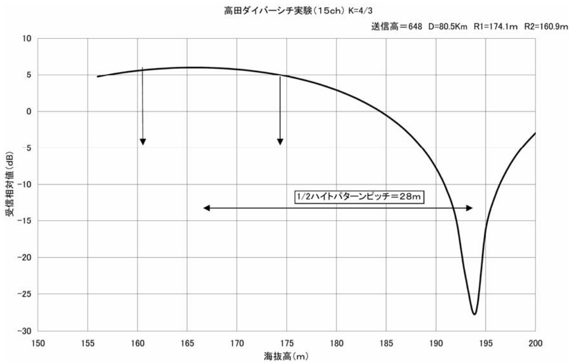
図3 弥彦～高田 受信ハイトパターン
