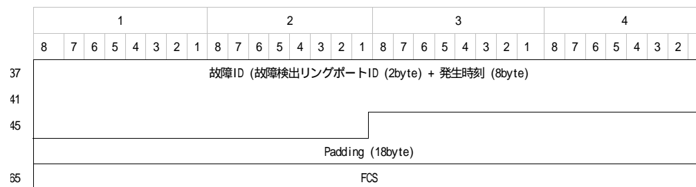
図 a-10 R-AIS フレーム構成
