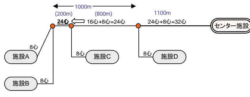
図7. 芯線数の考え方（ケース2）
