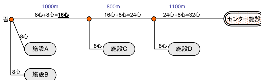
図6. 芯線数の考え方 (ケース1)
