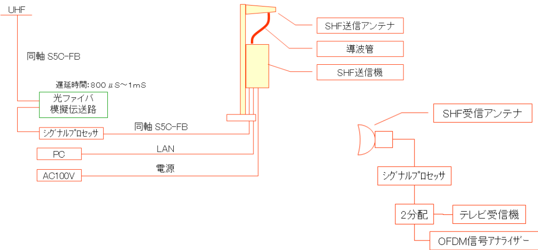
システム図
