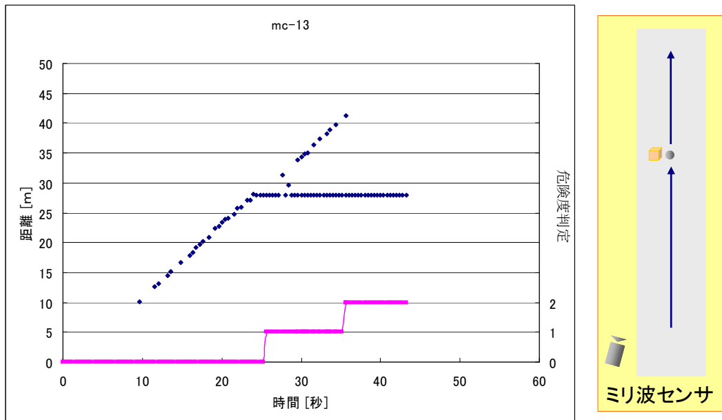
図 4-20 距離方向-投棄物残留 (人)
