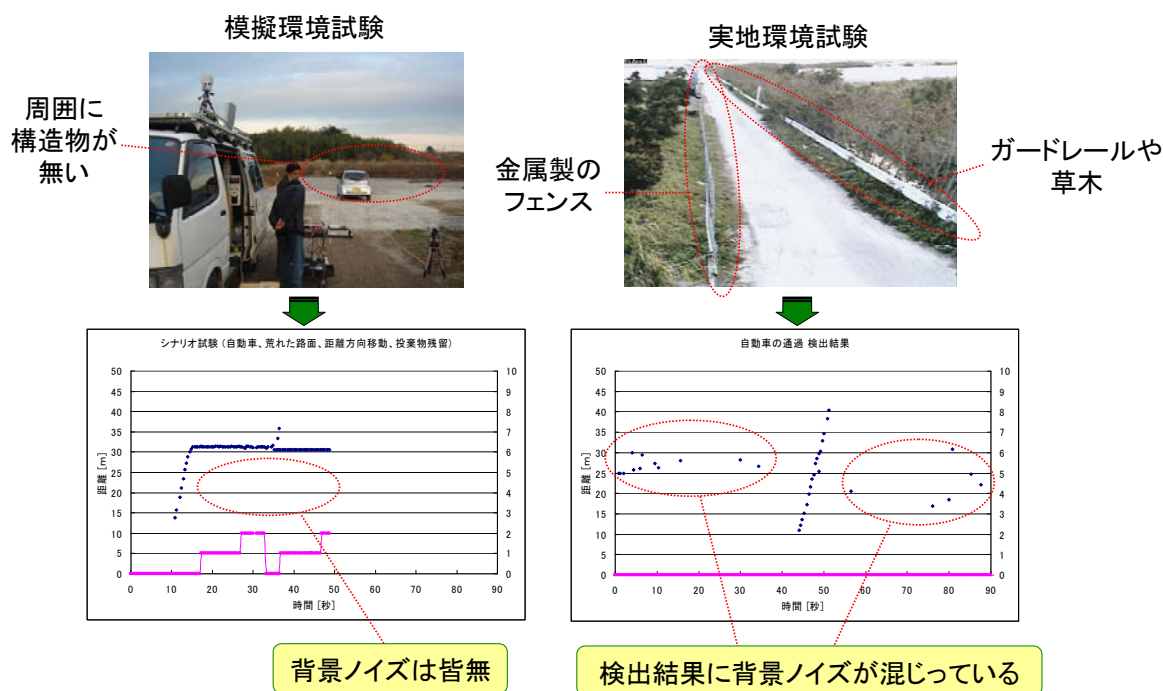
図 5-12 模擬環境試験と実地環境試験の差異
