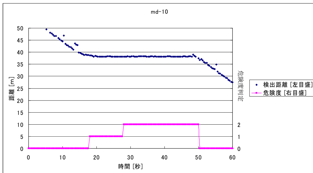
図 4-11 危険度 0→1→2 (自動車 遠→近) 40m 停止
