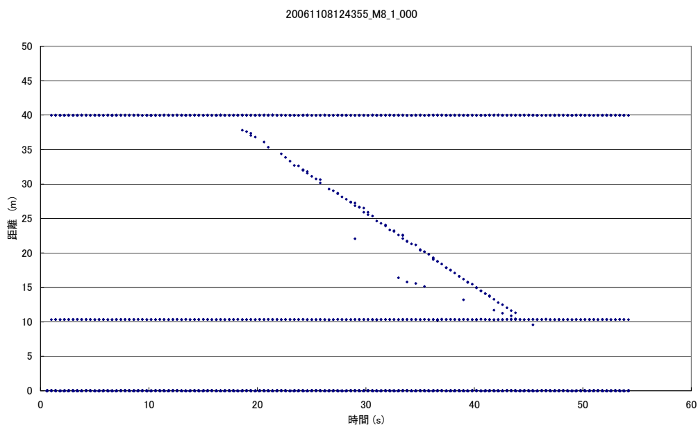
図 3-17 人の移動を検知した結果
