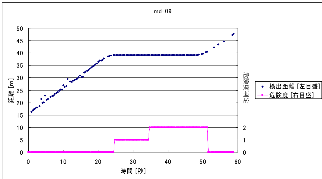
図 4-10 危険度 0→1→2 (自動車 近→遠) 40m 停止
