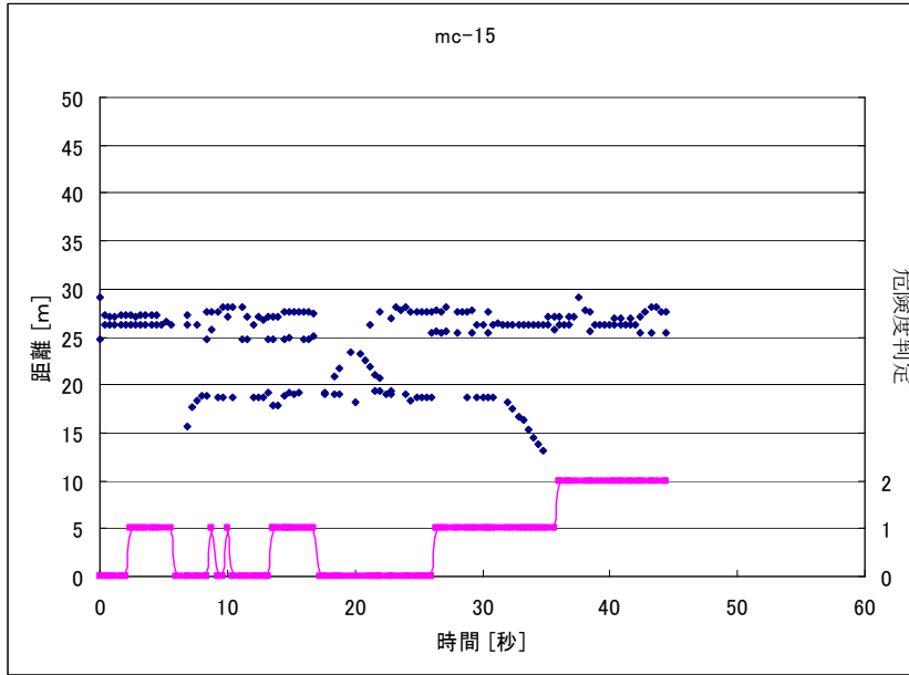
図 4-22 草地付近-投棄物残留 (自動車) 草地
