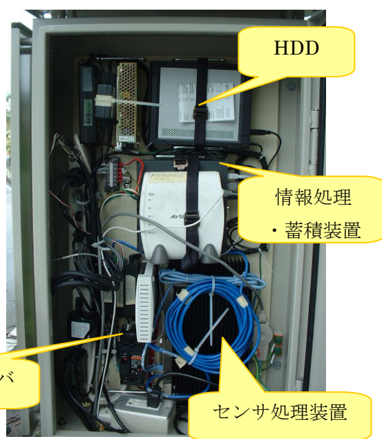
図 2-8 筐体内部写真
