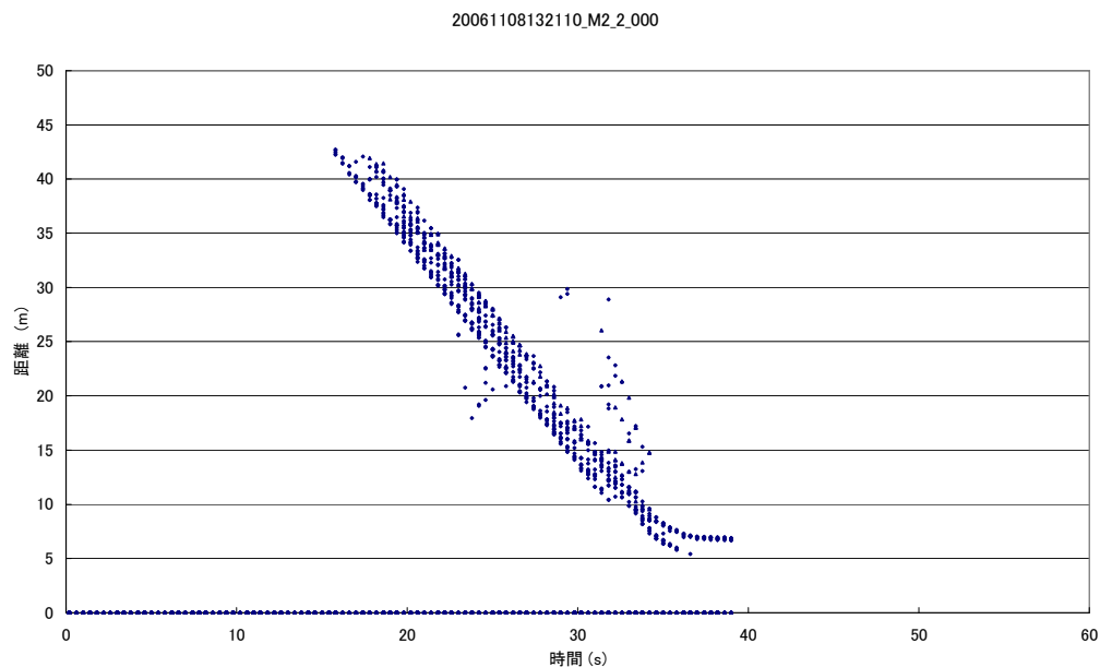
図 3-15 自動車の移動を検知した結果
