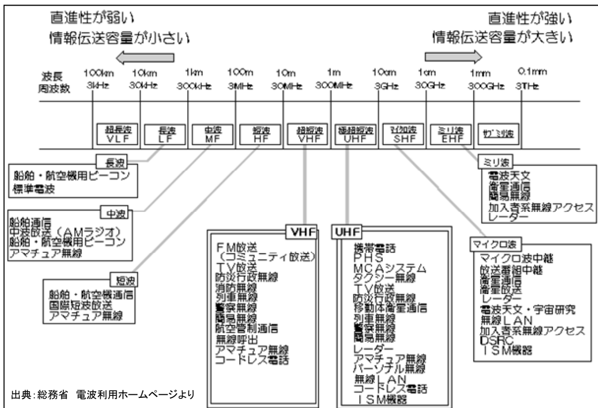
図 2-1 周波数 (波長) による電波の分類
