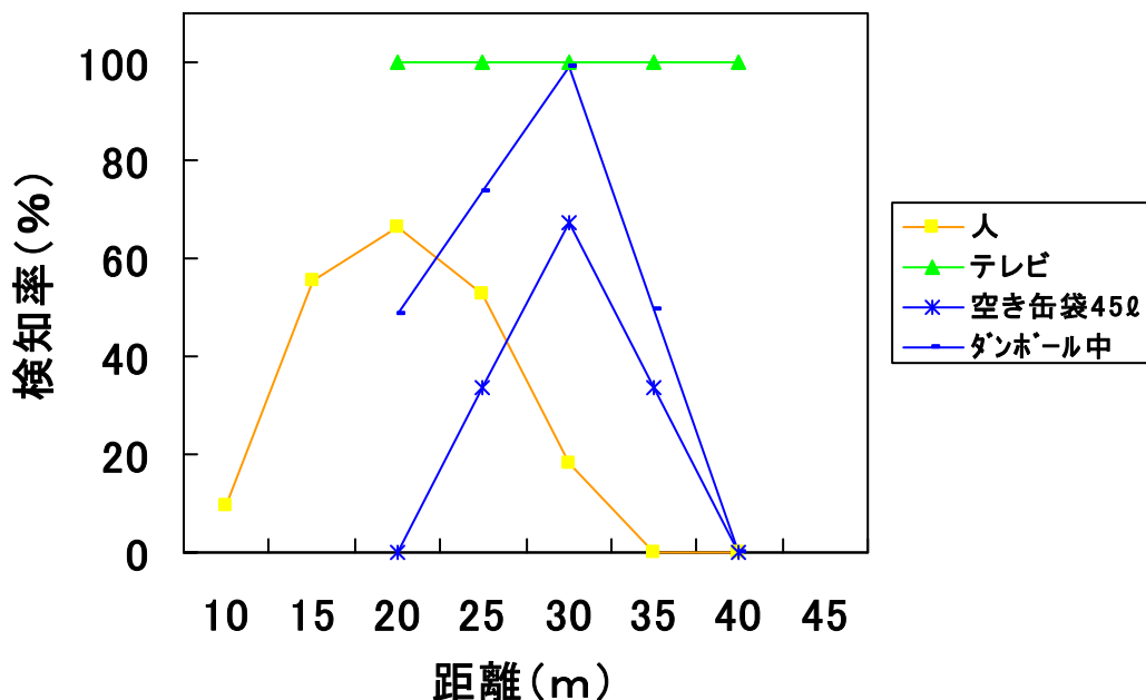
図 3-9 草地上での検知率
