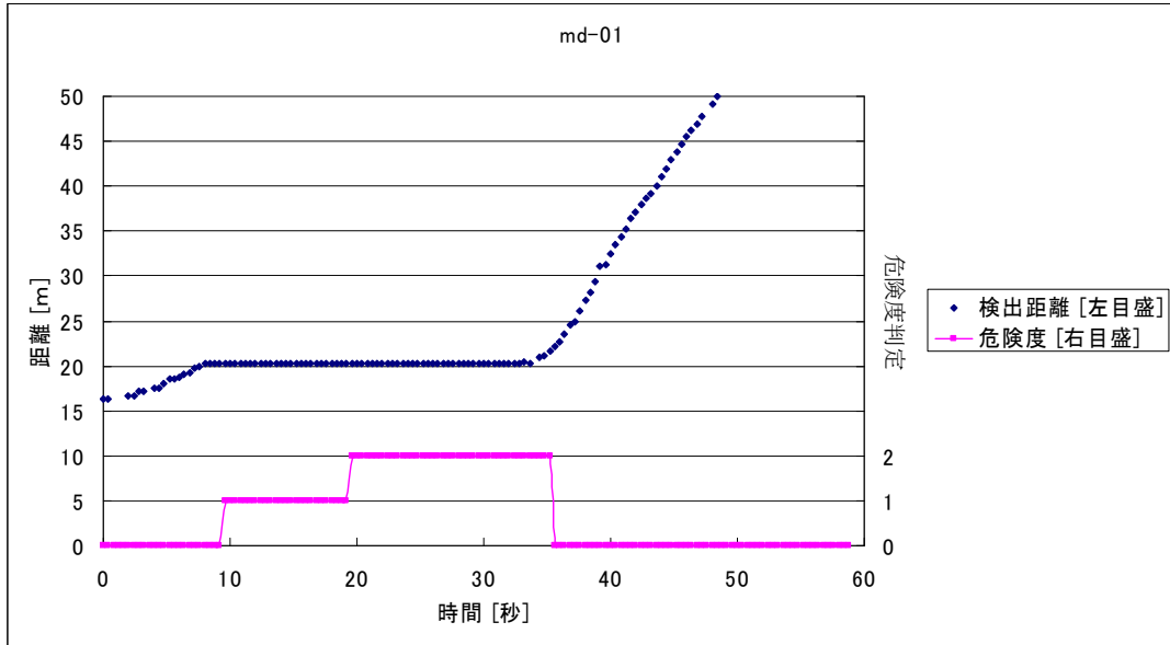
図 4-5 危険度 0→1→2 (自動車 近→遠) 20m 停止
