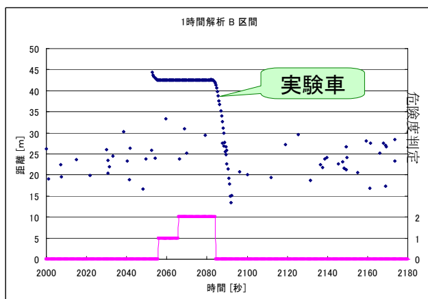
図 5-8 実験車両の判定結果
