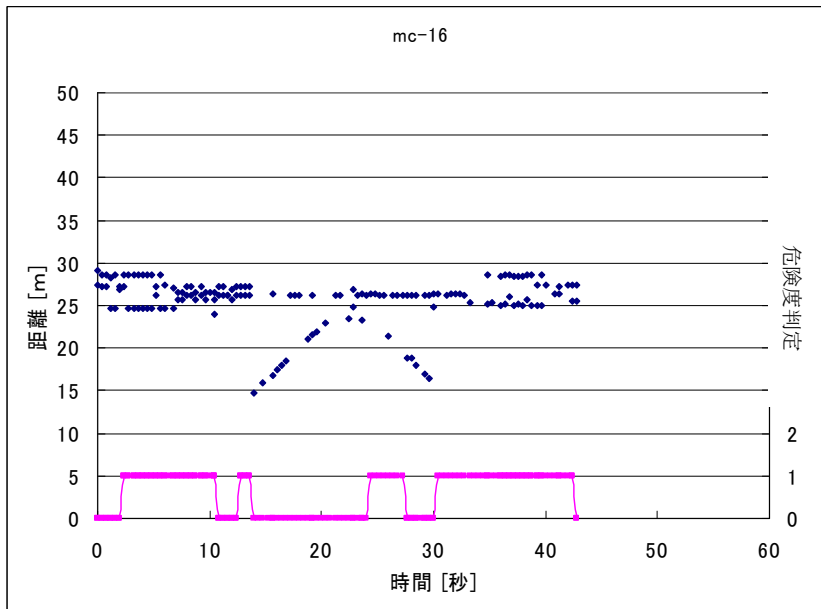
図 4-23 草地付近-投棄物残留 (人) 草地
