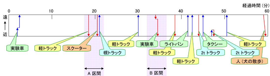
図 5-6 1時間分のデータ解析結果
