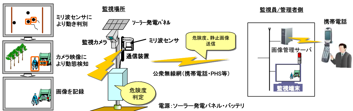
図 6-8 ミリ波センサを利用した不法投棄監視システムの例 (電源を用意できない場所)
