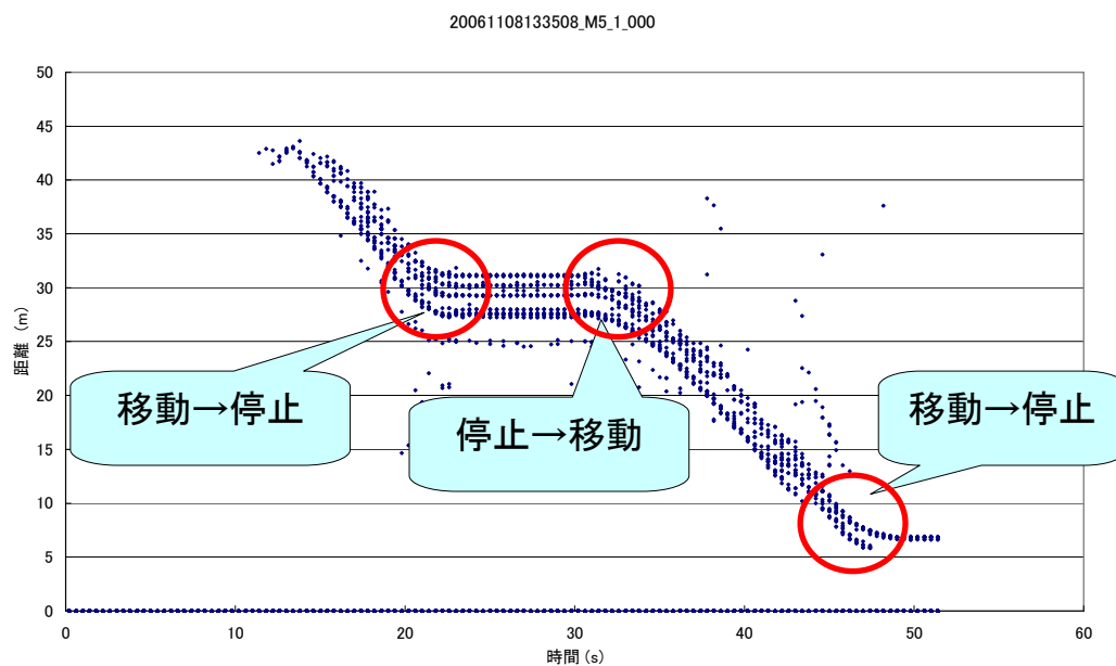
図 3-16 自動車の移動・停止を繰り返した結果
