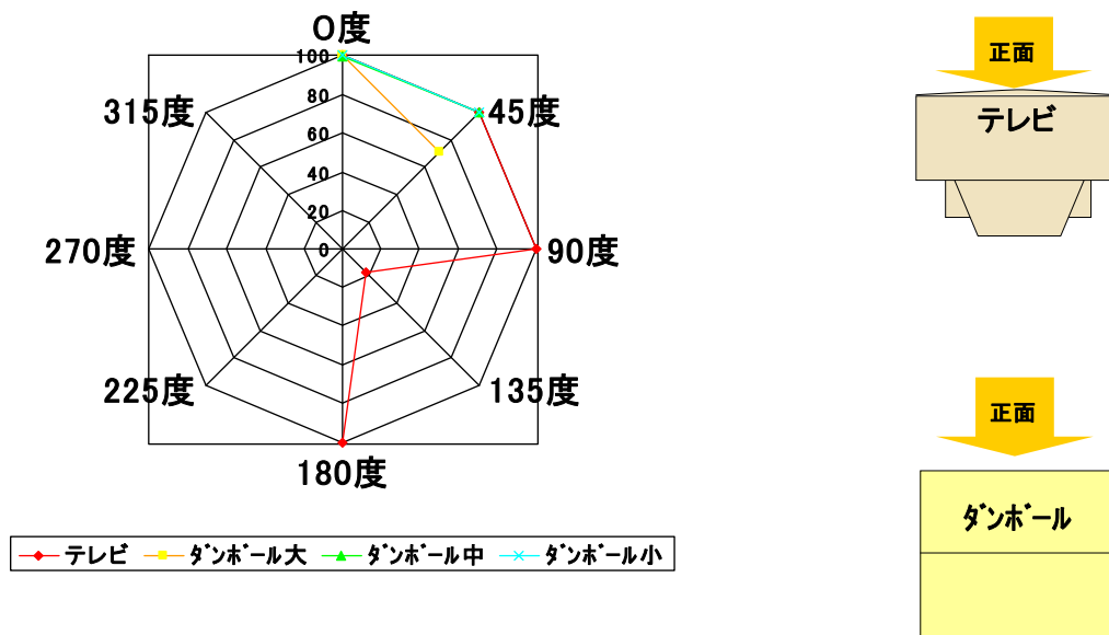
図 3-14 対象物回転時の検知率 (30m、アスファルト)
