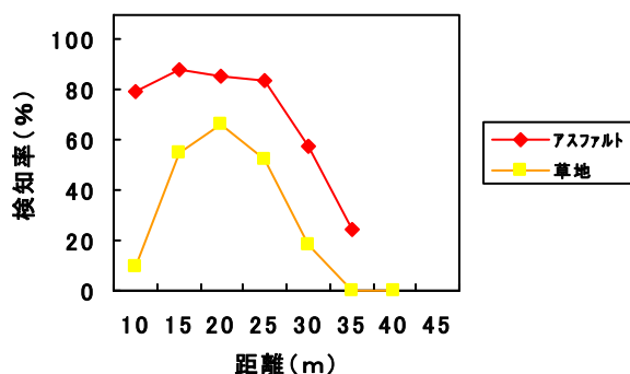
図 3-10 アスファルト・草地の比較 (人)
