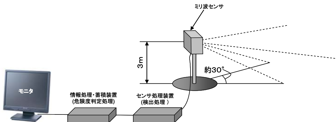
図 4-1 試験装置の構成
