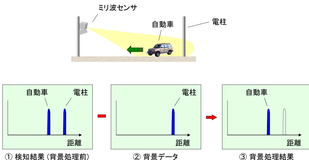
図 5-13 背景ノイズ
