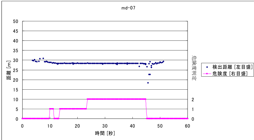
図 4-9 危険度 0→1→2 (自動車 横方向) 30m 停止
