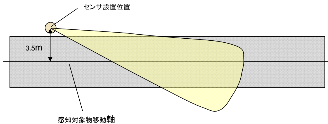
図 4-4 シナリオ試験時のセンサ配置
