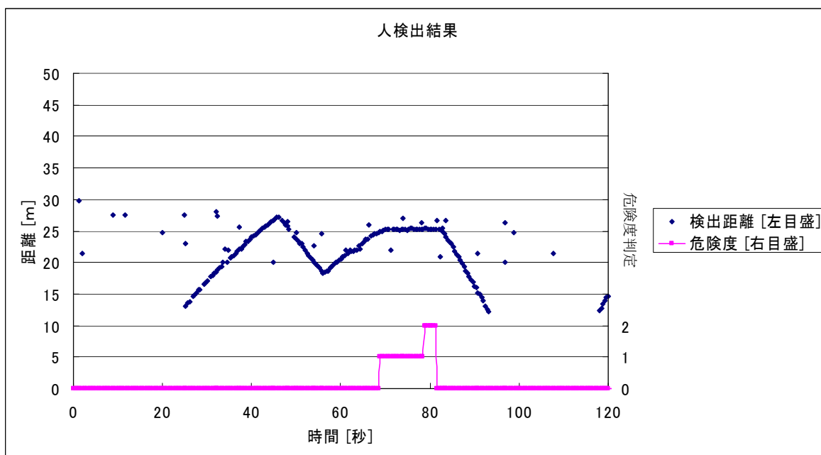
図 5-11 人の検知・判定結果
