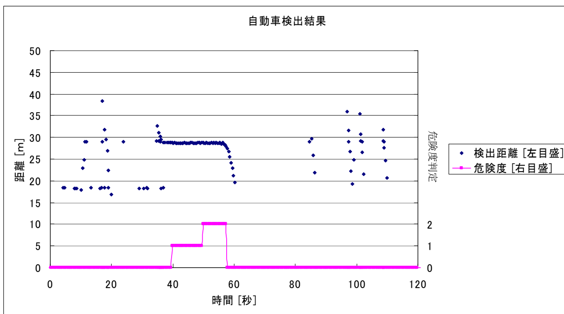
図 5-9 実験車両の検知・判定結果
