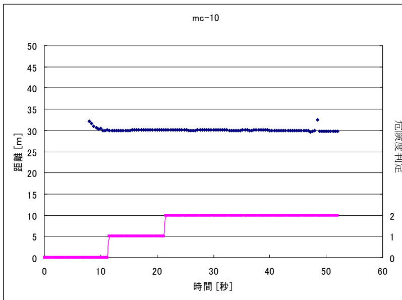
図 4-17 横方向停止 60 秒（自動車）荒れた路面
