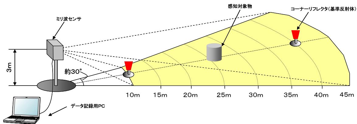
図 3-5 試験装置の構成イメージ
