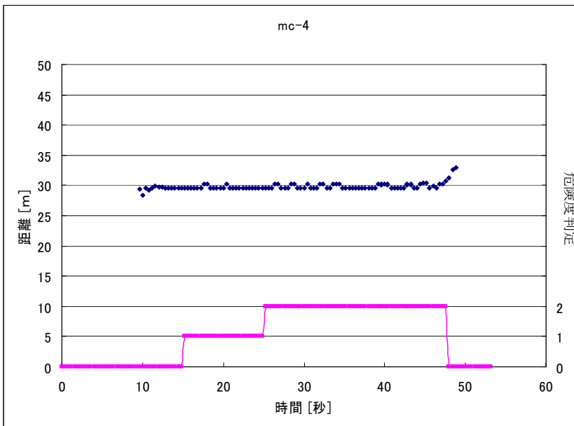
図 4-15 横方向停止 60 秒 (自動車)
