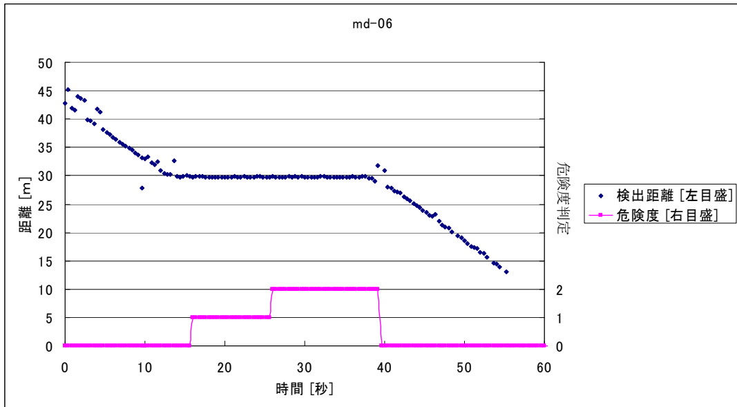
図 4-8 危険度 0→1→2 (自動車 遠→近) 30m 停止
