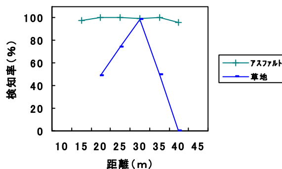
図 3-13 アスファルト・草地の比較 (ダンボール中)
