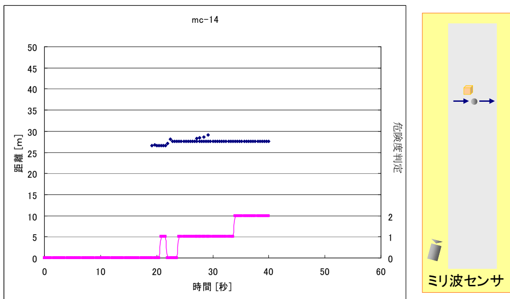
図 4-21 横方向-投棄物残留 (人)
