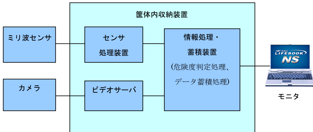
図 5-3 試験機器の構成
