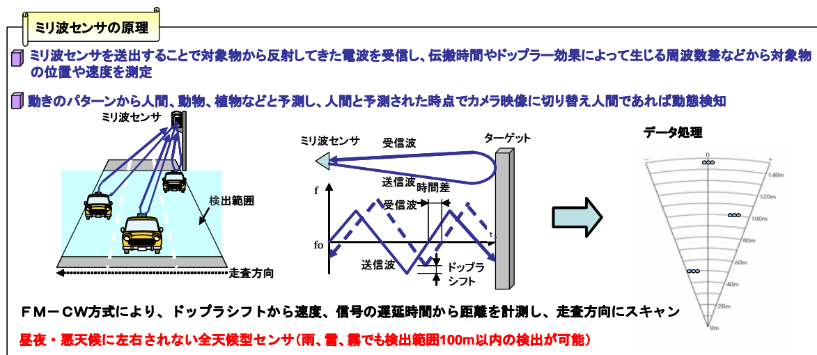
図 2-2 ミリ波センサの原理
