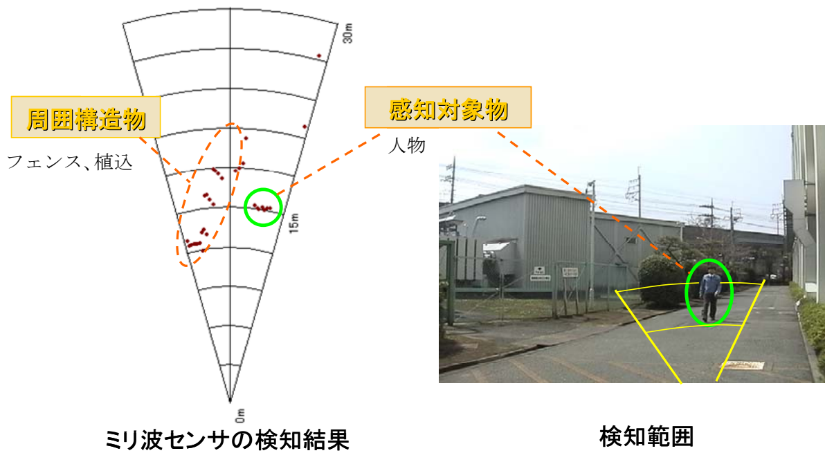
図 2-3 ミリ波センサの検知の例
