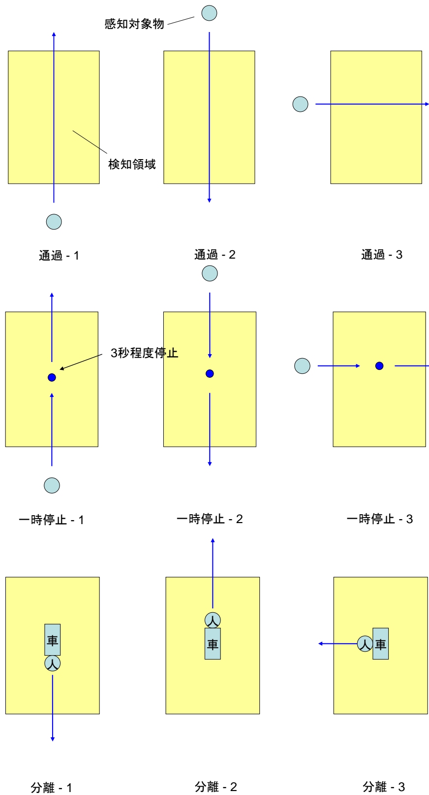
図 3-6 移動物検知試験における移動パターン
