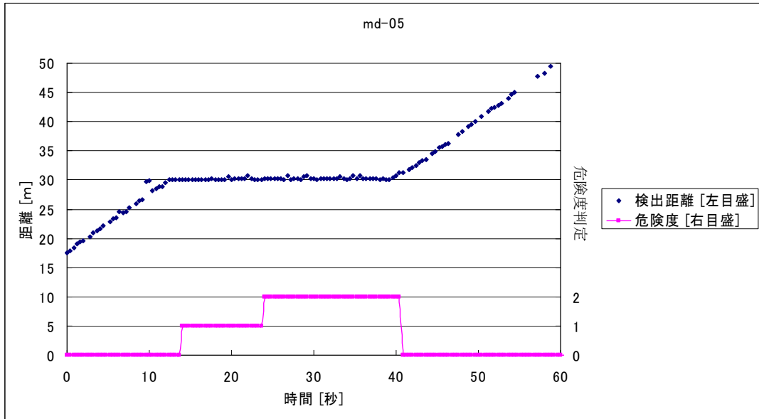
図 4-7 危険度 0→1→2 (自動車 近→遠) 30m 停止
