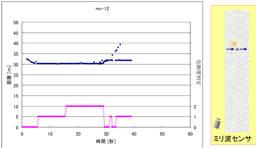
図 4-19 横方向停止 60 秒-投棄物残留 (自動車) 荒れた路面
