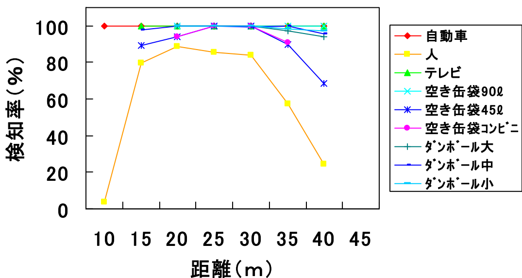
図 3-8 アスファルト上での検知率
