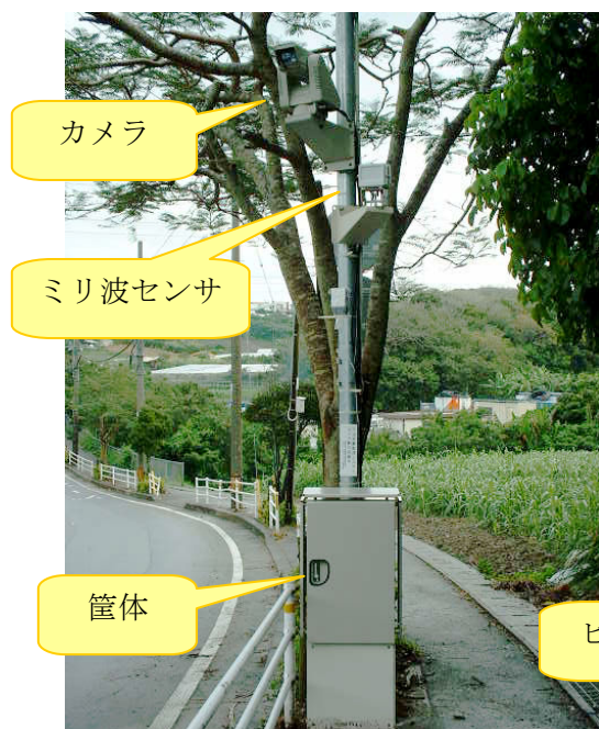
図 2-7 試作システム写真
