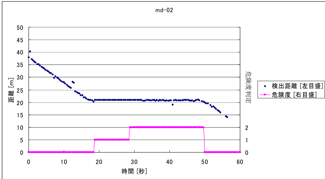
図 4-6 危険度 0→1→2 (自動車 遠→近) 20m 停止
