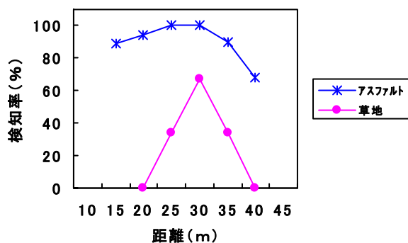
図 3-12 アスファルト・草地の比較 (空缶袋 450)
