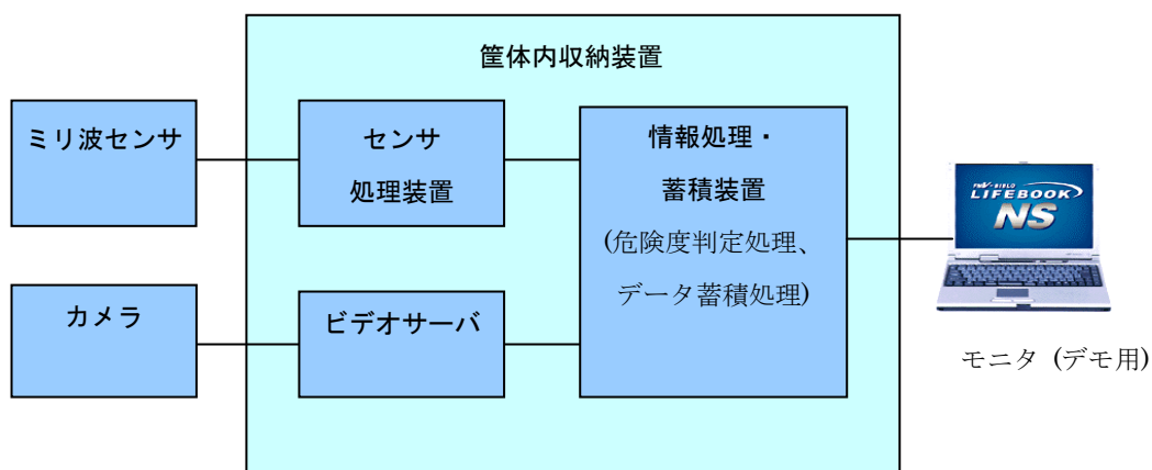
図 2-6 試作システムブロック図
