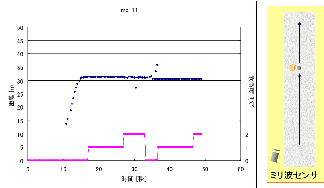
図 4-18 距離方向停止 60 秒-投棄物残留 (自動車) 荒れた路面
