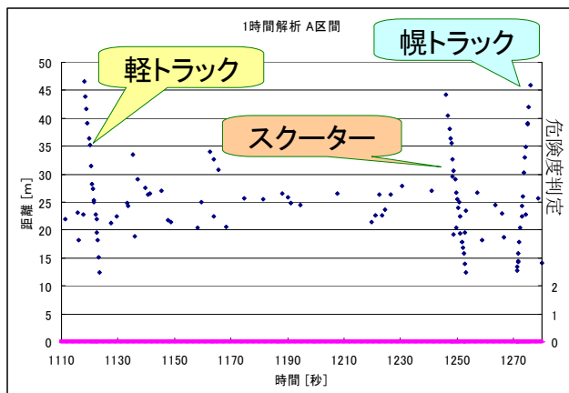
図 5-7 3つの対象物の通過の検知結果
