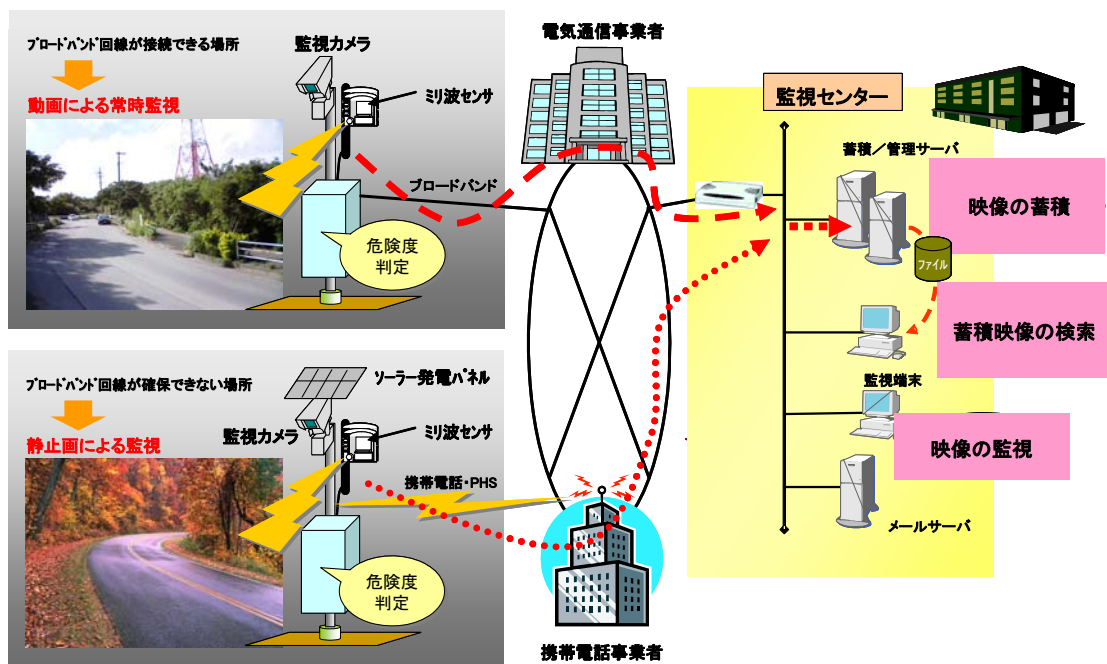
図 6-5 回線設定イメージ
