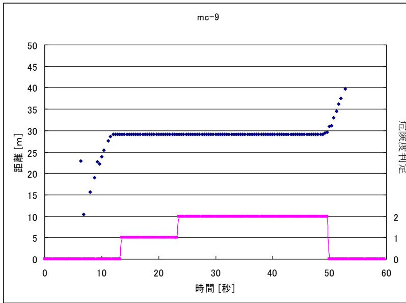
図 4-16 距離方向停止 60 秒（自動車）荒れた路面
