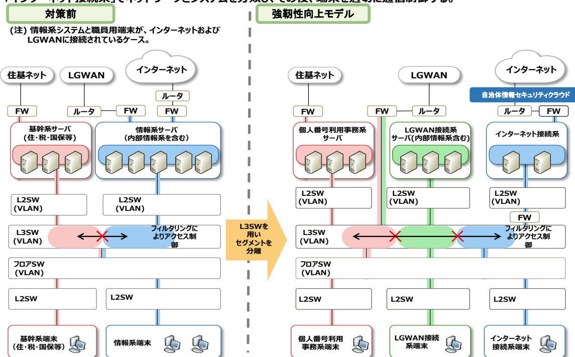
図表 22 強靱性向上モデルにおけるネットワーク再構成の一つのイメージ
