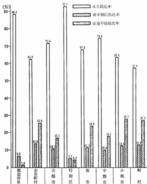
第49図 橋りょう整備の状況
