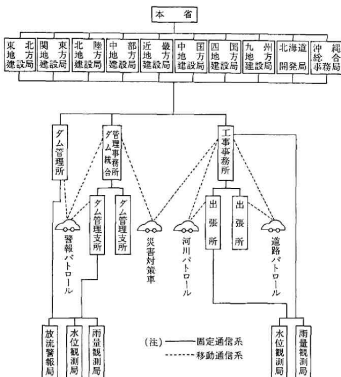
第2—3—17 図 水防道路用通信回線系統図
