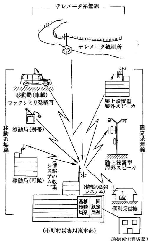
第2—3—21図 市町村防災行政用無線のシステム概念図
