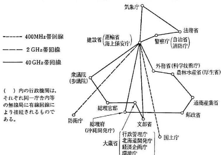
第 2—3—18 図 56年度末における中央防災無線網
