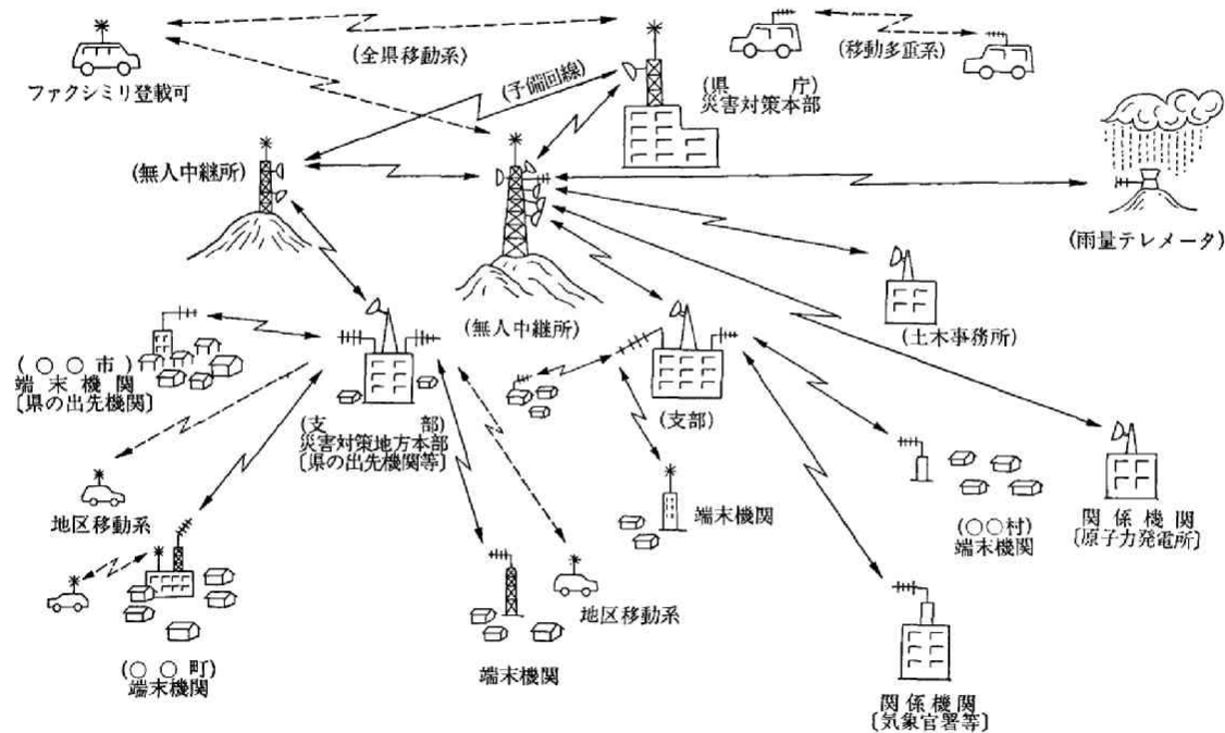
第 2-3-20 図 都道府県防災行政用無線のシステム概念図
