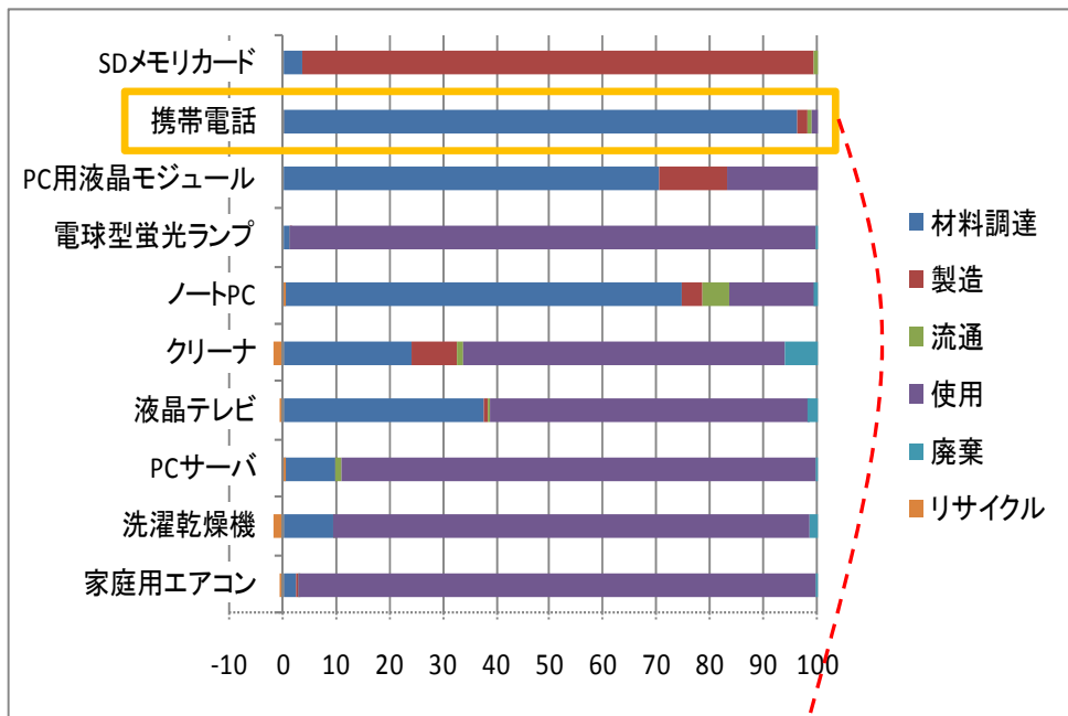
資料79-1 家電製品等のライフサイクルにおけるCO 2 排出割合
