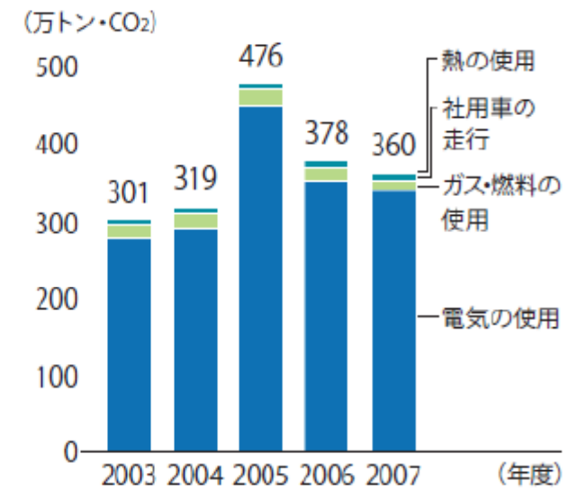
事業活動に伴うCO 2 排出量
