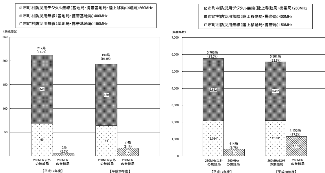
図表－４－５－８ 市町村防災用無線の整備状況【信越】
