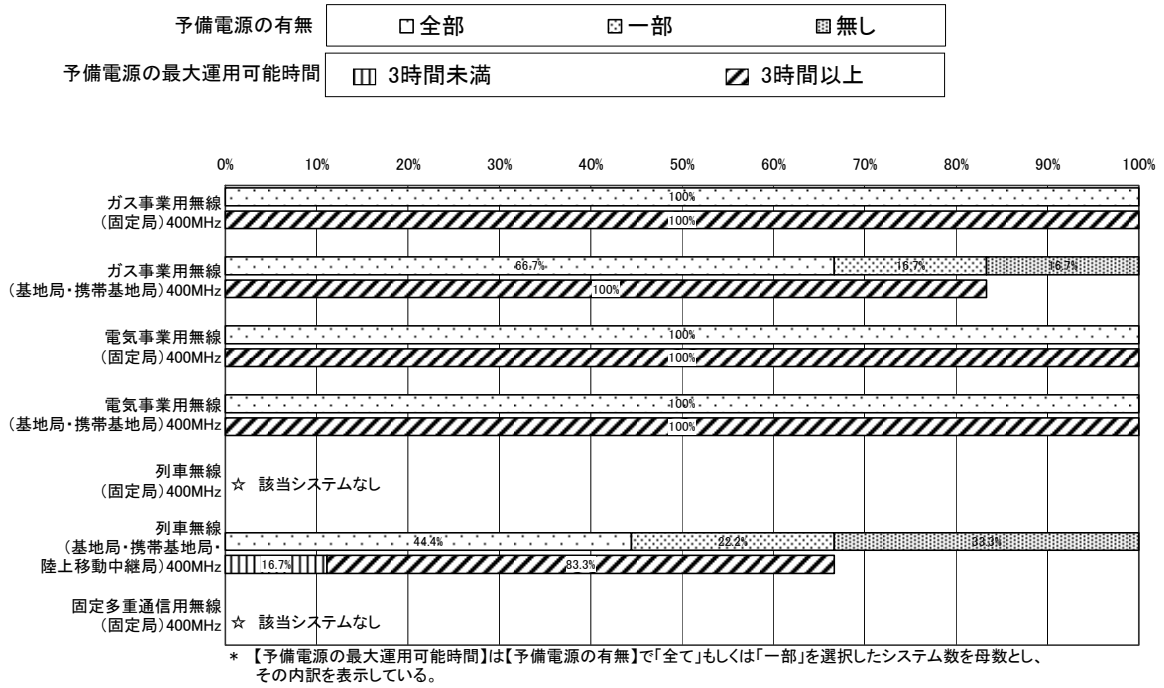
図表－４－６－１７ 予備電源保有状況及び予備電源の最大運用可能時間 (ガス事業用無線・電気事業用無線・列車無線・固定多重通信用無線) (内訳) 【信越】
