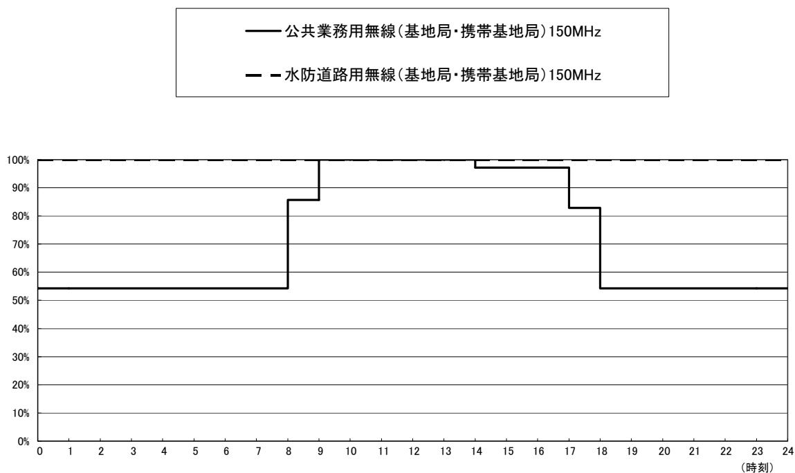
図表－４－４－９ 運用時間帯の分布（公共業務用無線・水防道路用無線 150MHz）【信越】
