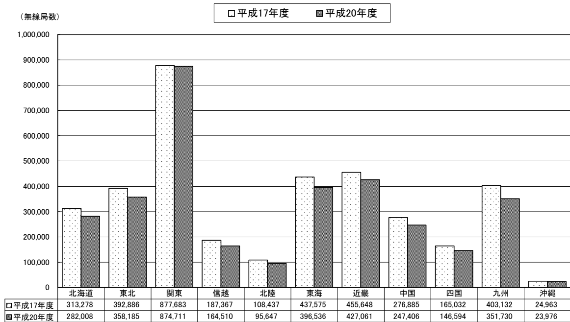
図表－４－１－３ 770MHz以下の無線局数の推移（各総合通信局の比較）
