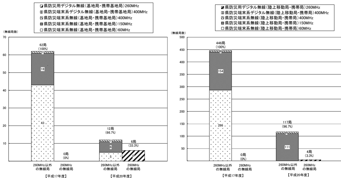
図表－４－５－７ 県防災用無線の整備状況【信越】
