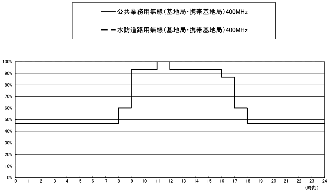
図表－４－６－８ 運用時間帯の分布（公共業務用無線・水防道路用無線 400MHz）【信越】
