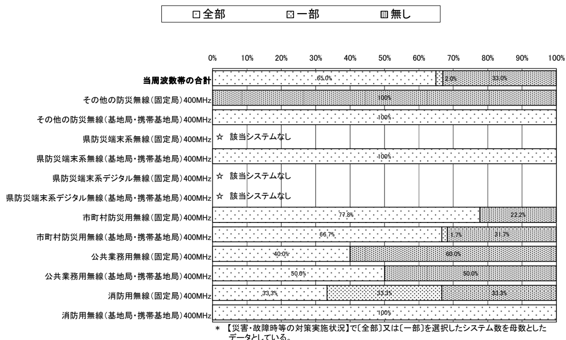
図表－４－６－１３ 復旧作業外部委託状況（内訳）【信越】
