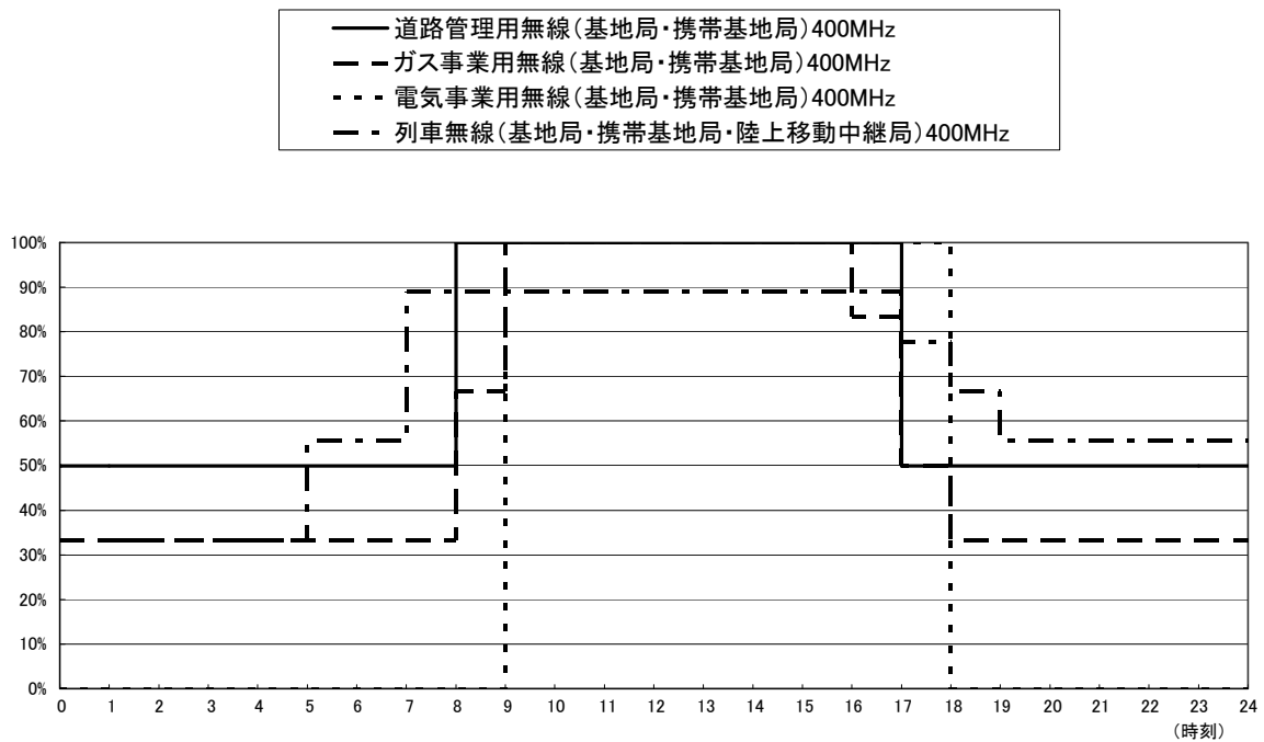
図表－４－６－９ 運用時間帯の分布 (道路管理用無線・ガス事業用無線・電気事業用無線・列車無線 400MHz)【信越】
