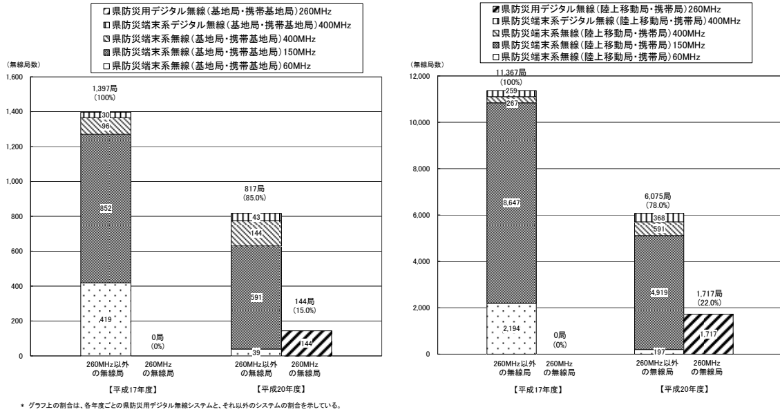
図表一全一五一六 県防災用無線局の整備状況【全国】
