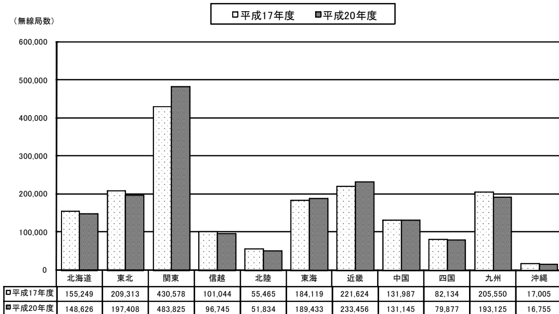
図表－全－1－5 770MHz 以下の無線局数の推移（各総合通信局の比較・アマチュア局を除く）
