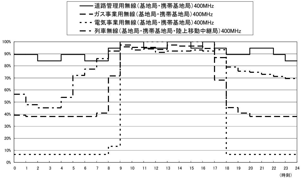
図表一全一6一7 運用時間帯の分布 (道路管理用無線・ガス事業用無線・電気事業用無線・列車無線 400MHz)【全国】
