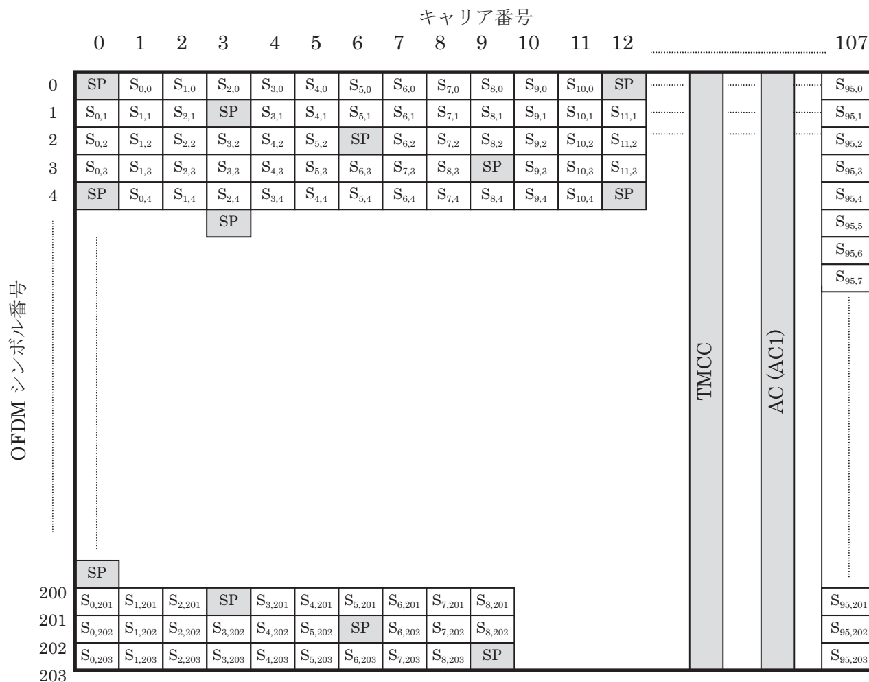
3.1.6.12-2 同期変調部の OFDM セグメント構成
