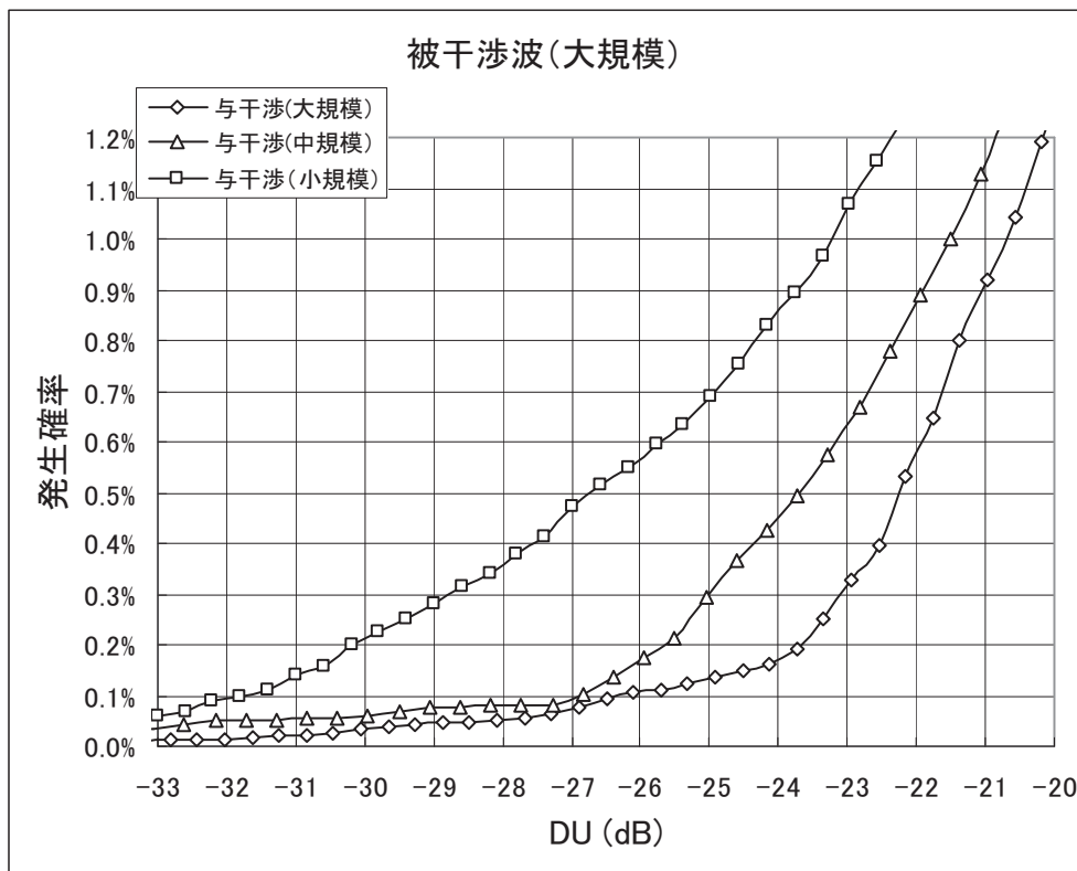
図 3.1.8.4-11 大規模局が被干渉局となる場合
