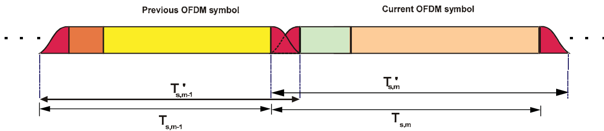
図 3.2.6.23.3-1. ウィンドウ処理された OFDM 信号の重ね合わせ
