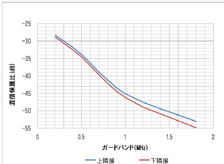
図 3.2.7.4.1.1-2 5%ESR 所要 DU ガードバンド (ISDB-Tmm to MediaFLO)
