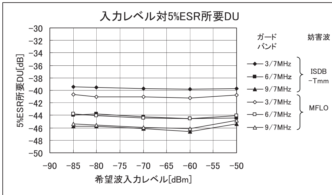
図 3.1.8.4-9 希望波入力レベル対 5%ESR 所要 DU (13 セグメント形式)
