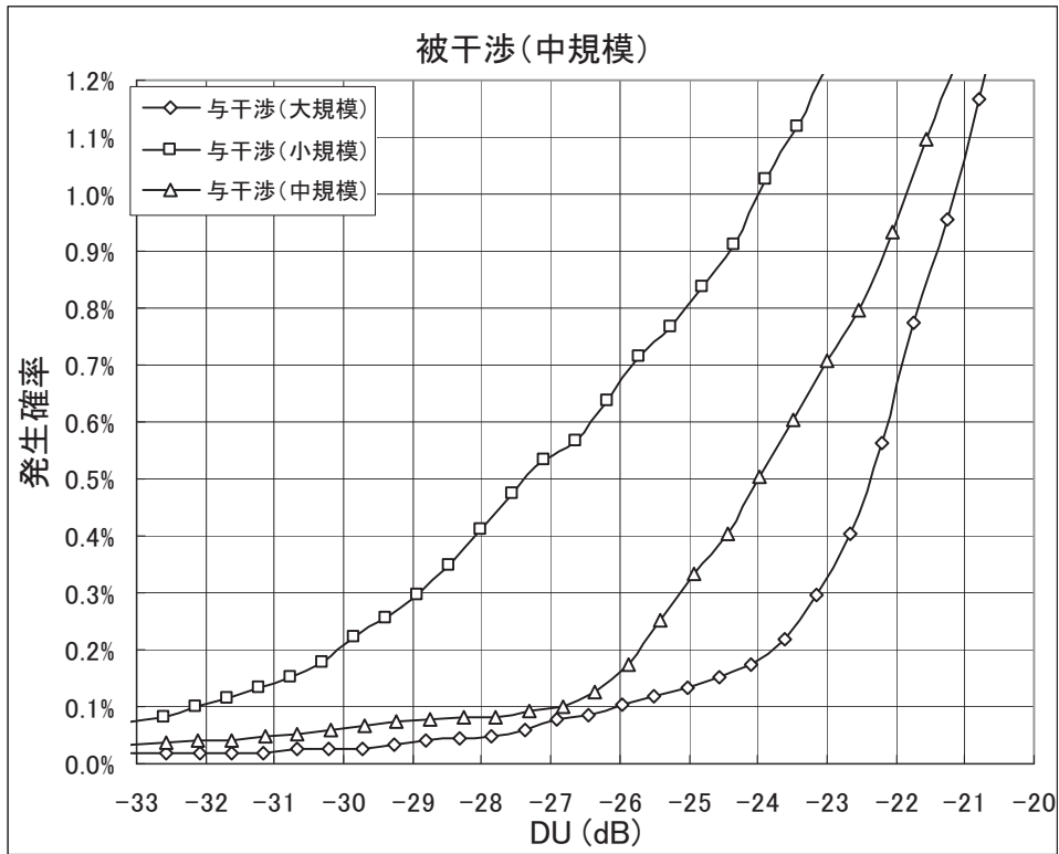
図 3.1.8.4-12 中規模局が被干渉局となる場合
