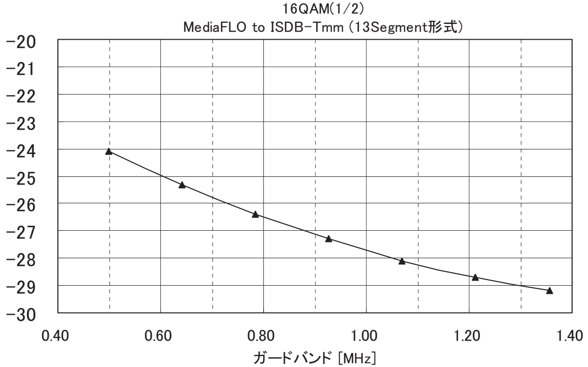
図 3.1.8.4-2 ガードバンド対混信保護比 (MediaFLO to ISDB-Tmm (13 セグメント形式))
