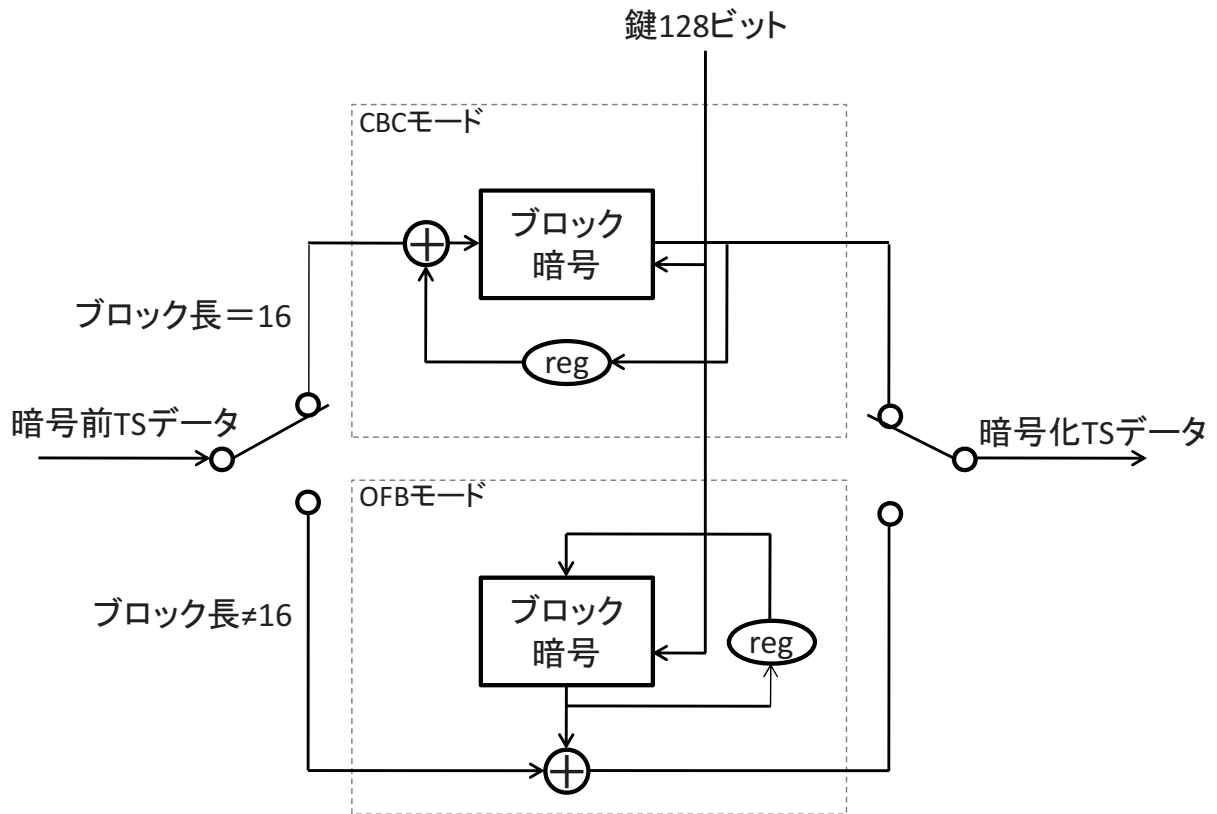
図 3.1.4.2-1 スクランブル方式は、128 ビットブロック暗号を適用した場合の例である。
