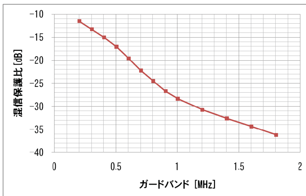
図 3.2.7.4.1-2 ガードバンド対混信保護比 (ISDB-Tmm to MediaFLO)
