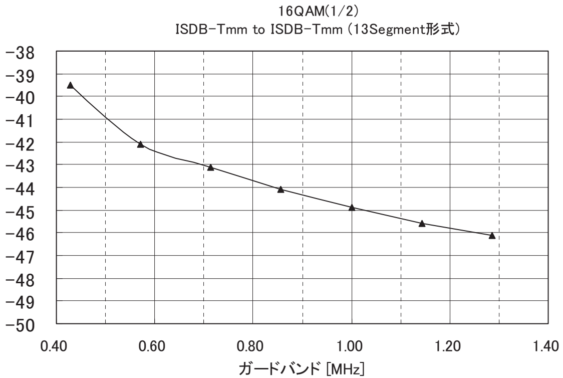
図 3.1.8.4-5 5%ESR 所要 DU 対ガードバンド (ISDB-Tmm to ISDB-Tmm (13 セグメント形式))
