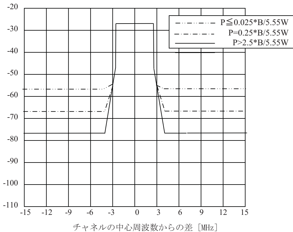
図 3.2.2.5-1 MediaFLO方式マルチメディア放送の送信スペクトルマスク (B=4.625、6.475もしくは7.4MHz)
