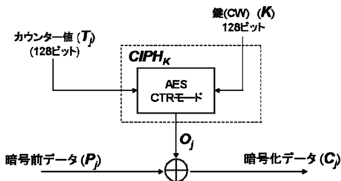
図 3.2.4.2-3 スクランブル方式の例
