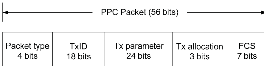
図3. 2. 6. 14. 2. 3. 2-1 PPCパケットフォーマット
