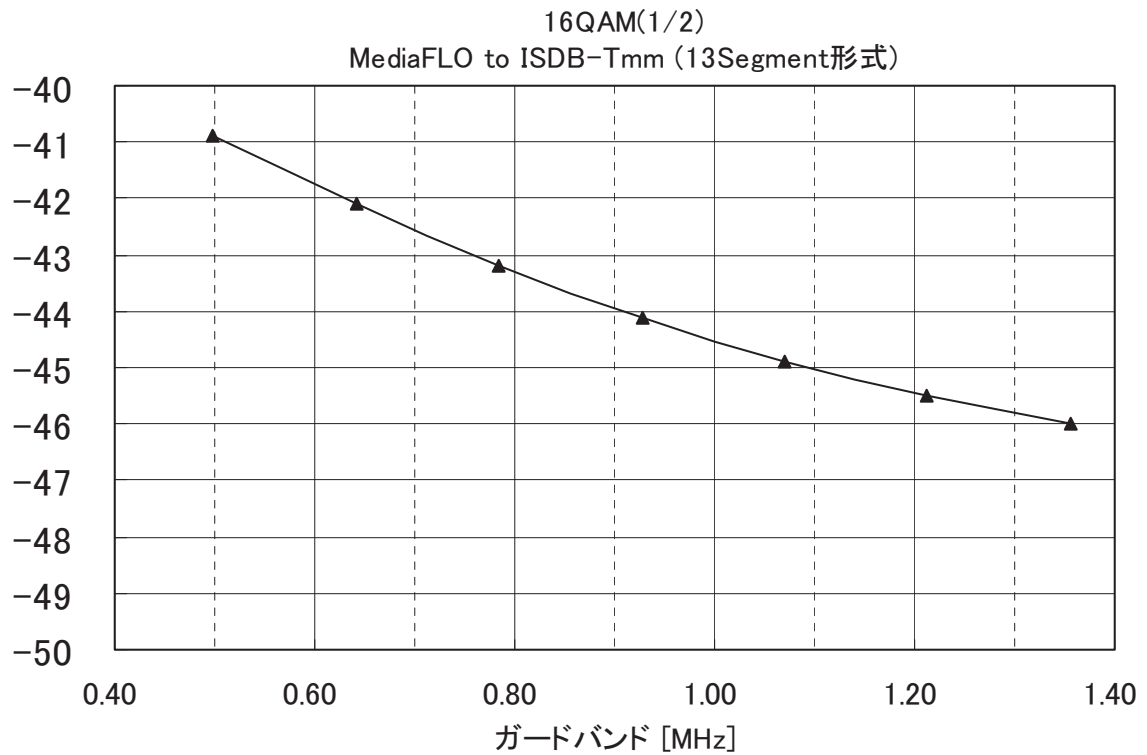
図 3.1.8.4-6 5%ESR 所要 DU 対ガードバンド (MediaFLO to ISDB-Tmm (13 セグメント形式))
