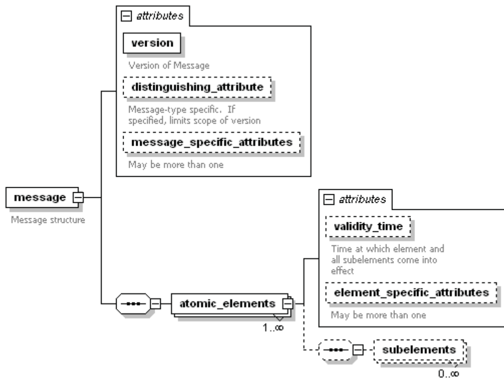
図 3.2.6.27-1. システム情報メッセージシNTAX
