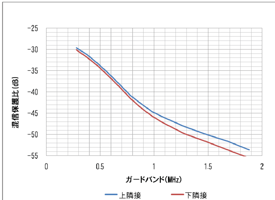
図 3.2.7.4.1.1-1 5%ESR 所要 DU 対ガードバンド (MediaFLO to MediaFLO)
