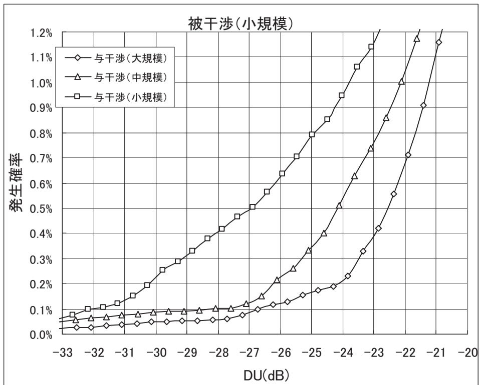
図 3.1.8.4-13 小規模局が被干渉局となる場合
