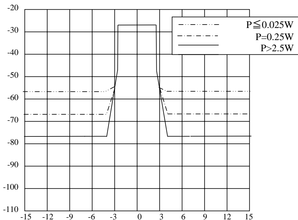
図 6-1: ISDB-Tmm方式マルチメディア放送の送信スペクトルマスク(n=13)
