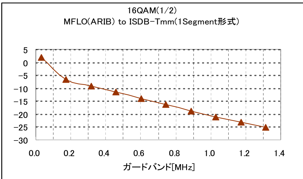
図5-5(a2) ガードバンド対混信保護比 (MFLO to ISDB-Tmm(1セグメント形式)) 16QAM((1/2))) (ガードバンド補正済)
