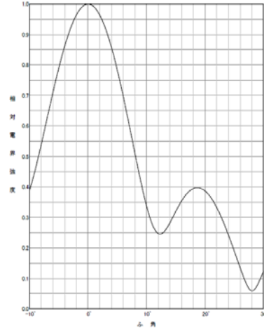
図5-11(b) 中規模局のアンテナパターン(2ダイポール4段4面)
