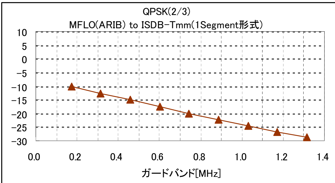
図5-5(b2) ガードバンド対混信保護比 (MFLO to ISDB-Tmm (1セグメント形式))
