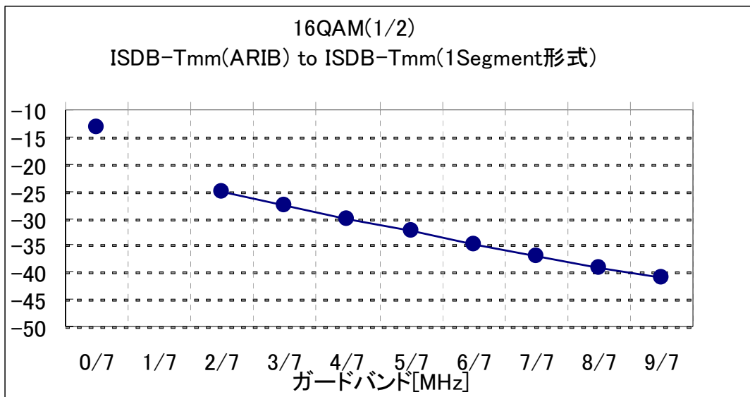
図5-8(a) 5%ESR所要DU対ガードバンド (ISDB-Tmm to ISDB-Tmm (1セグメント形式)) 16QAM (1/2)
