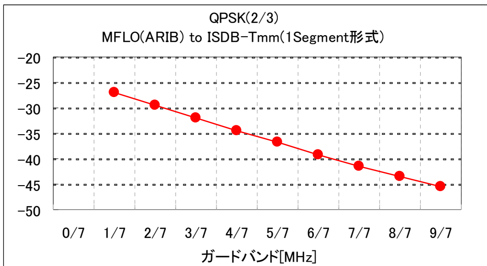
図5-9(b) 5%ESR所要DU対ガードバンド (MFLO to ISDB-Tmm (1セグメント形式)) QPSK (2/3)
