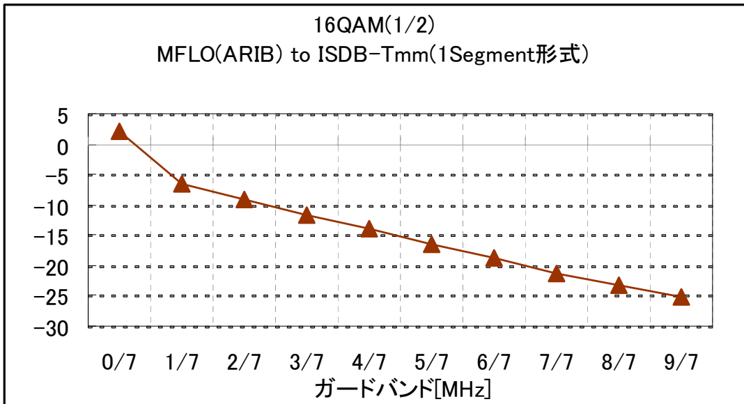
図5-5(a1) ガードバンド対混信保護比 (MFLO to ISDB-Tmm(1セグメント形式)) 16QAM((1/2))) (ガードバンド補正無)
