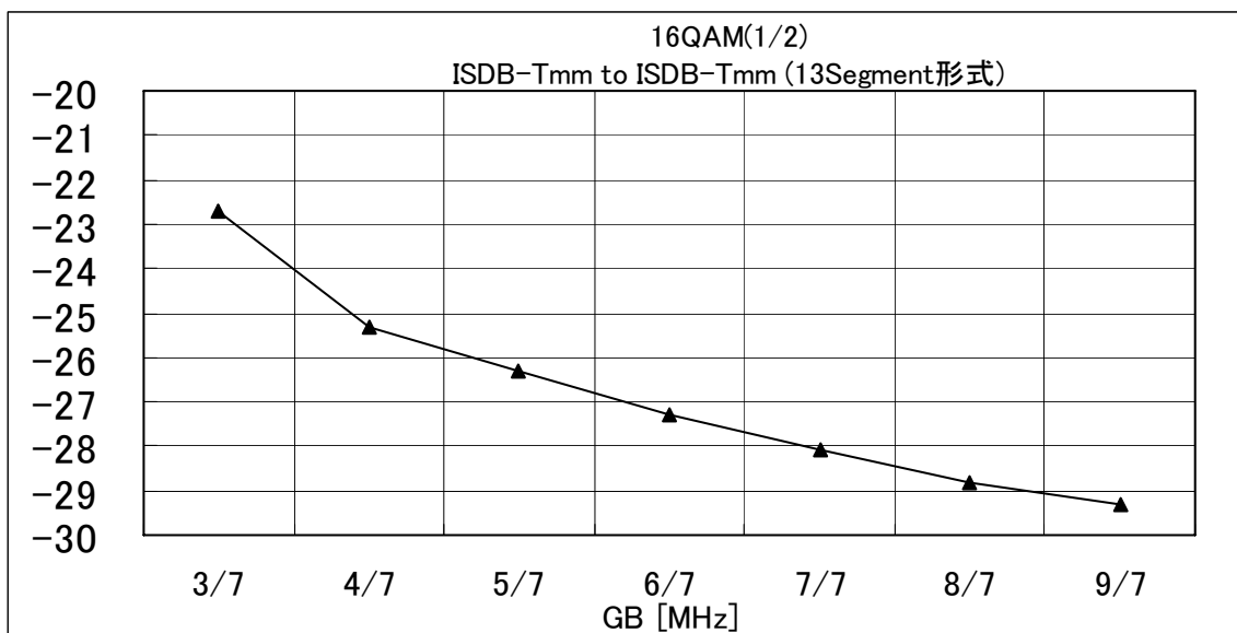
図5-1 ガードバンド対混信保護比 (ISDB-Tmm to ISDB-Tmm (13セグメント形式))
