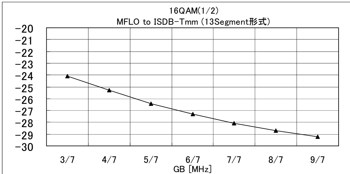
図5-2-1 ガードバンド対混信保護比 (MFLO to ISDB-Tmm (13セグメント形式)) (ガードバンド補正無)
