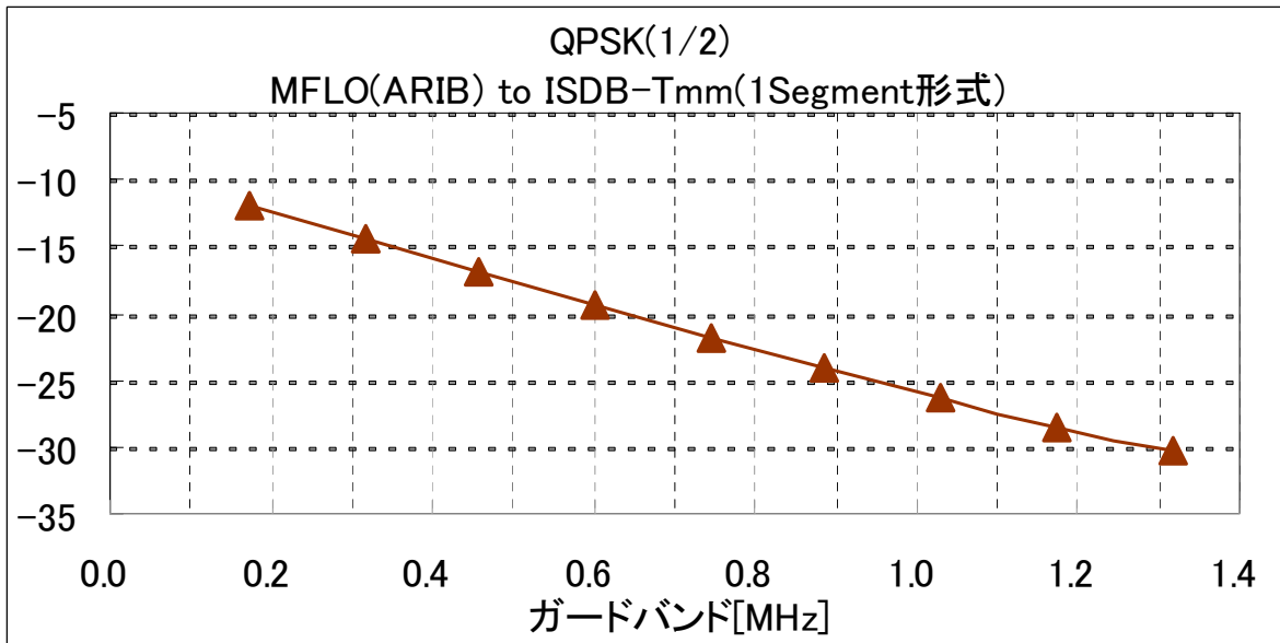
図5-5(c2) ガードバンド対混信保護比 (MFLO to ISDB-Tmm (1セグメント形式)) QPSK (1/2) (ガードバンド補正済)
