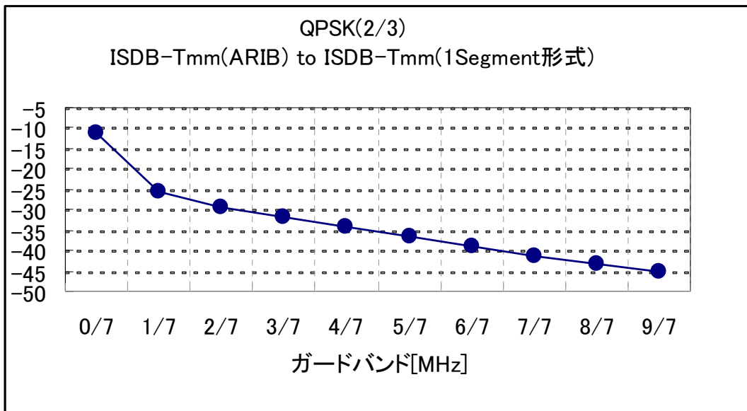
図5-8(b) 5%ESR所要DU対ガードバンド (ISDB-Tmm to ISDB-Tmm (1セグメント形式)) QPSK (2/3)
