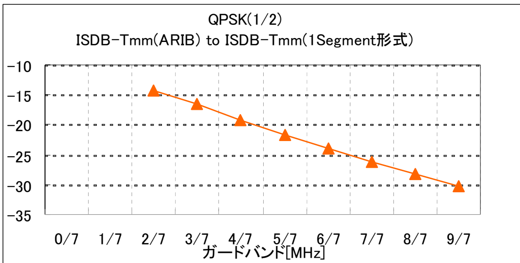
図5-4(c) ガードバンド対混信保護比 (ISDB-Tmm to ISDB-Tmm (1セグメント形式)) QPSK (1/2)
