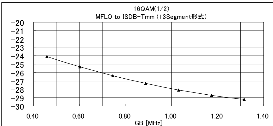
図5-2-2 ガードバンド対混信保護比 (MFLO to ISDB-Tmm (13セグメント形式)) (ガードバンド補正済)
