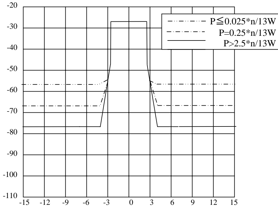
図 6-2 ISDB-Tmm方式マルチメディア放送の送信スペクトルマスク( n \geq 13 )
