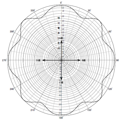
図5-11(b) 中規模局のアンテナパターン(2ダイポール4段4面)
