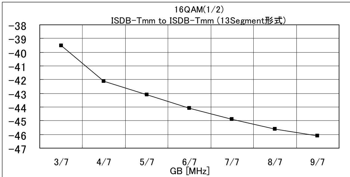
図5-6 5%ESR所要DU対ガードバンド (ISDB-Tmm to ISDB-Tmm (13セグメント形式))
