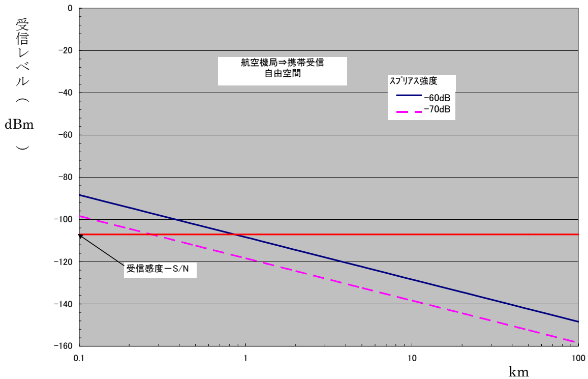
3 航空機局 携帯端末 の受信 の 干渉ルート 2
