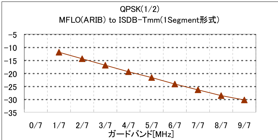
図5-5(c1) ガードバンド対混信保護比 (MFLO to ISDB-Tmm (1セグメント形式)) QPSK (1/2) (ガードバンド補正無)
