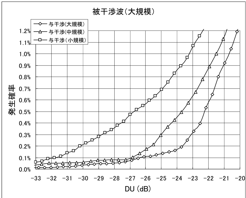
図5-12: 大規模局が被干渉局となる場合
