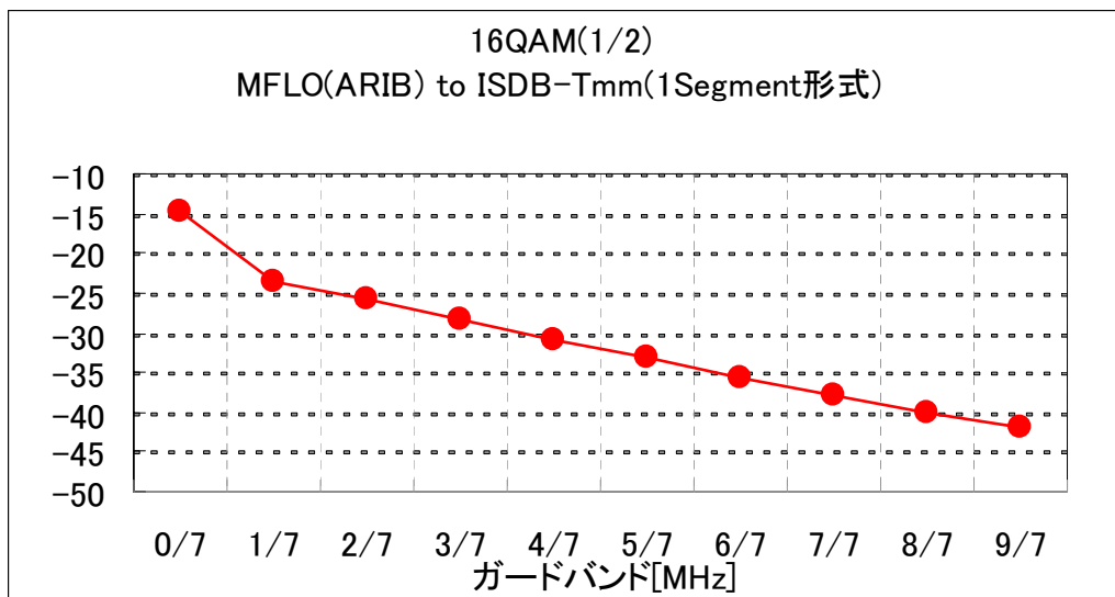
図5-9(a) 5%ESR所要DU対ガードバンド (MFLO to ISDB-Tmm (1セグメント形式)) 16QAM (1/2)
