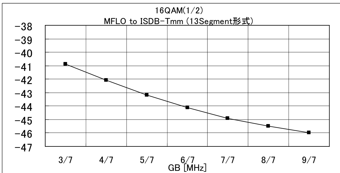
図5-7 5%ESR所要DU対ガードバンド (MFLO to ISDB-Tmm (13セグメント形式))
