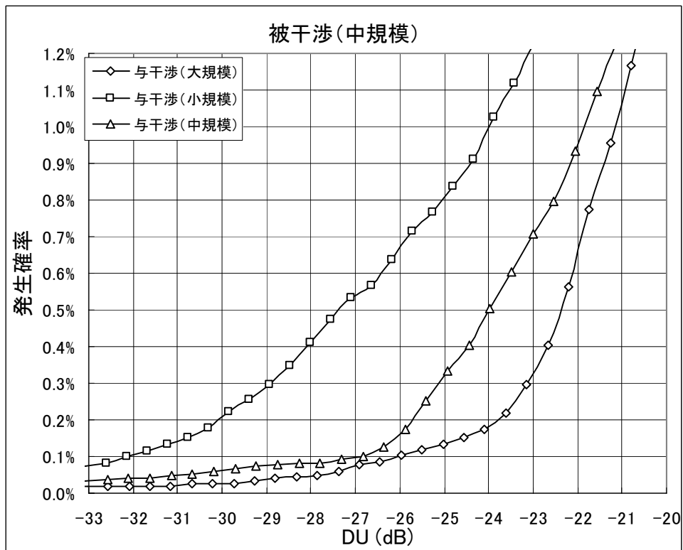
図5-13: 中規模局が被干渉局となる場合
