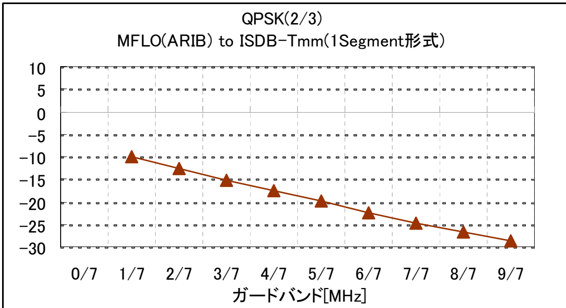
図5-5(b1) ガードバンド対混信保護比 (MFLO to ISDB-Tmm (1セグメント形式))
