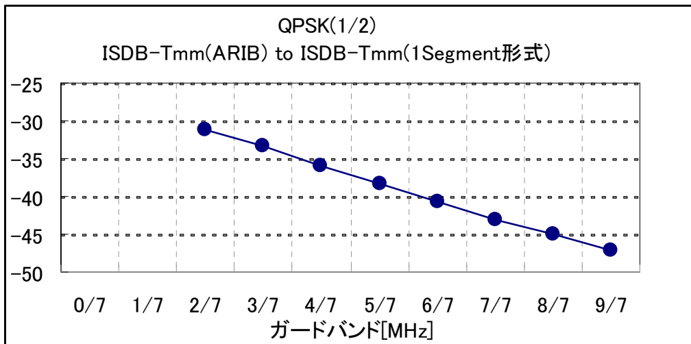
図5-8(c) 5%ESR所要DU対ガードバンド (ISDB-Tmm to ISDB-Tmm (1セグメント形式)) QPSK (1/2)
