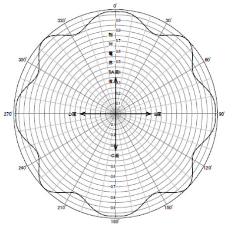
図5-11(a) 大規模局のアンテナパターン(2ダイポール8段4面)
