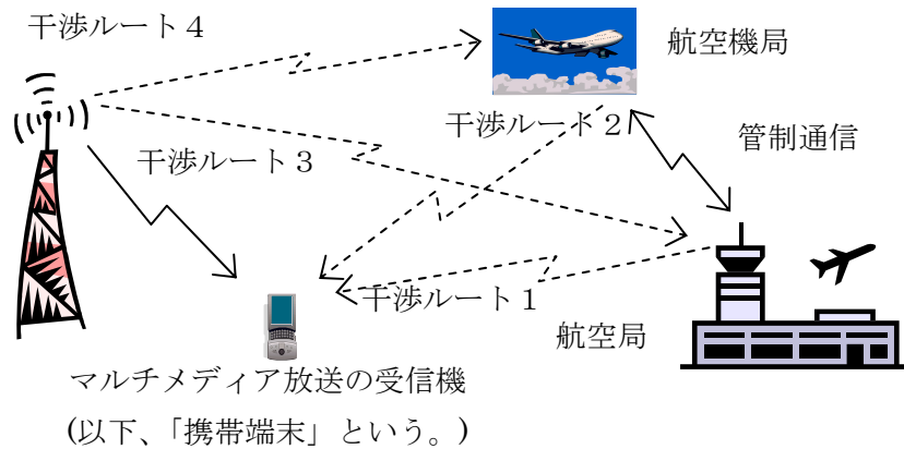
図1 航空無線システムの概要及びマルチメディア放送との干渉ルート
