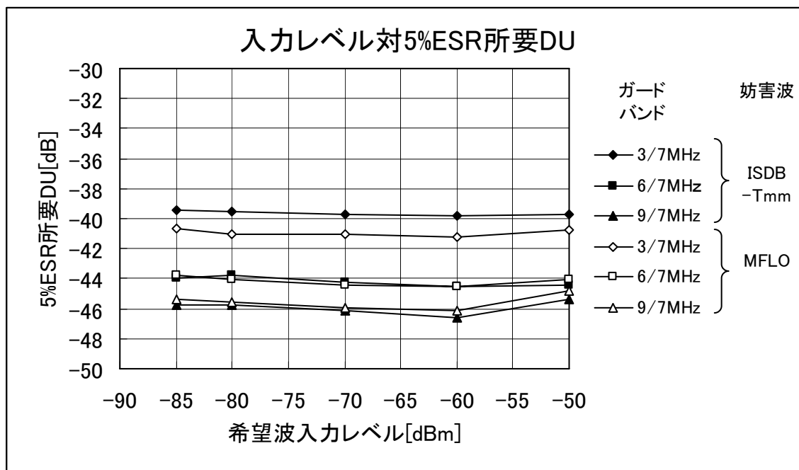
図5-10 希望波入力レベル対5%ESR所要DU (13セグメント形式))
