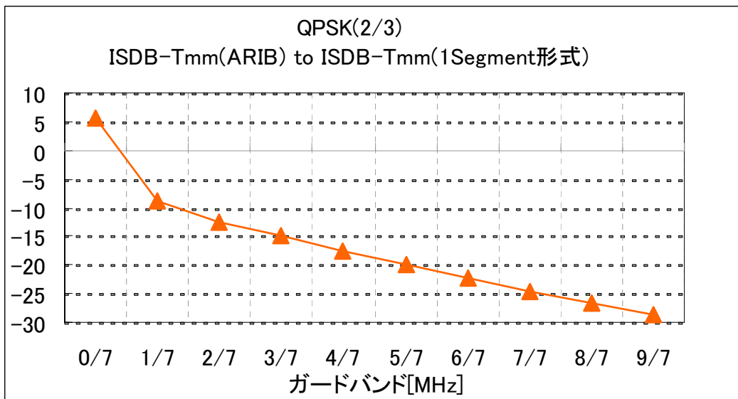
図5-4(b) ガードバンド対混信保護比 (ISDB-Tmm to ISDB-Tmm (1セグメント形式)) QPSK (2/3)
