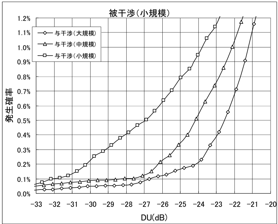
図5-14: 小規模局が被干渉局となる場合
