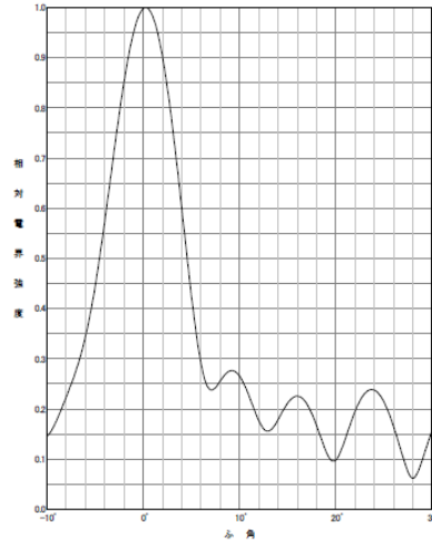
図5-11(a) 大規模局のアンテナパターン(2ダイポール8段4面)
