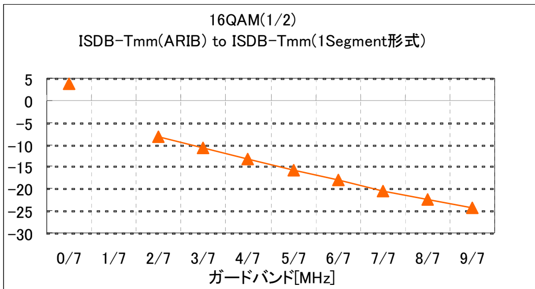
図5-4(a) ガードバンド対混信保護比 (ISDB-Tmm to ISDB-Tmm (1セグメント形式)) 16QAM (1/2)
