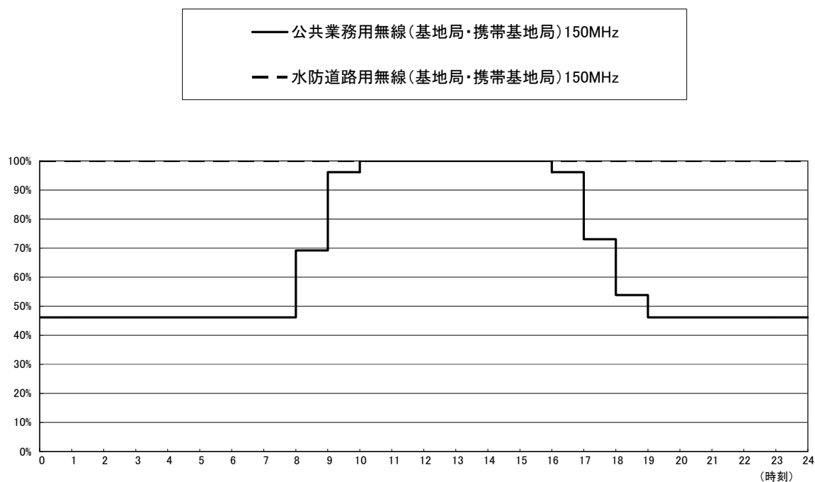
図表－6－4－9 運用時間帯の分布（公共業務用無線・水防道路用無線 150MHz）【東海】
