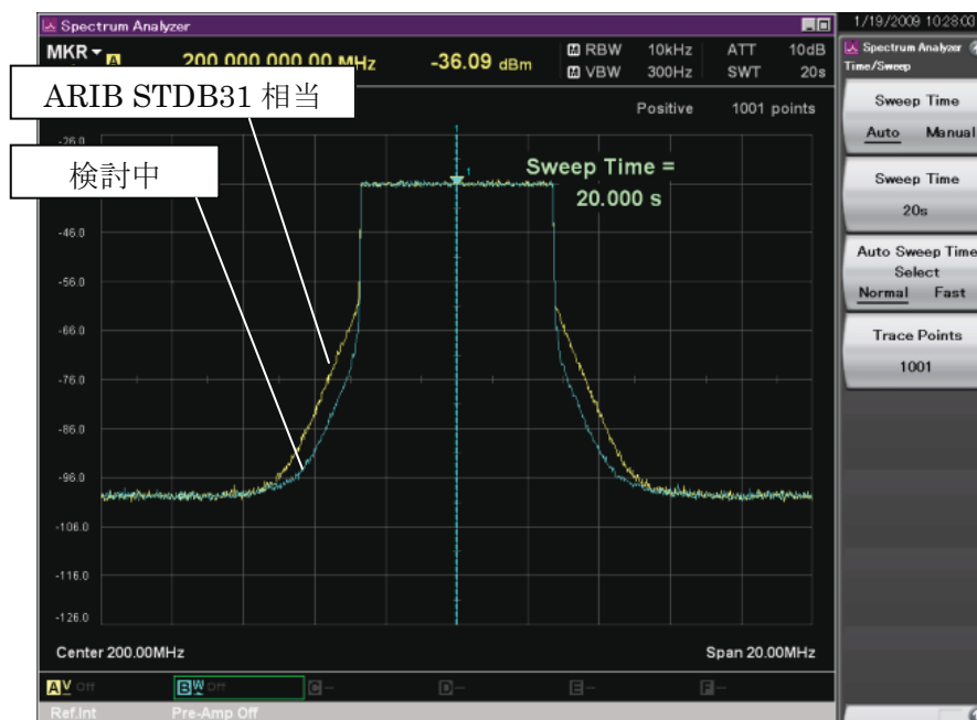
図 2-4(a) MFLO 信号
