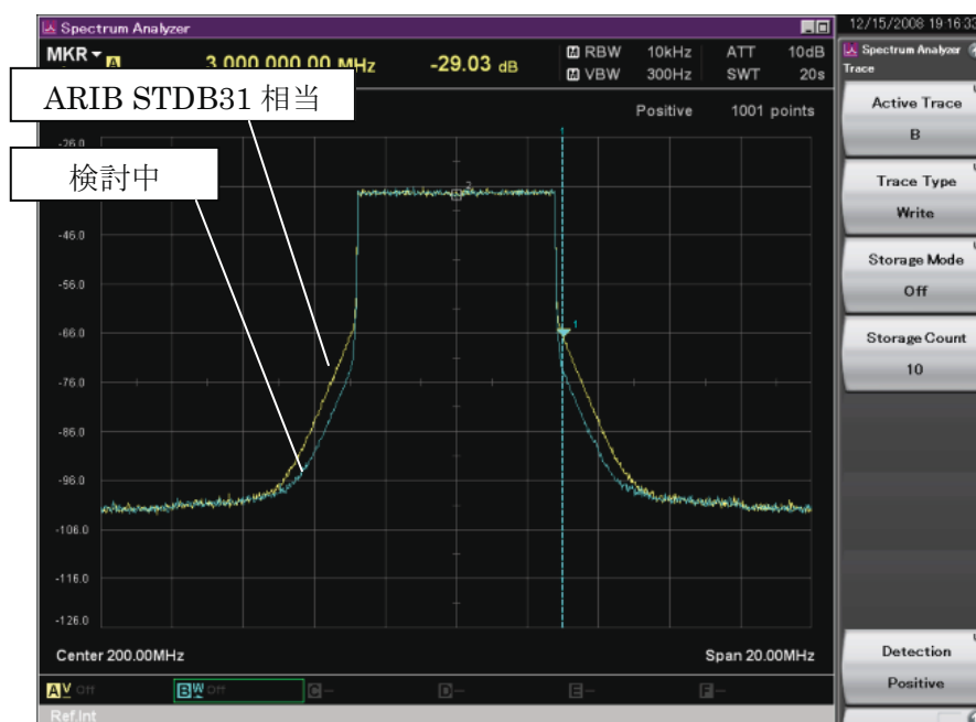
図 2-4(b) ISDB-Tmm 信号
