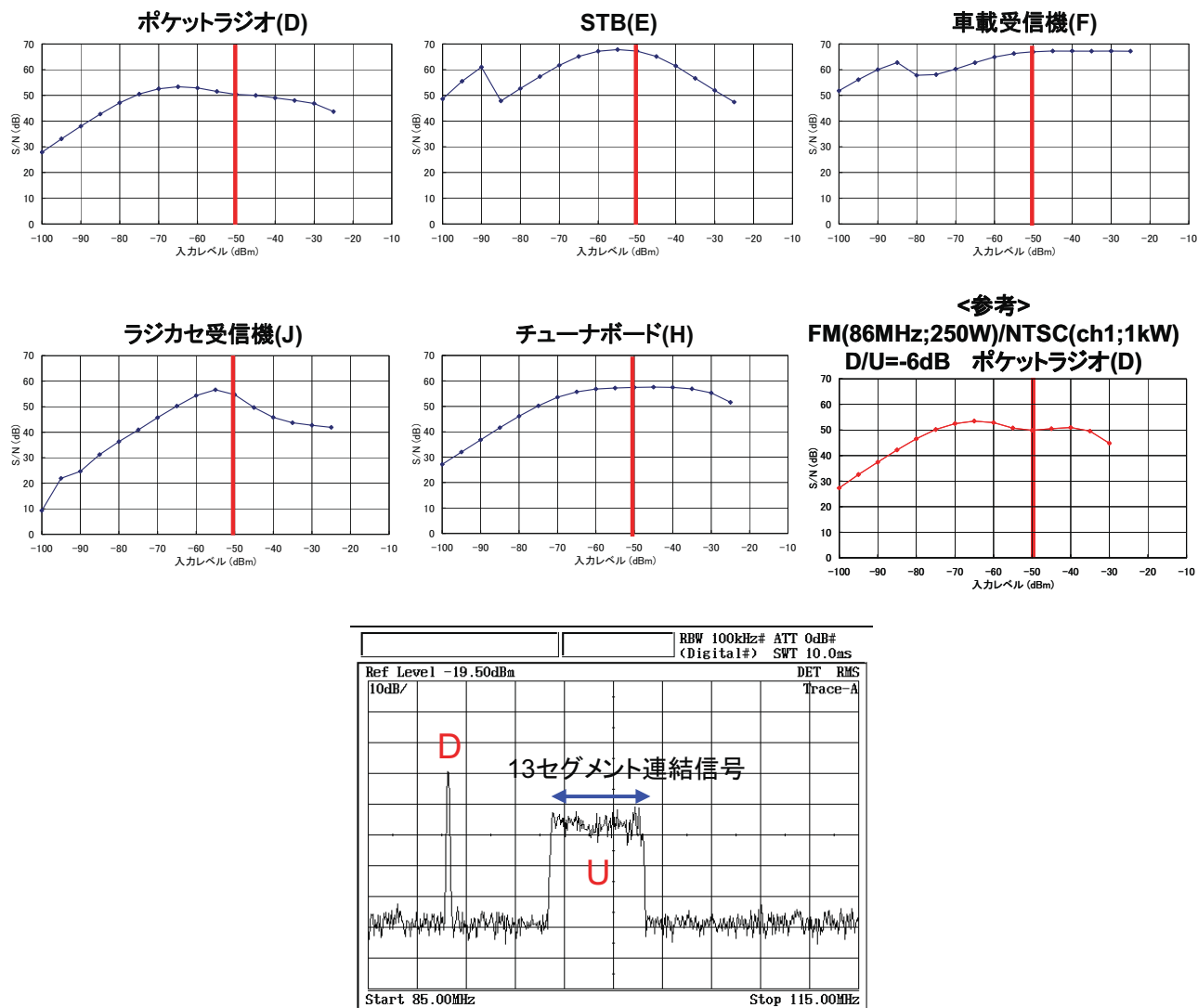
図 9 ガードバンドが 6+1/14MHz、干渉 D/U が 9dB の場合の入力レベルに対する S/N
