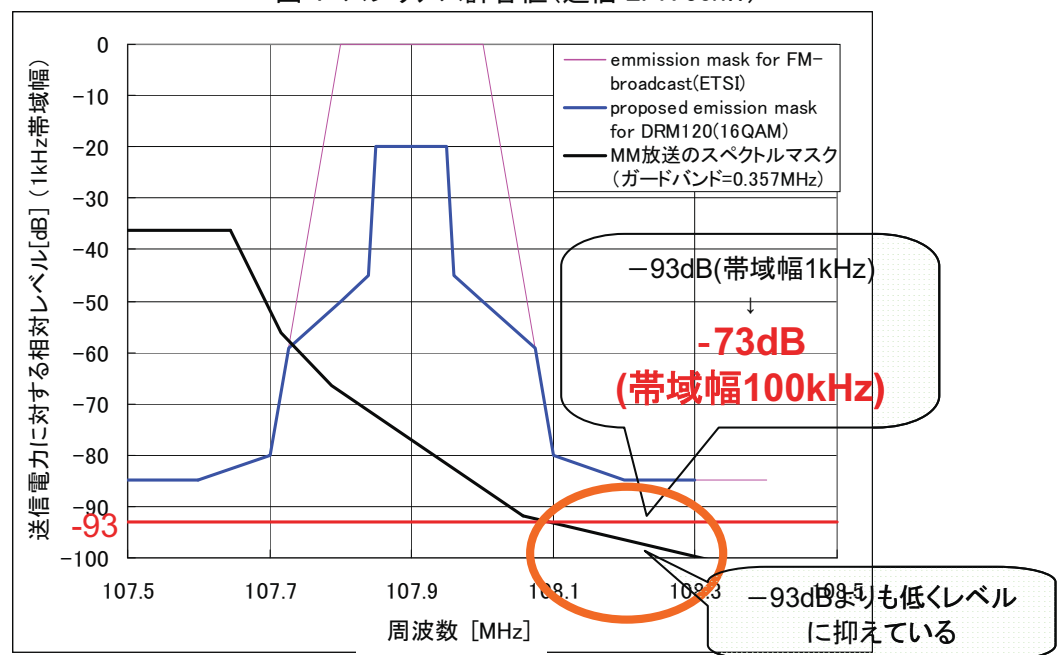
図 5 MM 放送の放射許容マスクの例(送信 ERP 50 kW)
