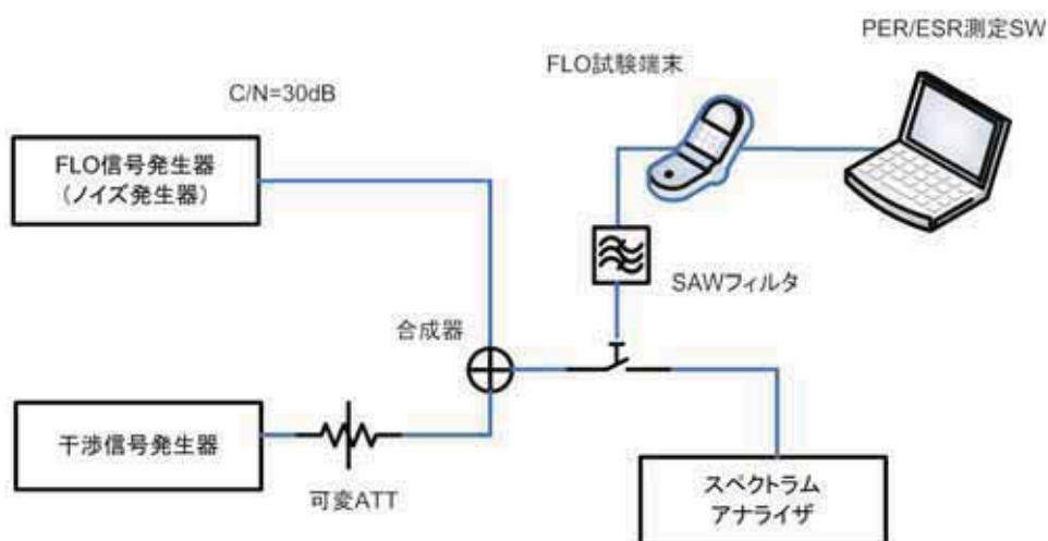
図1. 実験系統図
