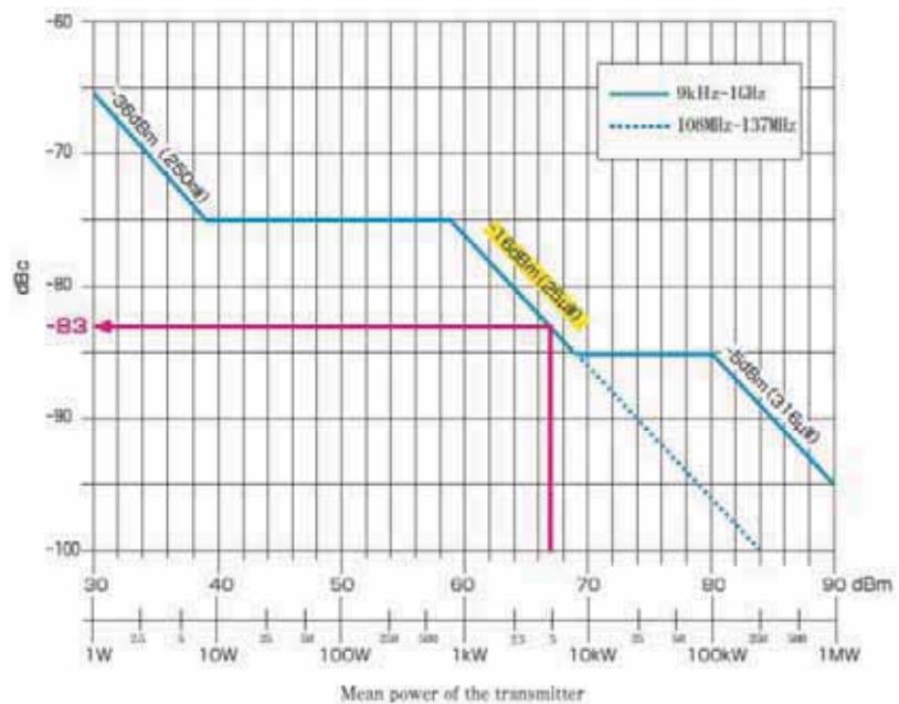
図 6 スプリアス許容値(送信 ERP5kW)
