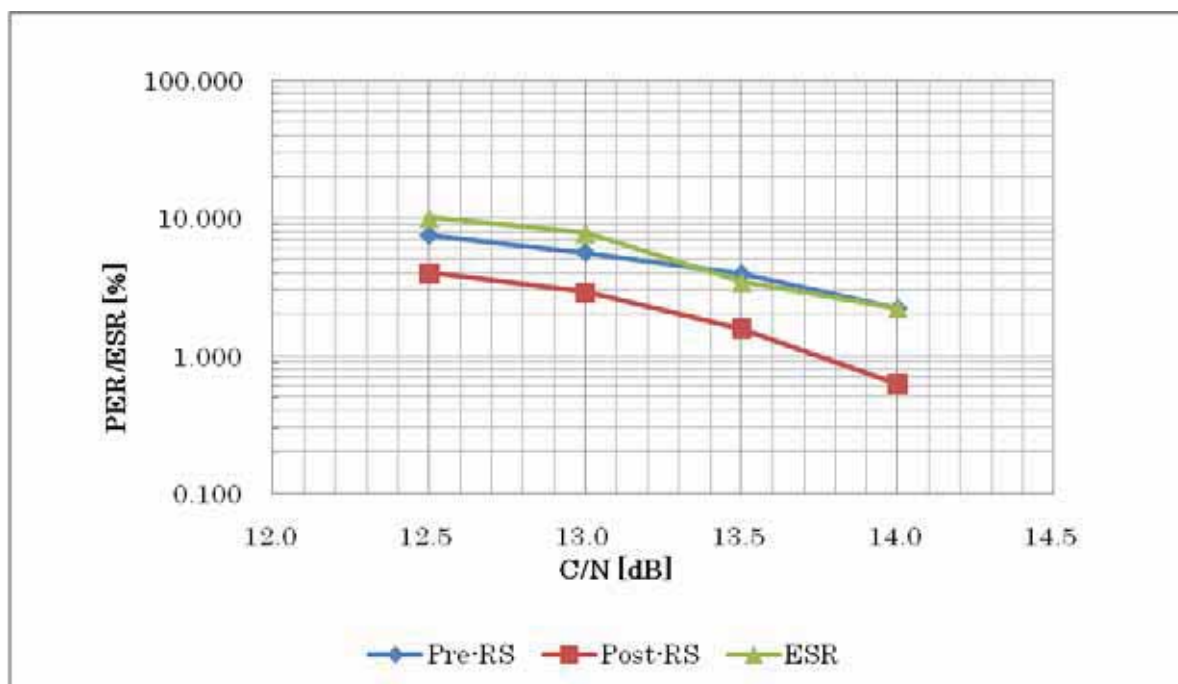
図15. フェージング環境下における所要C/N: 16QAM 1/2 RS=12/16 F_d=0.6\text{Hz}
