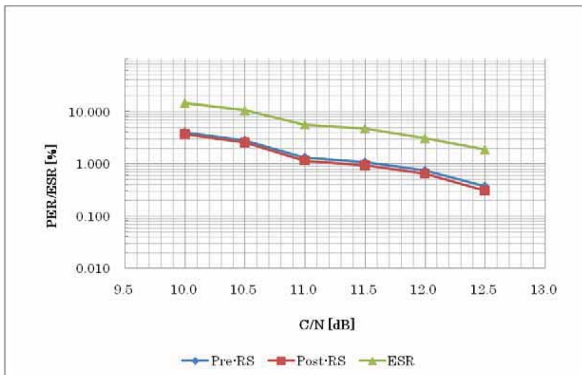
図11. フェージング環境下における所要C/N: 16QAM 1/3 RS=14/16 F_d=0.6\text{Hz}
