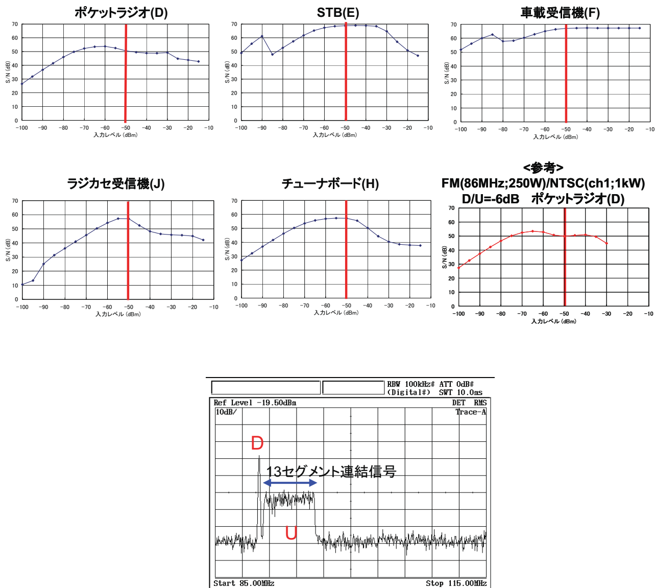
図 7 ガードバンドが 5/14MHz、干渉 D/U が 17dB の場合の入力レベルに対する S/N
