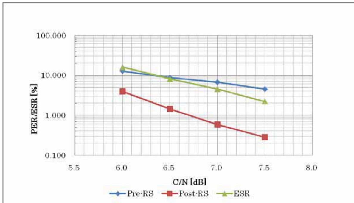
図9. フェージング環境下における所要C/N: QPSK 1/2 RS=12/16 F_d=20\text{Hz}
