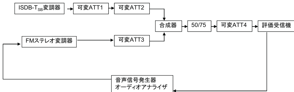
図 1 実験系統図
