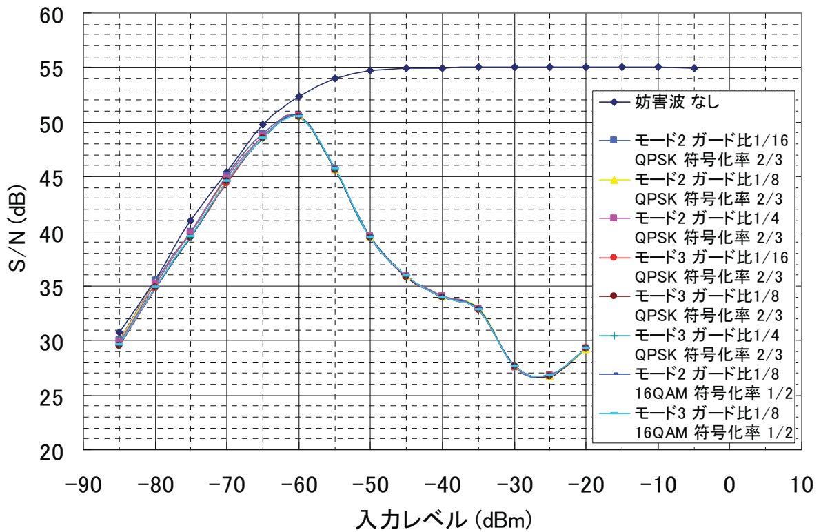
図2 伝送パラメータによる比較
