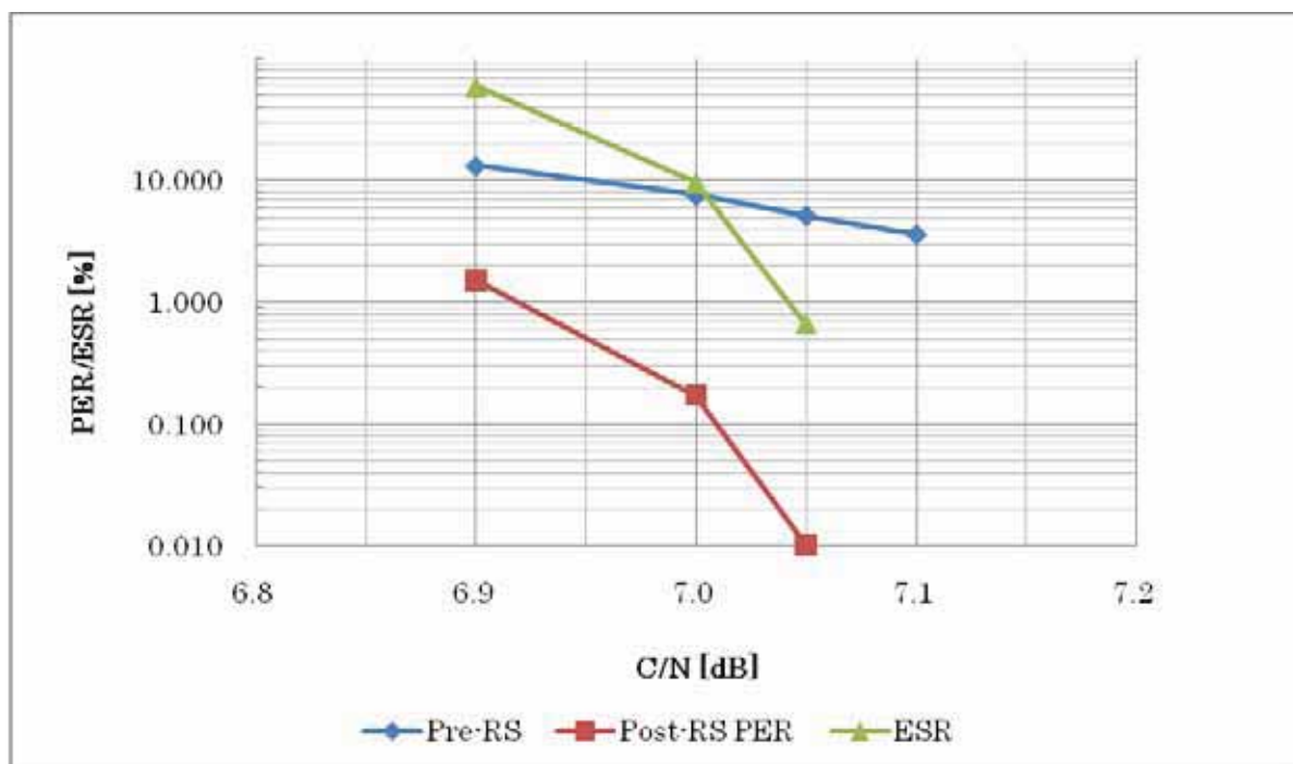
図6. AWGN環境下における所要C/N: 16QAM 1/2 RS=12/16
