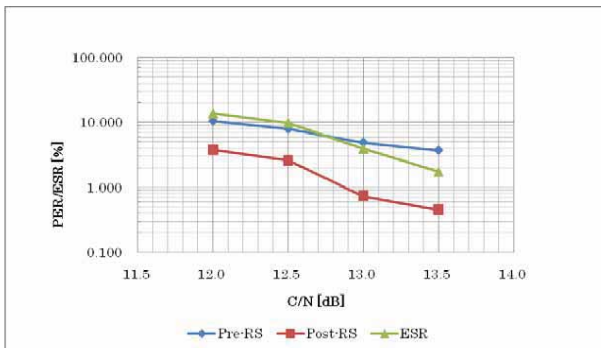
図16. フェージング環境下における所要C/N: 16QAM 1/2 RS=12/16 F_d=10\text{Hz}
