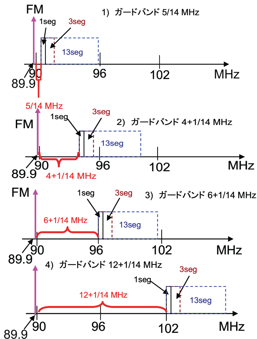
図 3 周波数配置
