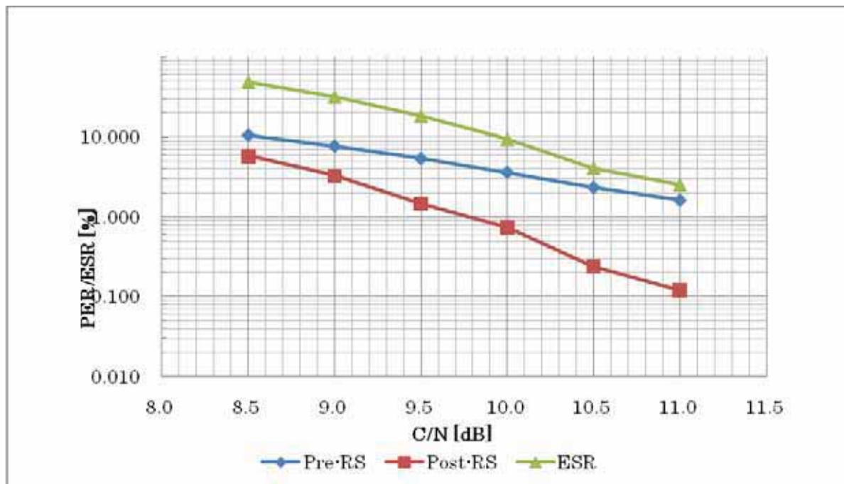
図13. フェージング環境下における所要C/N: 16QAM 1/3 RS=14/16 F_d=20\text{Hz}
