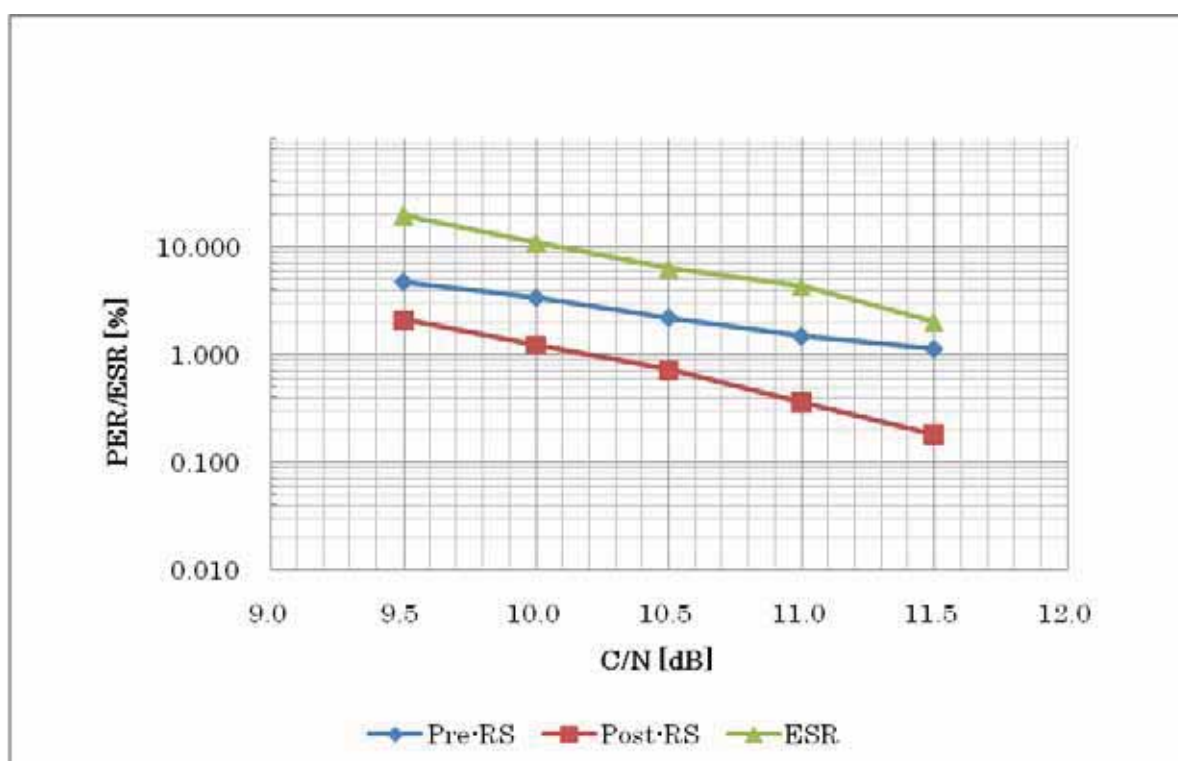
図12. フェージング環境下における所要C/N: 16QAM 1/3 RS=14/16 F_d=10\text{Hz}
