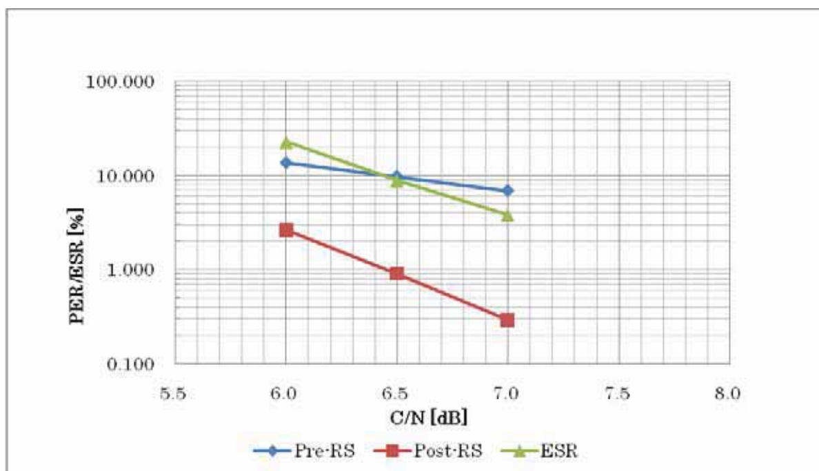
図10. フェージング環境下における所要C/N: QPSK 1/2 RS=12/16 F_d=40\text{Hz}
