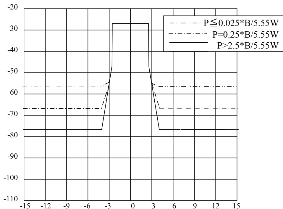
図 1-2 MediaFLO方式マルチメディア放送の送信スペクトルマスク ( B=4.625 、 6.475 もしくは 7.4\text{MHz} )
