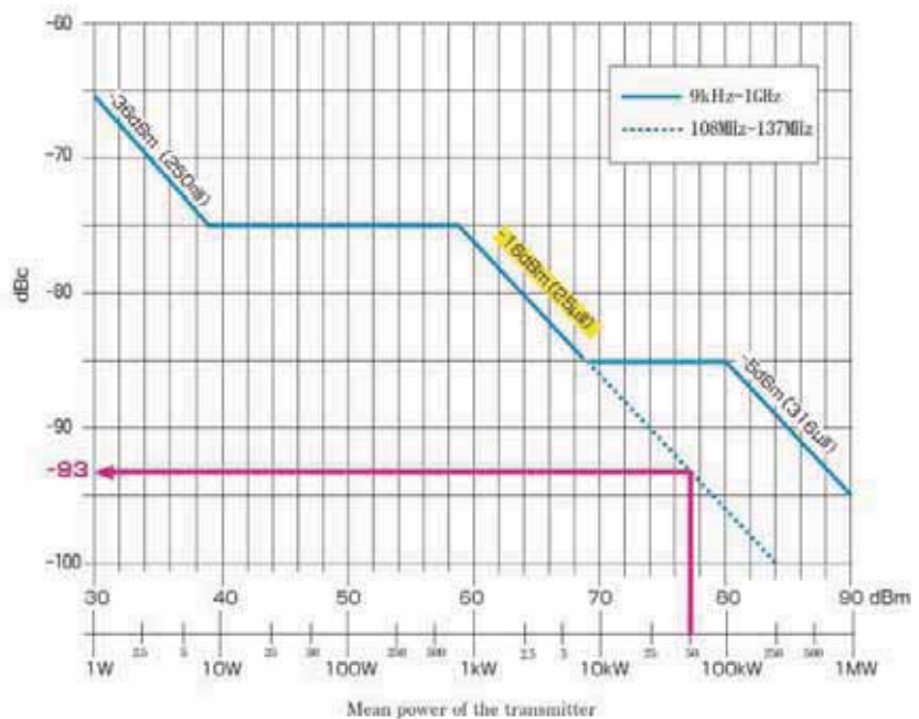
図 4 スプリアス許容値(送信 EPR 50kW)
