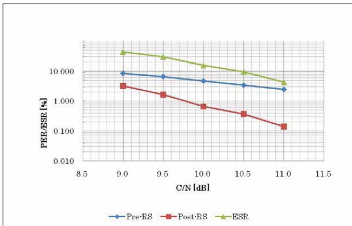
図14. フェージング環境下における所要C/N: 16QAM 1/3 RS=14/16 F_d=40\text{Hz}
