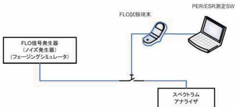
図1. 実験系統図
