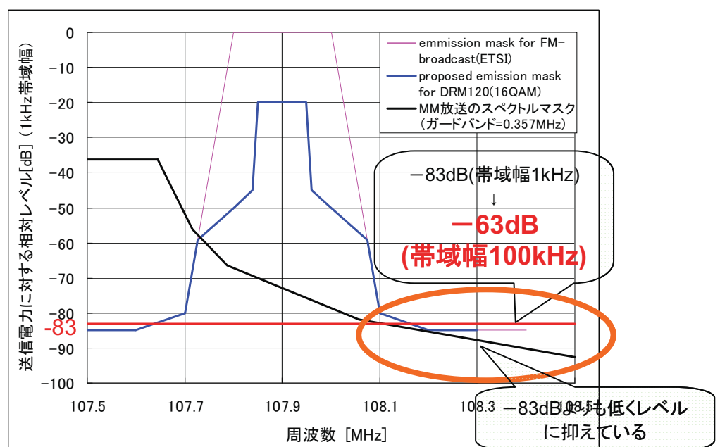
図 7 MM 放送の放射許容マスクの例 (送信 ERP 5kW)
