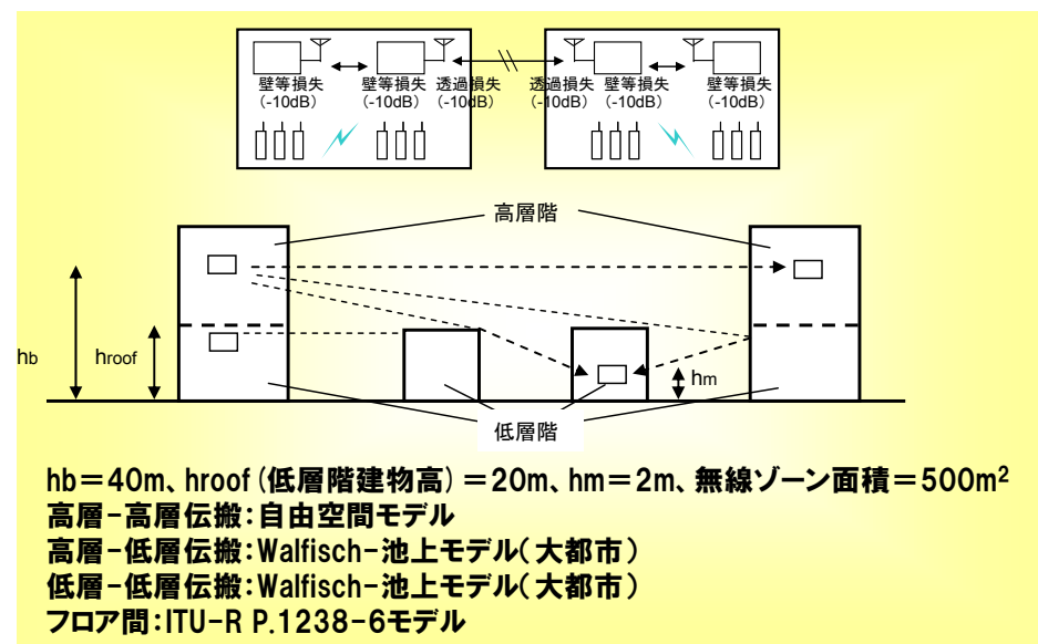
(2) オフィス街の干渉モデル
