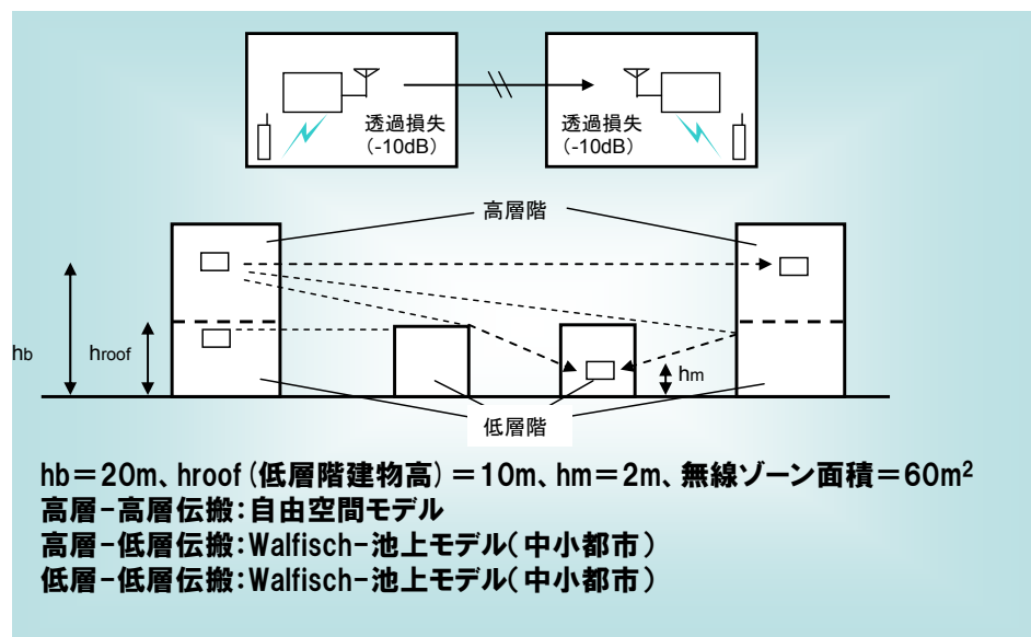
(1) マンション群の干渉モデル
